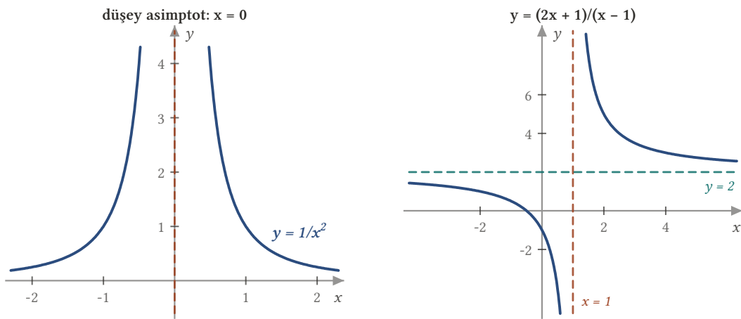
Şekil 32.3: Solda y = 1/x^2 : x \rightarrow 0 iken değerler sınırsız büyür, grafik x = 0 doğrusuna yaslanır (düşey asimptot); x \rightarrow \pm\infty iken de 0'a yaklaşır. Sağda y = (2x + 1)/(x - 1) : x = 1 'de düşey asimptot vardır; x \rightarrow \pm\infty iken limit 2 olduğundan y = 2 doğrusu yatay asimptottur.
