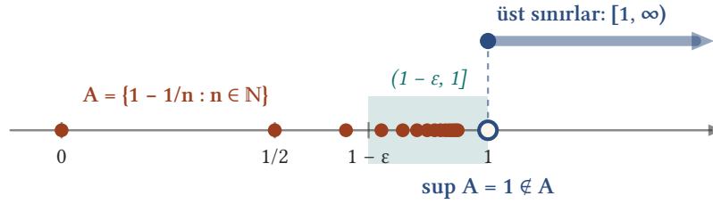
Şekil 10.1: A = \{1 - 1/n\} kümesinin elemanları 1'e soldan yığılır; 1 kümeye ait olmayan (içi boş) en küçük üst sınırdır. 1'in sağındaki her sayı üst sınırdır ve 1'in hemen solundaki her (1 - \varepsilon, 1] penceresi kümeden en az bir eleman içerir.
