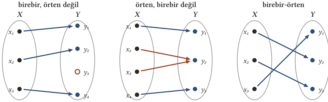
Şekil 5.2: Solda farklı x 'ler farklı y 'lere gider ama y_3 'e hiç ok gelmez (birebir, örten değil). Ortada her y 'ye ok gelir ama y_2 'ye iki ok gelir (örten, birebir değil). Sağda her y 'ye tam bir ok gelir: birebir-örten.
