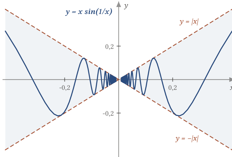
Şekil 30.1: y = x \sin(1/x) grafiği, kesikli çizilen y = |x| ve y = -|x| zarfları arasında kalır: -|x| \leq x \sin(1/x) \leq |x| . Salınımlar 0 'a yaklaşırken sıklaşır, ama iki zarf 0 'da birleştiğinden fonksiyon aralarında sıkışıp 0 'a gider.
