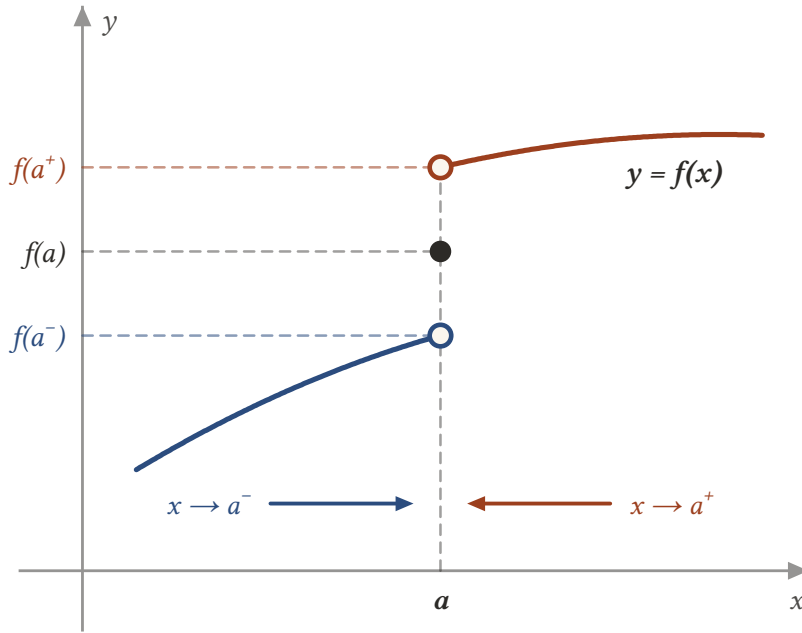
Şekil 31.1: a noktasında sıçrayan bir fonksiyon. Soldan yaklaşıncsa değerler f(a^-) 'ye, sağdan yaklaşıncsa f(a^+) 'ya yığılır; iki tek yönlü limit de vardır ama farklıdır, bu yüzden x \rightarrow a limiti yoktur. Fonksiyonun a 'daki değeri f(a) ise ikisinden de bağımsızdır: tek yönlü limitler yalnızca a 'nın yanındaki noktalara bakar.
