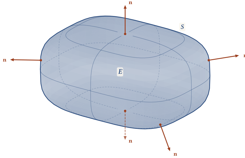
Şekil 18.1: Basit katı bölge E ve onu çevreleyen kapalı S yüzeyi. Pozitif yönde birim normal \mathbf{n} her noktada E 'nin dışına bakar (kesikli ok, görünmeyen alt yüzdeki normaldir). Diverjans Teoremi, \mathbf{F} 'nin S 'den dışarı akısını \operatorname{div} \mathbf{F} 'nin E üzerindeki integraline eşitler.
