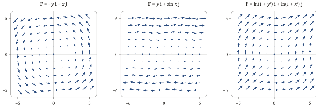
Şekil 10.3: Bilgisayarla çizilmiş üç vektör alanı. Oklar aynı oranda kısaltıldı; birbirine çarpmazlar ama uzunlukları gerçek uzunluklarıyla orantılıdır. Soldaki alan dönme alanıdır.
