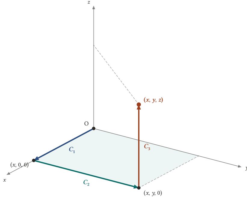
Şekil 14.1: Potansiyel, orijinden (O) (x, y, z) noktasına eksenlere paralel üç doğru parçası boyunca toplanır: C_1 üzerinde yalnız x , C_2 üzerinde yalnız y , C_3 üzerinde yalnız z değişir; bu yüzden sırasıyla yalnız P , Q ve R katkı verir.
