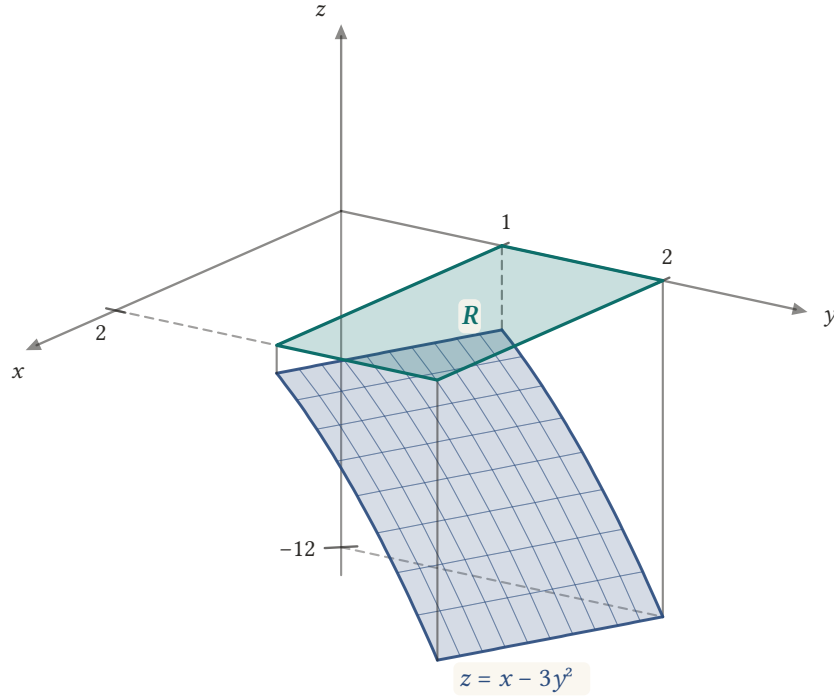
Şekil 1.6: R = [0, 2] \times [1, 2] üzerinde z = x - 3y^2 yüzeyi xy -düzleminin tümüyle altındadır (düşey eksen küçültülmüş ölçekte). R ile yüzey arasındaki cismin hacmi 12'dir; integral bunun ters işaretlisi olan -12 'dir.
