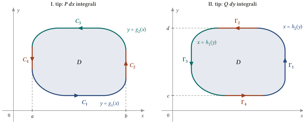
Şekil 13.2: Aynı basit bölge iki biçimde. Solda I. tip betim: alt eğri C_1 ( y = g_1(x) ), üst eğri C_3 ( y = g_2(x) ) ve üzerlerinde dx = 0 olan düşey parçalar C_2, C_4 . Sağda II. tip betim: sağ eğri \Gamma_1 ( x = h_2(y) ), sol eğri \Gamma_3 ( x = h_1(y) ) ve üzerlerinde dy = 0 olan yatay parçalar \Gamma_2, \Gamma_4 .
