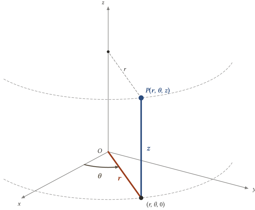
Şekil 7.1: P noktasının silindirik koordinatları: (r, \theta) , P 'nin xy -düzlemindeki izdüşümünün kutupsal koordinatları, z ise P 'nin yüksekliğidir. r aynı zamanda P 'nin z eksenine uzaklığıdır; kesikli yaylar P 'den geçen r = \text{sabit} silindirin izleridir.
