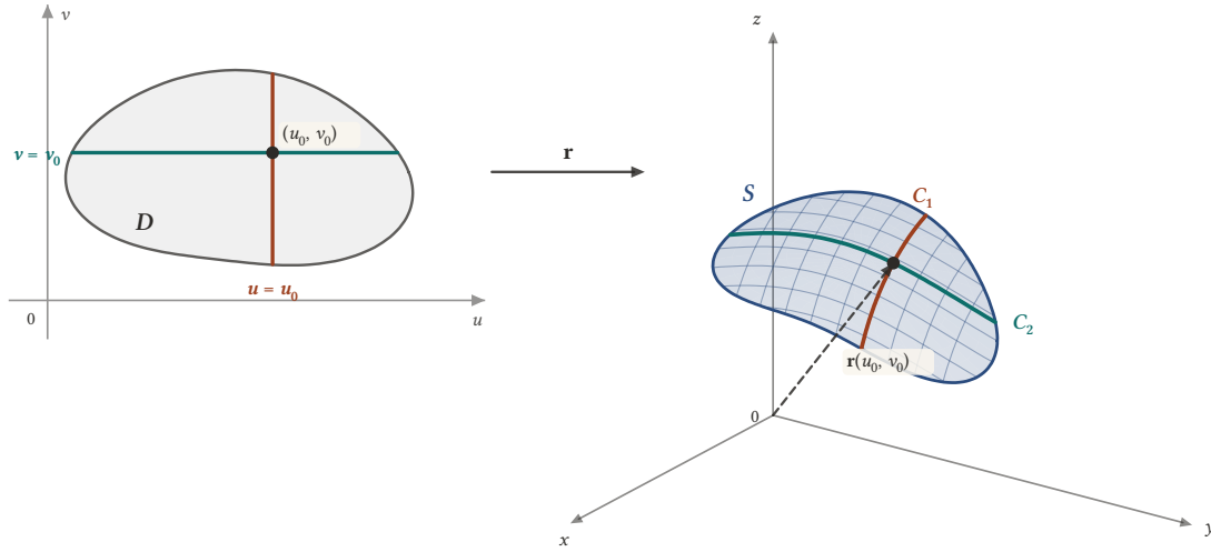
Şekil 15.1: \mathbf{r} , uv -düzlemindeki D bölgesini uzaydaki S yüzeyine gönderir: (u_0, v_0) noktası, konum vektörü \mathbf{r}(u_0, v_0) olan noktaya gider. D 'deki u = u_0 düşey doğrusunun görüntüsü C_1 , v = v_0 yatay doğrusunun görüntüsü C_2 koordinat eğrisidir.
