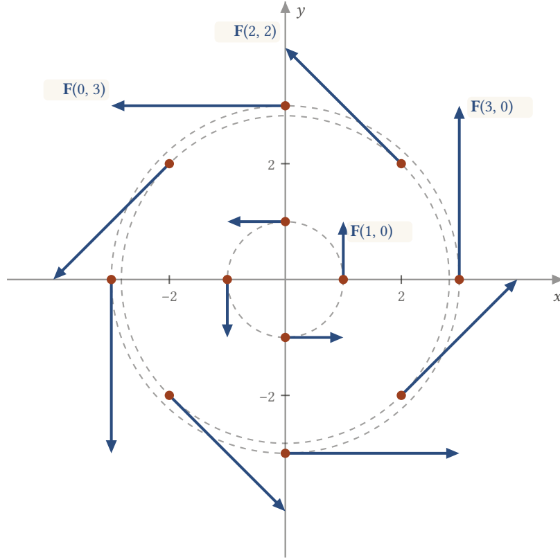
Şekil 10.2: Tablodaki on iki vektör, başlangıçları kendi noktalarında olacak biçimde çizildi. Her ok, orijin merkezli bir çembere (kesikli) teğettir ve uzunluğu o çemberin yarıçapına eşittir; oklar saat yönünün tersine döner.
