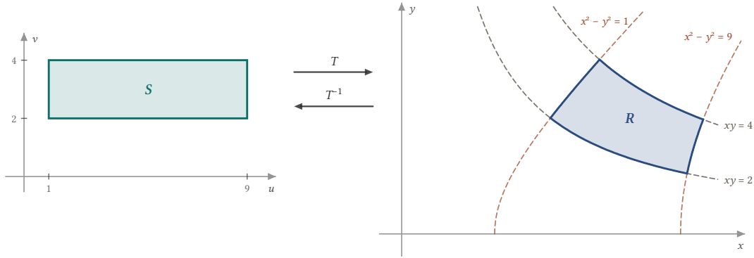
Şekil 9.7: u = x^2 - y^2 , v = xy değişkenleri birinci bölgedeki dört hiperbolün sınırladığı R bölgesini [1, 9] \times [2, 4] diktörtgenine çevirir.
