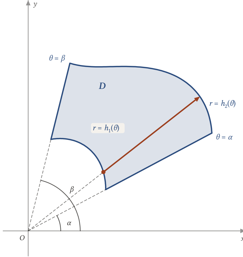
Şekil 3.4: D = \{(r, \theta) \mid \alpha \leq \theta \leq \beta, h_1(\theta) \leq r \leq h_2(\theta)\} . Orijinden çıkan her ışın D'ye r = h_1(\theta) eğrisinde girer, r = h_2(\theta) eğrisinde çıkar; iç integralin sınırları bunlardır.
