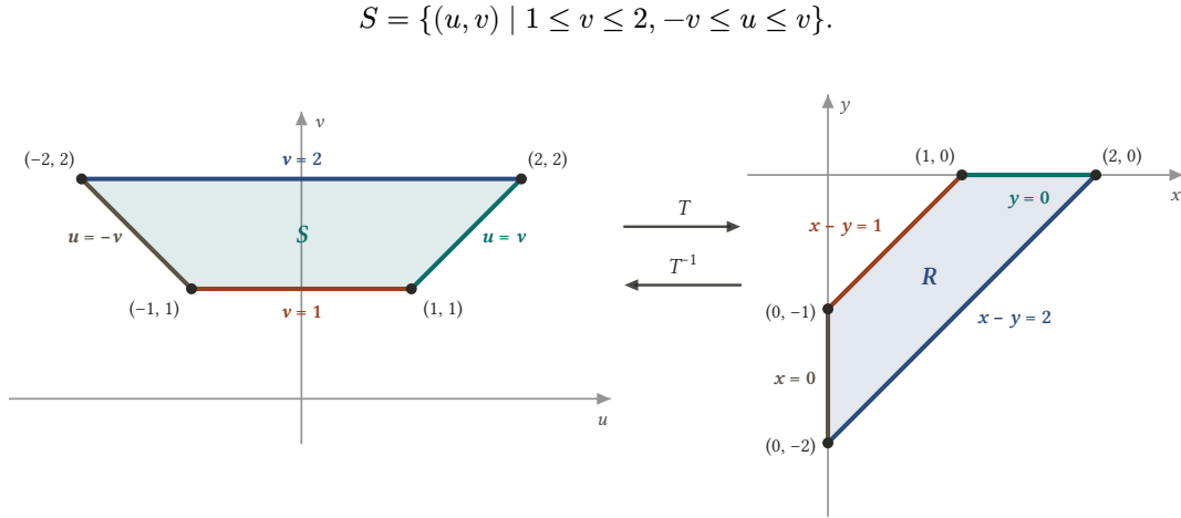
Şekil 9.6: u = x + y , v = x - y ile R yamuğunun her kenarı S yamuğunun aynı renkteki kenarına gider. T ise x = (u + v)/2 , y = (u - v)/2 ile S 'yi R 'ye geri götürür.
