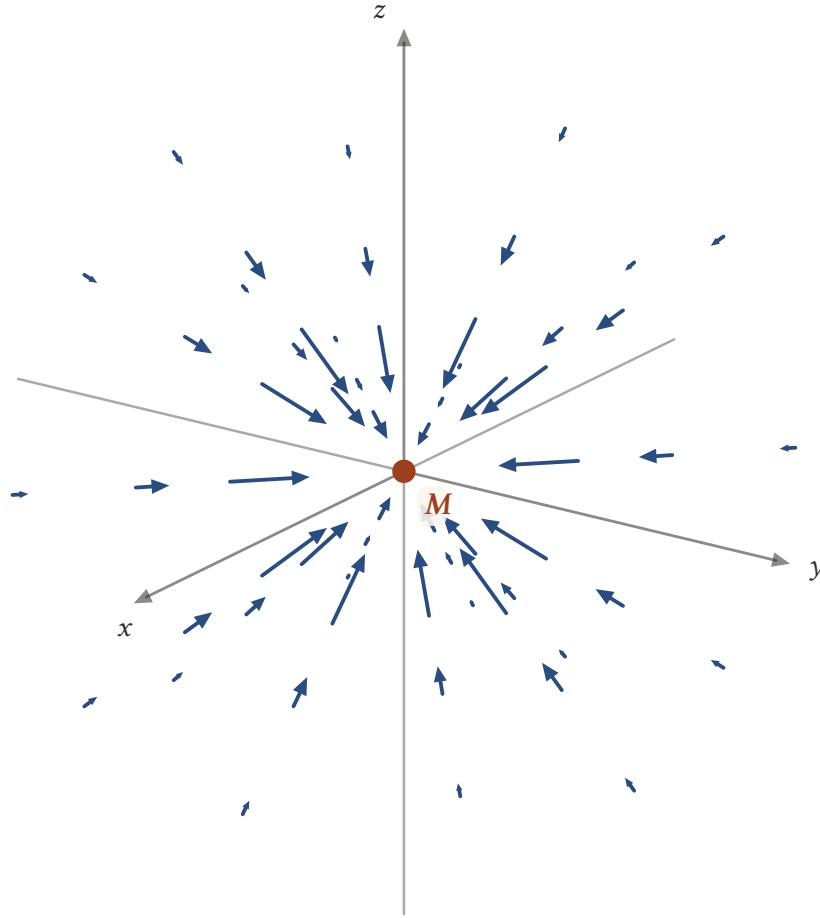
Şekil 10.6: Orijindeki M kütesinin kütle çekim alanı. Oklar orijine yönelir; büyüklükleri uzaklığın karesiyle ters orantılı olduğundan orijine yaklaştıkça hızla uzar. Oklar orijin merkezli üç küre üzerindeki noktalardan çizildi.
