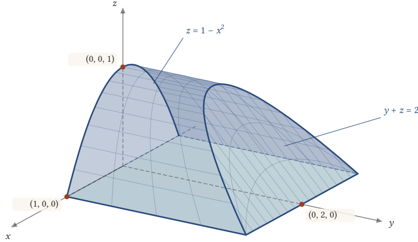
Şekil 18.3: E cismi: üstten z = 1 - x^2 parabolik silindiri, alttan z = 0 , arkadan y = 0 ve sağdan y + z = 2 düzlemiyle sınırlıdır. Yüzeyi dört parçadan oluşur.
