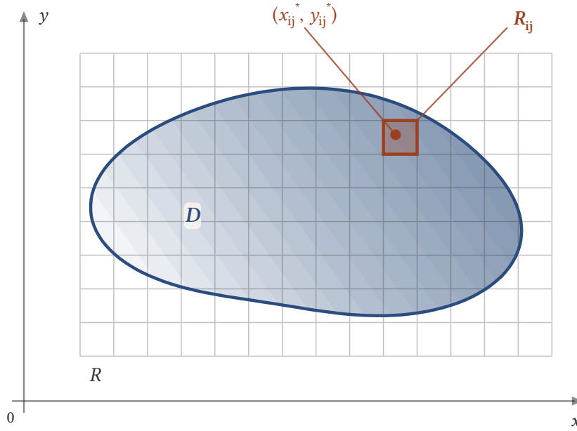
Şekil 4.1: D bölgesini içeren R dikdörtgeni eşit alt dikdörtgenlere bölünür ve D dışında \rho = 0 alınır; renk koyulaştıkça yoğunluk büyür. Turuncu R_{ij} parçasının kütlesi yaklaşık \rho(x_{ij}^*, y_{ij}^*) \Delta A 'dır.
