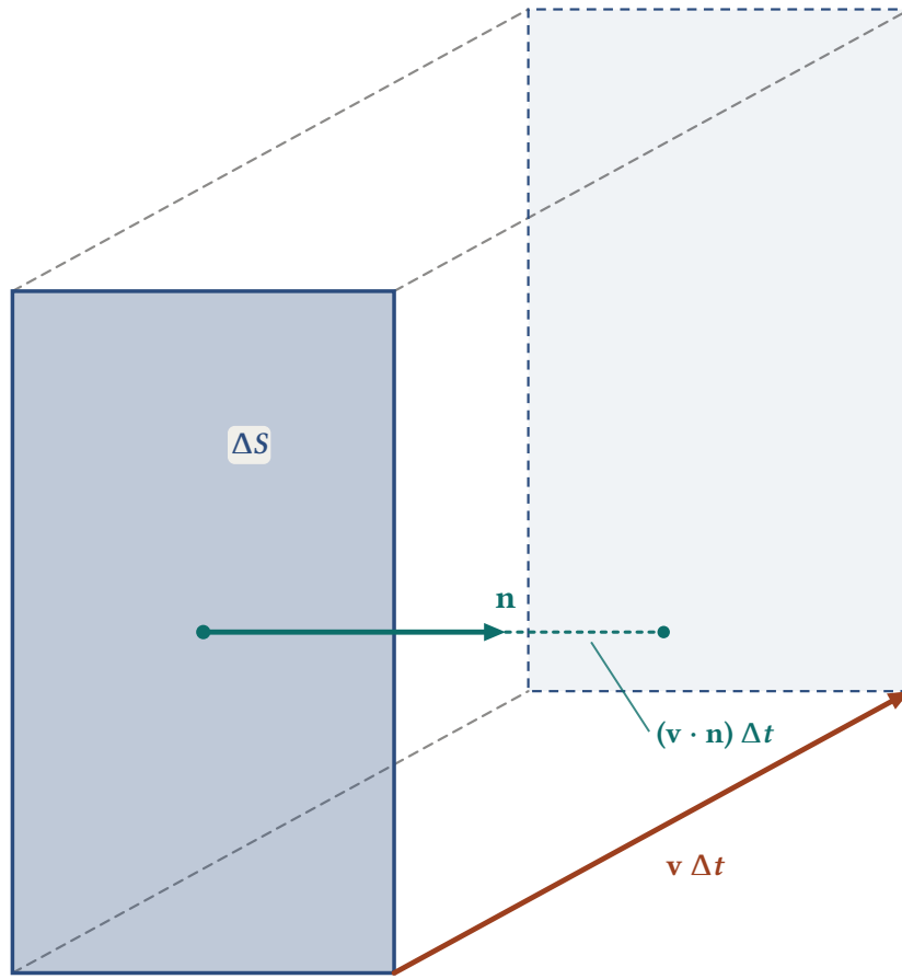
Şekil 16.6: Alanı \Delta S olan küçük, düz bir yamadan \Delta t sürede geçen akışkan, tabanı bu yama ve yan kenarları \mathbf{v} \Delta t olan eğik bir prizmayı doldurur. Prizmanın yüksekliği \mathbf{v} \Delta t 'nin \mathbf{n} doğrultusundaki bileşeni (\mathbf{v} \cdot \mathbf{n}) \Delta t , hacmi (\mathbf{v} \cdot \mathbf{n}) \Delta S \Delta t 'dir.
