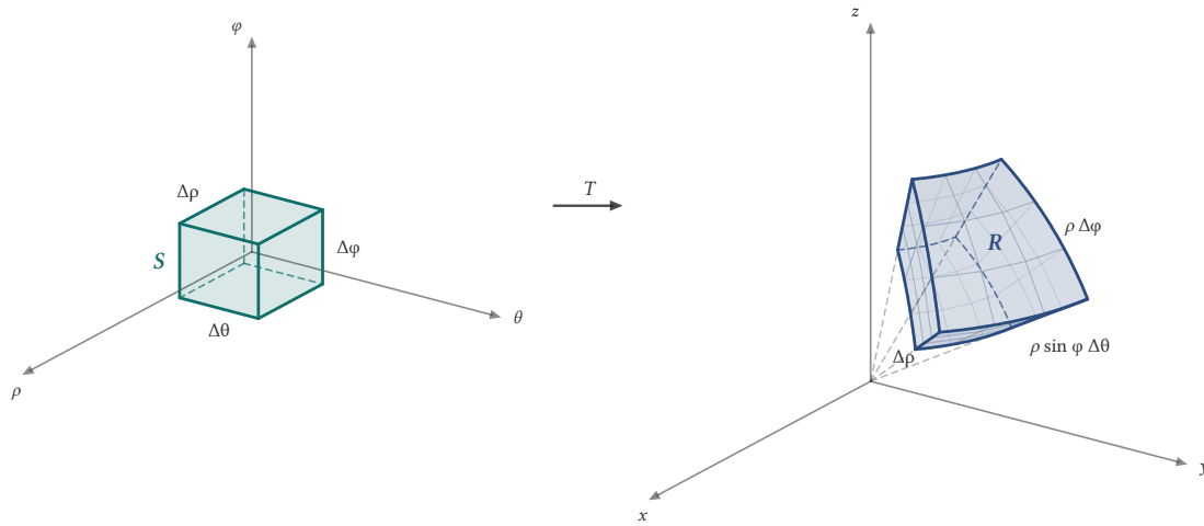
Şekil 9.8: Küresel koordinat dönüşümü (\rho, \theta, \varphi) -uzayındaki küçük S kutusunu bir küresel kama R 'ye götürür. Kamanın kenarları yaklaşık \Delta\rho , \rho \sin \varphi \Delta\theta ve \rho \Delta\varphi olduğundan hacmi yaklaşık \rho^2 \sin \varphi \Delta\rho \Delta\theta \Delta\varphi 'dir; bu çarpan Jacobi determinantının mutlak değeridir.
