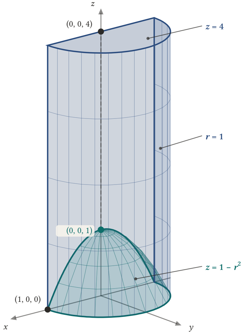
Şekil 7.6: x^2 + y^2 = 1 silindirisinin içinde, y \geq 0 tarafında, z = 1 - x^2 - y^2 paraboloidinin üstünde ve z = 4 düzleminin altında kalan cisim. Silindirik koordinatlarda 0 \leq \theta \leq \pi , 0 \leq r \leq 1 , 1 - r^2 \leq z \leq 4 'tür.
