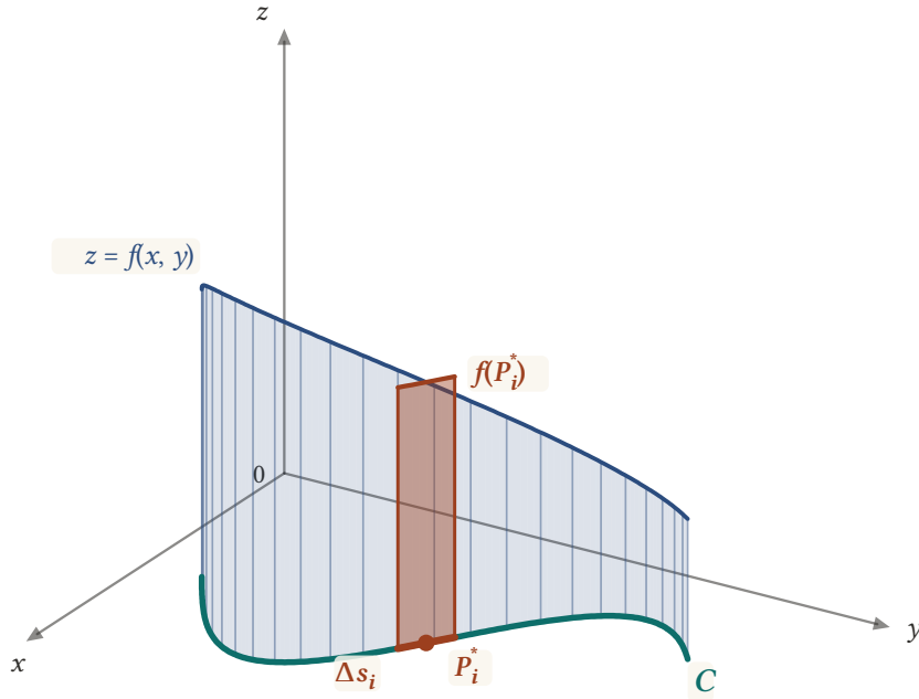
Şekil 11.2: f \geq 0 iken \int_C f ds , tabanı xy -düzlemindeki C eğrisi ve (x, y) noktasındaki yüksekliği f(x, y) olan perdenin bir yüzünün alanıdır. Turuncu şeridin alanı f(P_i^*) \Delta s_i çarpımıdır; bu şeritlerin toplamı Riemann toplamını verir.
