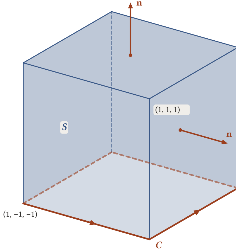
Şekil 17.8: Köşeleri (\pm 1, \pm 1, \pm 1) olan küpün tabanı çıkarılmış yüzeyi S : üst yüz ve dört yan yüz, normaller dışa doğru. Sınırı, z = -1 düzlemindeki kare C dir ve yukarıdan bakınca saat yönünün tersine dolanır.
