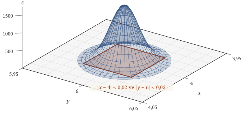
Şekil 4.7: Ortak yoğunluk f(x, y) = (5000/\pi) e^{-5000[(x-4)^2 + (y-6)^2]} , (4, 6) noktası üzerinde dik bir tepedir; en büyük değeri 5000/\pi \approx 1592 'dir. Tabandaki turuncu kare |x - 4| < 0,02 , |y - 6| < 0,02 bölgesidir; bu karenin üstünde ve grafiğin altında kalan hacim yaklaşık 0,91'dir.
