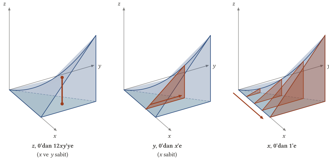
Şekil 6.4: z \rightarrow y \rightarrow x sırasındaki ardışık integral E 'yi üç adımda tarar. Önce sabit (x, y) için z 0'dan 12xy 'ye giden bir dikey çubuk, sonra sabit x için bu çubukların süpürdüğü üçgen dilim, en sonda x 0'dan 1'e giderken dilimlerin doldurduğu cisim.
