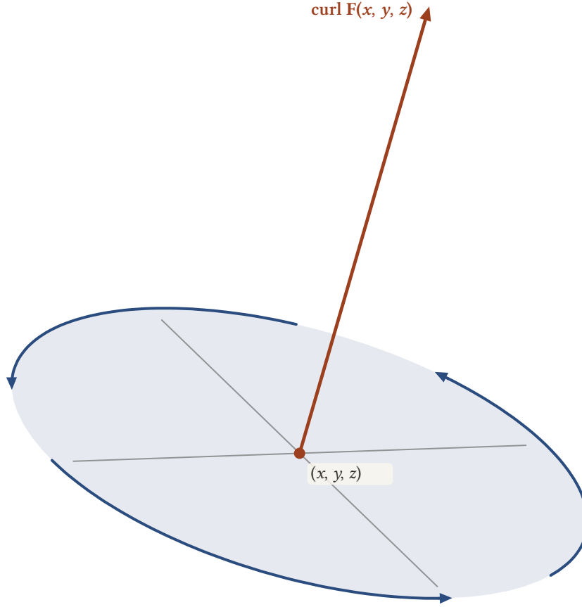
Şekil 14.2: Hız alanı \mathbf{F} olan bir akışkanda (x, y, z) noktasının yakınındaki parçacıklar, \text{curl } \mathbf{F}(x, y, z) doğrultusundaki eksen etrafında döner. Vektörün ucundan bakıldığında dönme saatin tersi yönündedir (sağ el kuralı); vektörün uzunluğu dönmenin hızını ölçer.
