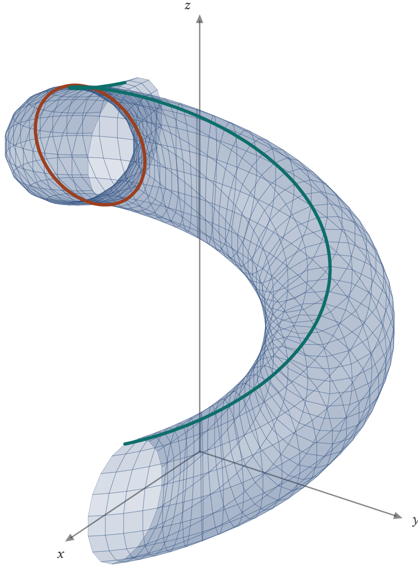
Şekil 15.3: Yüzeyin 0 \leq u \leq 2\pi , 0 \leq v \leq 2\pi parçası bir tam tur atan bir tüptür. Kalın çizilen iki koordinat eğrisinden biri küçük bir çember, öbürü bir sarmaldır.
