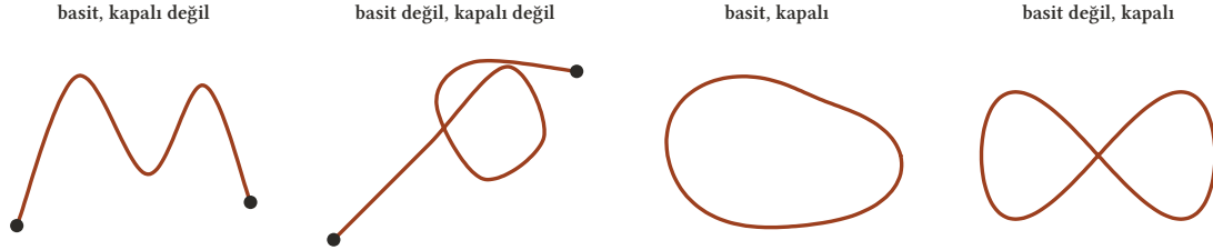
Şekil 12.5: Eğri türleri. Kapalı olmayan eğrilerde uç noktalar işaretlidir. İkinci eğri kendisini bir kez keser; dördüncü eğri (8 biçimi) başladığı yere döner ama ortadaki noktadan iki kez geçer.
