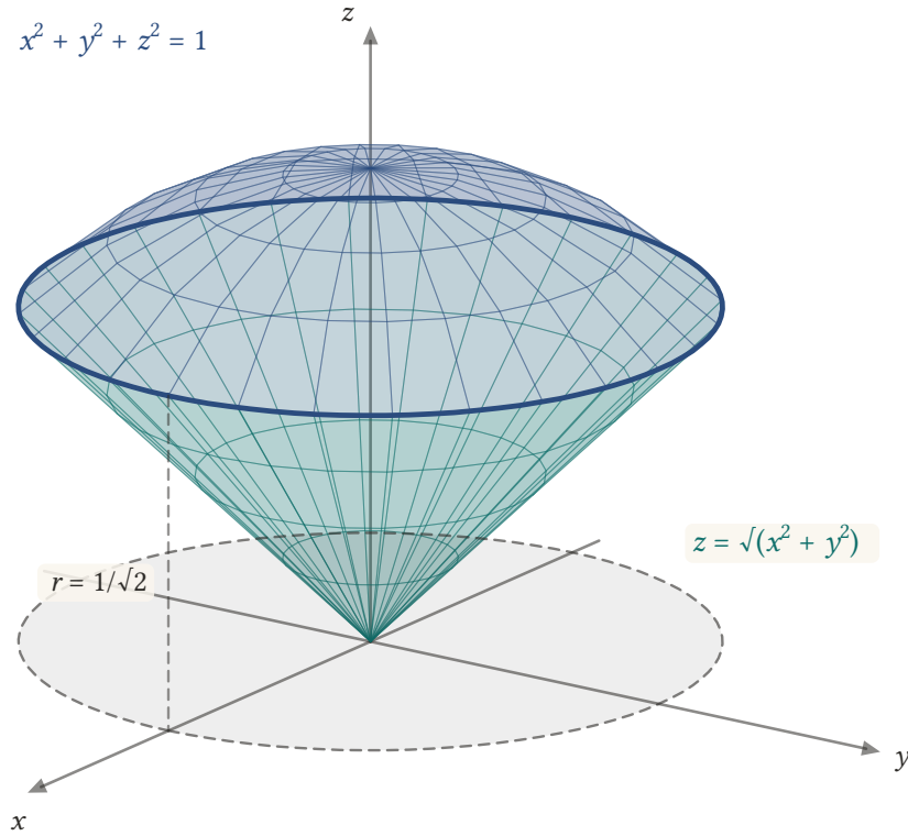
Şekil 3.8: z = \sqrt{x^2 + y^2} konisinin üstünde ve birim kürenin altında kalan dondurma külahı biçimli cisim. Koni ile küre z = 1/\sqrt{2} yüksekliğinde, r = 1/\sqrt{2} yarıçaplı çember boyunca kesişir; cismin xy -düzlemindeki izdüşümü bu yarıçaplı disklerdir.
