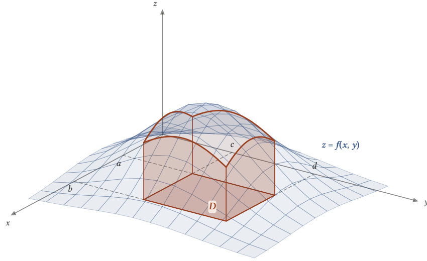
Şekil 4.6: P(a \leq X \leq b, c \leq Y \leq d) olasılığı, D = [a, b] \times [c, d] dikdörtgeninin üstünde ve ortak yoğunluk fonksiyonunun grafiğinin altında kalan cismin hacmidir. Bütün grafiğin altındaki hacim 1'dir.
