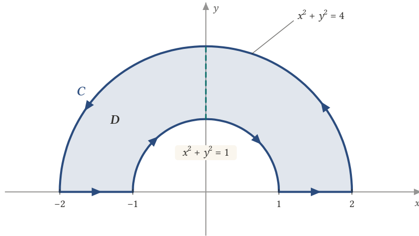
Şekil 13.5: Üst yarı düzlemde x^2 + y^2 = 1 ile x^2 + y^2 = 4 çemberleri arasındaki D bölgesi ve pozitif yönlü sınırı C : dış yay saat yönünün tersine, iç yay saat yönünde dolaşılır. Kesikli y eksenı parçası D 'yi iki basit bölgeye ayırır.
