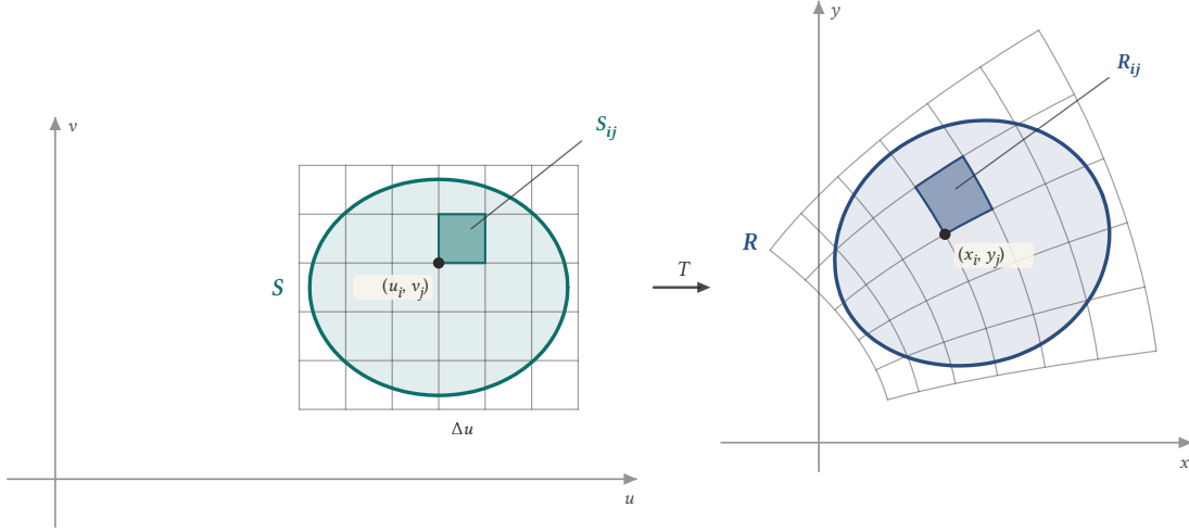
Şekil 9.4: S bölgesi \Delta u \times \Delta v boyutlu S_{ij} dikdörtgenlerine bölünür; T bu ızgarayı R üzerinde eğri bir ızgaraya götürür. Her R_{ij} parçasının alanı yaklaşık |\partial(x, y)/\partial(u, v)| \Delta u \Delta v olur (burada T(u, v) = (u^2 - v^2, 2uv) ).
