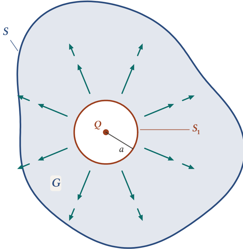
Şekil 18.5: Kesit görünüşü: Q yükü orijinde, S onu içine alan herhangi bir kapalı yüzey, S_1 ise orijin merkezli küçük a yarıçaplı küredir. \mathbf{E} alanı (oklar) orijinde tanımsızdır ama aradaki G bölgesinde \operatorname{div} \mathbf{E} = 0 olduğundan iki yüzeyin akısı eşittir.
