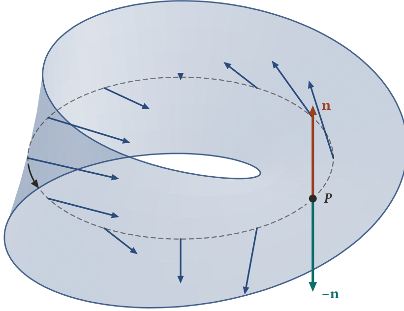
Şekil 16.3: Möbius şeridi. P noktasında seçilen \mathbf{n} normali orta çember (kesikli) boyunca sürekli olarak taşınırsa, bir tur sonra aynı P noktasına -\mathbf{n} olarak döner. Bu yüzden şeridin her noktasında sürekli değişen bir birim normal seçilemez.
