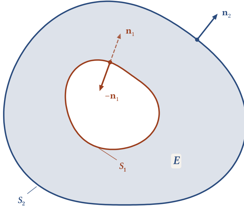
Şekil 18.4: Kesit görünüşü: E, içteki S_1 ile dıştaki S_2 kapalı yüzeyleri arasında kalır. E'nin dış normali S_2 üzerinde \mathbf{n}_2 'dir; S_1 üzerinde ise deliğin içine, yani -\mathbf{n}_1 yönüne bakar (kesikli ok, S_1 'in kendi dış normali \mathbf{n}_1 'dir).
