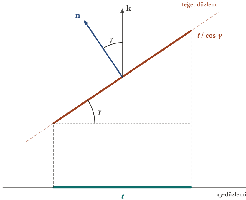
Şekil 5.3: Teğet düzlemi en dik doğrultusu boyunca kesen düşey düzlem. Düzlem xy -düzlemiyle \gamma açısı yapar; bu, \mathbf{n} normali ile \mathbf{k} arasındaki açıdır. Bu doğrultudaki \ell uzunluğundaki bir gölge düzlemde \ell/\cos \gamma uzunluğuna karşılık gelir; buna dik (yatay) doğrultudaki uzunluklar değişmez.
