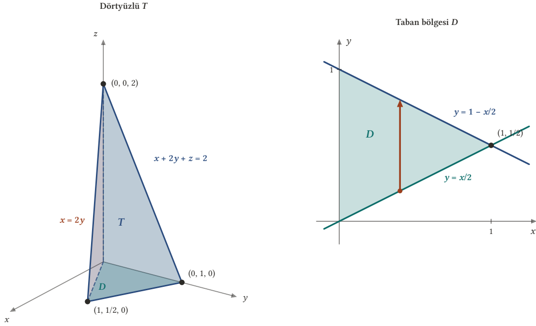
Şekil 2.6: Solda x=0 , z=0 , x=2y ve x+2y+z=2 düzlemlerinin sınırladığı T dörtyüzlüsü. Sağda tabanı olan D üçgeni: x+2y+z=2 düzlemi xy -düzlemini y=1-x/2 doğrusu boyunca keser.
