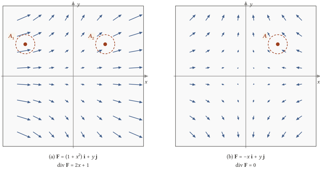
Şekil 14.4: (a) A_1 = (-1, 5; 1) noktasında \text{div } \mathbf{F} = -2 < 0 : kesikli çemberin içine giren oklar çıkanlardan uzundur, net akış içeri doğrudur. A_2 = (1, 1) noktasında \text{div } \mathbf{F} = 3 > 0 : çıkan oklar daha uzundur, net akış dışarı doğrudur. (b) \text{div } \mathbf{F} = 0 her yerde; A = (1, 1) çevresine giren ve çıkan akış dengededir.
