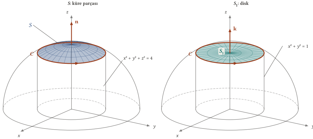
Şekil 17.5: Solda x^2 + y^2 + z^2 = 4 küresinin x^2 + y^2 = 1 silindiri içinde kalan üst parçası S , sağda z = \sqrt{3} düzlemindeki birim disk S_1 . İkisinin sınırı aynı C çemberidir ( x^2 + y^2 = 1 , z = \sqrt{3} ) ve yukarı yönlendirildiklerinde C 'ye aynı yönü verirler.
