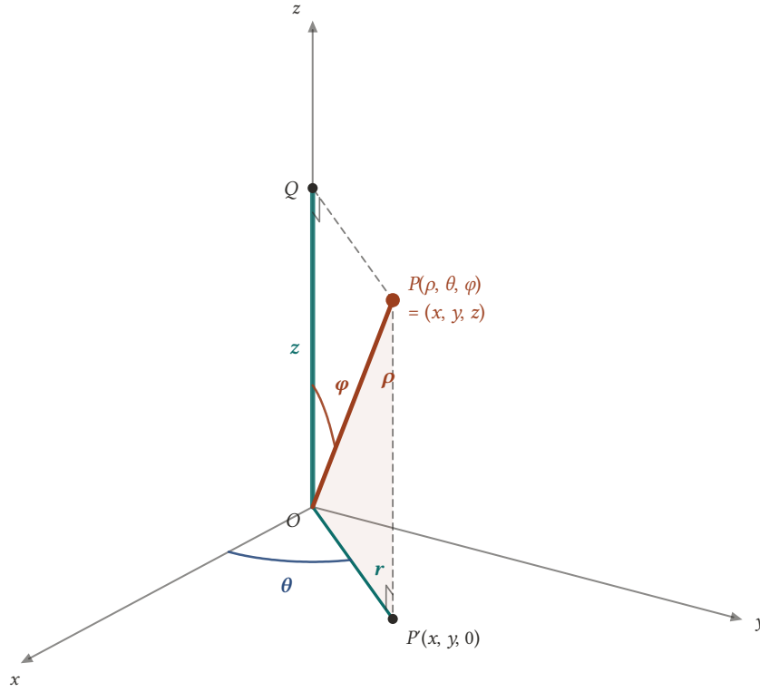
Şekil 8.1: P noktasının küresel koordinatları: \rho = |OP| orijine uzaklık, \varphi pozitif z eksenine OP arasındaki açı, \theta ise P izdüşümünün kutupsal açısıdır. OQP ve OP'P dik üçgenlerinden z = \rho \cos \varphi ve r = |OP'| = \rho \sin \varphi okunur.
