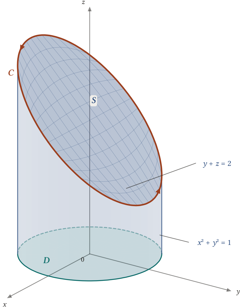
Şekil 17.3: y + z = 2 düzlemi x^2 + y^2 = 1 silindirin C elipsinde keser. S , düzlemin C içinde kalan parçasıdır; gölgesi birim daire D 'dir. C yukarıdan bakınca saat yönünün tersine dolandır, bu yüzden S yukarı yönlendirilir.
