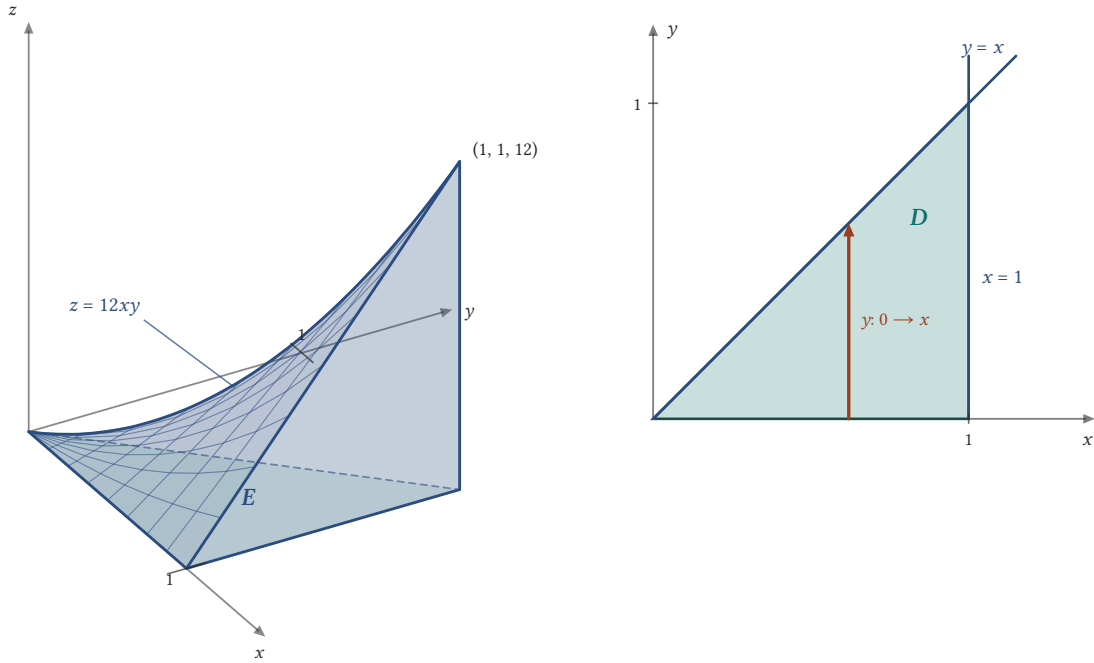
Şekil 6.3: Solda E cismi: altta z = 0 , üstte z = 12xy yüzeyi, yanlarda y = x ve x = 1 düzlemleri (dikey eksen 1/10 ölçeklidir). Sağda E 'nin xy -düzlemine izdüşümü olan D üçgeni; ok, sabit x için y 'nin 0'dan x 'e değiştiğini gösterir.
