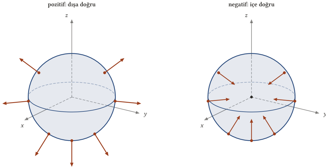
Şekil 16.5: Kapalı bir yüzey olan kürenin iki yönlendirmesi. Solda normaller kürenin içindeki bölgeden dışa doğru bakar (pozitif yönlendirme), sağda içe doğru bakar (negatif yönlendirme).
