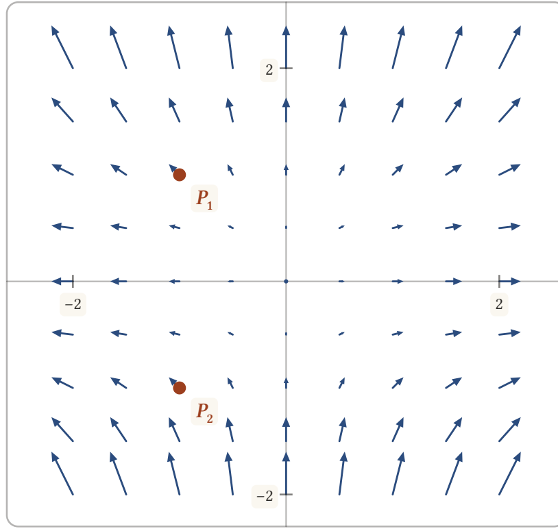
Şekil 18.8: \mathbf{F}(x, y) = x \mathbf{i} + y^2 \mathbf{j} alanı (oklar aynı oranda kısaltıldı) ve P_1(-1, 1) , P_2(-1, -1) noktaları.
