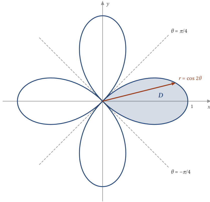
Şekil 3.6: r = \cos 2\theta dört yapraklı gülü. Sağdaki yaprak \theta = -\pi/4 ile \theta = \pi/4 ışınları arasındadır; bu açılardaki her ışın orijinden çıkıp eğriye r = \cos 2\theta da ulaşır.
