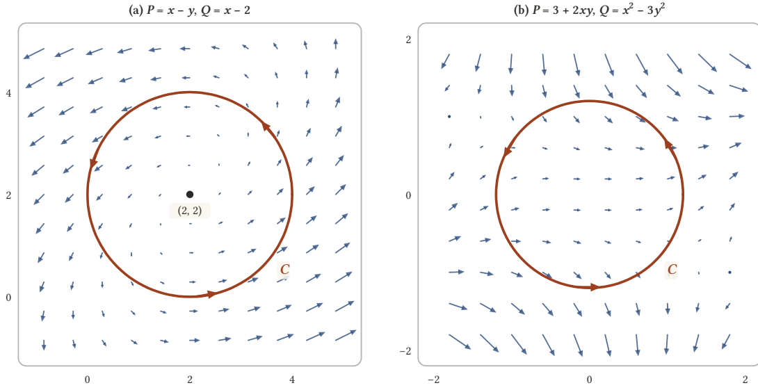
Şekil 12.7: Konservatiflik ölçütünün iki örneğindeki alanlar; okların hepsi aynı oranda kısaltılmıştır. (a) Merkezi (2, 2), yarıçapı 2 olan C çemberi boyunca oklar hep dolaşılma yönüne bakar ve integral 8\pi çıkar. (b) Konservatif alanda C çemberinin bazı yerlerinde oklar dolaşılma yönüne, bazı yerlerinde ters yöne bakar; katkılar birbirini götürür ve integral 0'dır.
