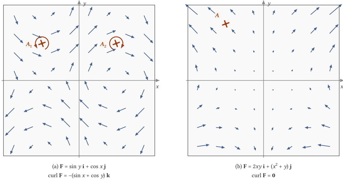
Şekil 14.3: İki düzlem akışı (alanlar z 'den bağımsızdır, z -bileşenleri 0'dır). (a) A_1 = (-\pi/2, \pi/2) noktasında \text{curl } \mathbf{F} = \mathbf{k} olduğundan buraya konan küçük çark saatin tersi yönünde, A_2 = (\pi/2, \pi/2) noktasında \text{curl } \mathbf{F} = -\mathbf{k} olduğundan saat yönünde döner. (b) Her yerde \text{curl } \mathbf{F} = \mathbf{0} olduğundan A noktasındaki çark akışla birlikte sürüklenir ama kendi ekseninde dönmez.
