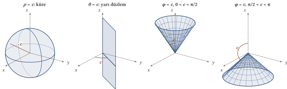
Şekil 8.3: Küresel koordinatlarda bir koordinatı sabitleyen yüzeyler. \rho = c merkezi orijinde olan bir küre, \theta = c kenarı z eksenine olan düşey bir yarı düzlem, \phi = c ise eksen z eksenine olan bir yarı konidir: c < \pi/2 iken yukarı, c > \pi/2 iken aşağı açılır.
