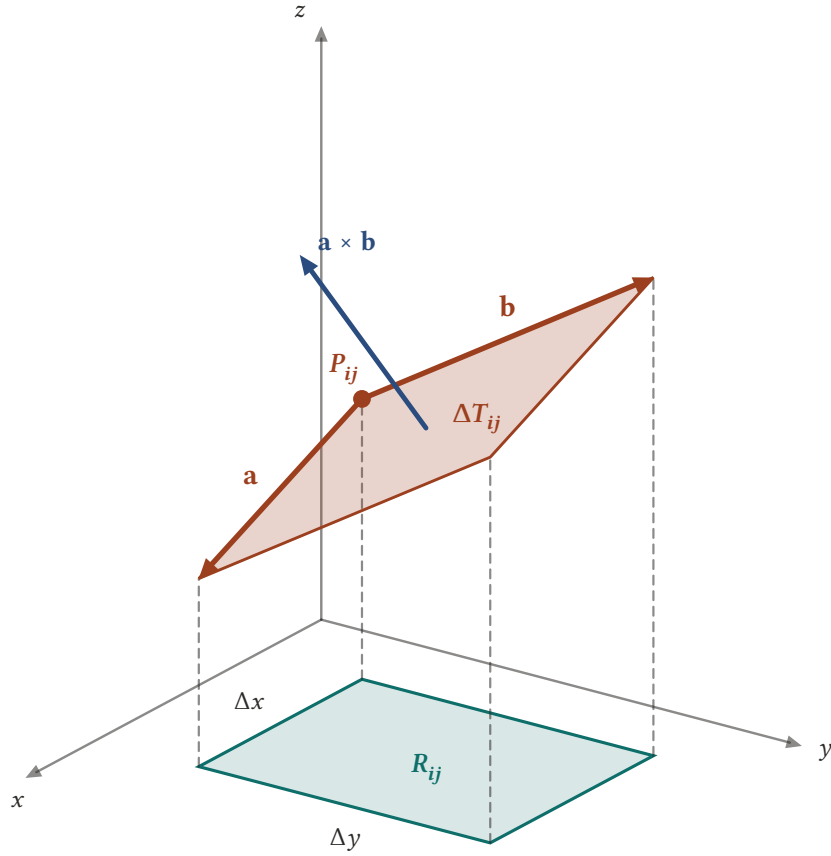
Şekil 5.2: Teğet düzlemin R_{ij} üstündeki parçası, P_{ij} köşesinden çıkan \mathbf{a} = \Delta x \mathbf{i} + f_x \Delta x \mathbf{k} ve \mathbf{b} = \Delta y \mathbf{j} + f_y \Delta y \mathbf{k} vektörlerinin gerdiği paralelkenardır. \mathbf{a} ve \mathbf{b} 'nin xy -düzlemine izdüşümleri R_{ij} 'nin kenarlarıdır; \mathbf{a} \times \mathbf{b} paralelkenara diktir ve uzunluğu alanını verir.
