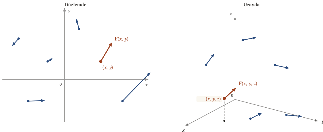
Şekil 10.1: Bir vektör alanı her noktaya bir vektör atar. \mathbf{F}(x, y) vektörünü başlangıcı (x, y) noktası olan bir okla, uzayda \mathbf{F}(x, y, z) vektörünü başlangıcı (x, y, z) olan bir okla çizeriz. Birkaç temsilci noktadaki oklar alanın genel görünüşünü verir.
