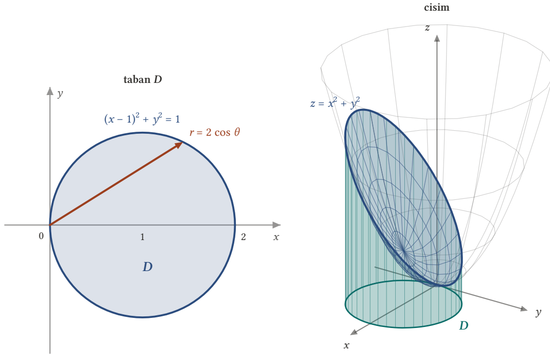
Şekil 3.7: Sol: taban D , (x-1)^2 + y^2 = 1 diskidir; kutupsal denklemi r = 2 \cos \theta , -\pi/2 \leq \theta \leq \pi/2 . Sağ: x^2 + y^2 = 2x silindirin içinde, xy -düzleminin üstünde ve z = x^2 + y^2 paraboloidinin altında kalan cisim.
