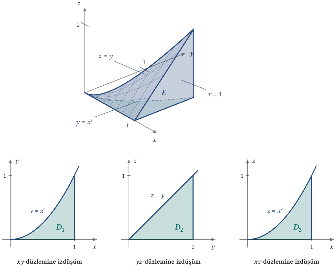
Şekil 6.6: Üstte E cismi; altta z = 0 , üstte z = y düzlemi, önde x = 1 düzlemi, arkada y = x^2 parabolik silindiri. Altta E 'nin üç koordinat düzlemine izdüşümleri: D_1 ( 0 \leq y \leq x^2 ), D_2 ( 0 \leq z \leq y \leq 1 ) ve D_3 ( 0 \leq z \leq x^2 ).
