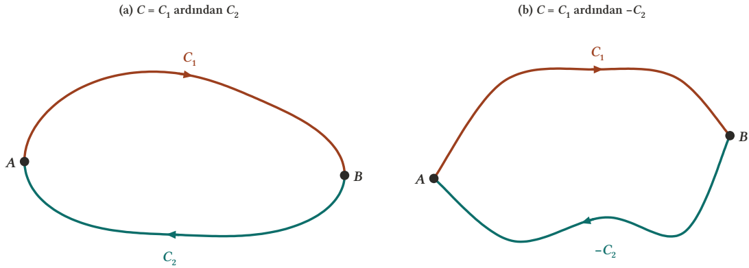
Şekil 12.3: (a) Kapalı bir C yolu, üzerindeki iki A, B noktasında ikiye ayrılır: A 'dan B 'ye giden C_1 ve B 'den A 'ya dönen C_2 . (b) A 'dan B 'ye giden iki yoldan C_1 'i izleyip C_2 'yi ters yönde ( -C_2 ) geri dönmek kapalı bir yol verir.
