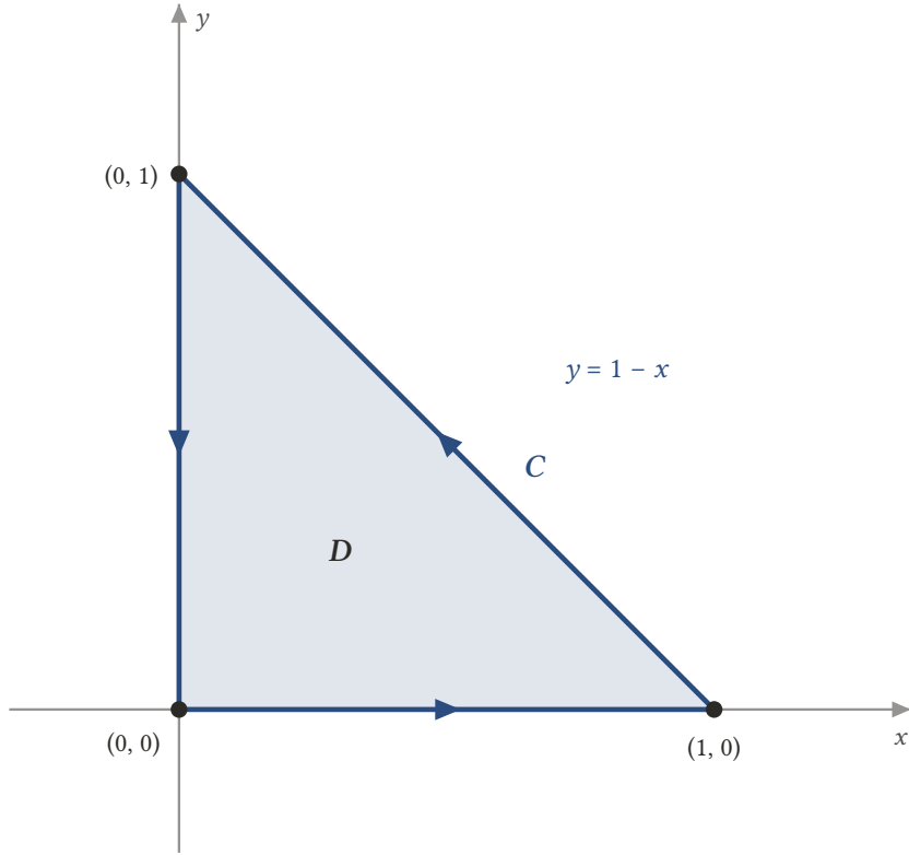
Şekil 13.3: Üçgen C eğrisi (0, 0) \rightarrow (1, 0) \rightarrow (0, 1) \rightarrow (0, 0) sırasıyla, yani saat yönünün tersine dolaşılır; sınırladığı D bölgesi 0 \leq x \leq 1, 0 \leq y \leq 1 - x ile verilir.
