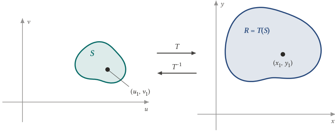
Şekil 9.1: T dönüşümü uv -düzlemindeki S bölgesini xy -düzlemindeki R = T(S) bölgesine, her (u_1, v_1) noktasını da görüntüsü (x_1, y_1) noktasına götürür. T bire bir ise T^{-1} geri dönüşü sağlar. Burada T(u, v) = (u^2 - v^2, 2uv) alınmıştır.
