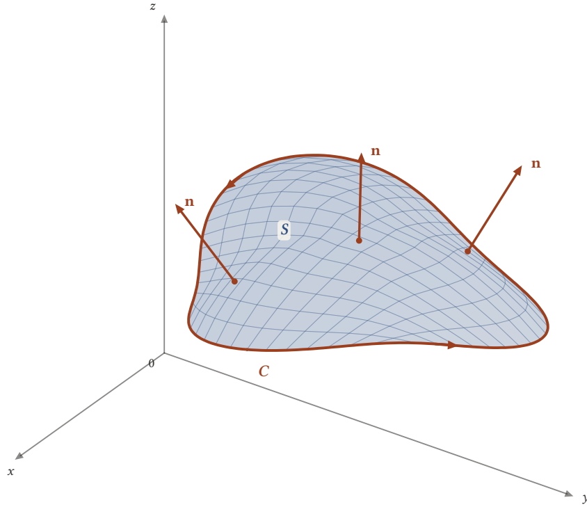
Şekil 17.1: Birim normali \mathbf{n} olan yönlendirilmiş S yüzeyi ve sınır eğrisi C 'nin pozitif yönü. Başı \mathbf{n} yönünde olan biri C üzerinde oklar yönünde yürürse yüzey hep solunda kalır. Burada \mathbf{n} yukarı baktığından bu yön, yukarıdan bakınca saat yönünün tersidir.
