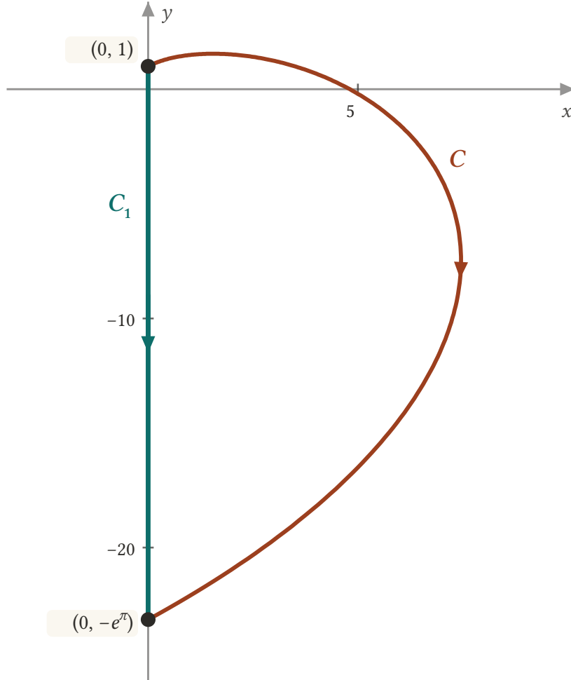
Şekil 12.8: C eğrisi \mathbf{r}(t) = e^t \sin t \mathbf{i} + e^t \cos t \mathbf{j} , 0 \leq t \leq \pi , (0, 1) noktasından sağa doğru açılıp (0, -e^\pi) \approx (0, -23, 1) noktasına iner. C_1 , aynı iki noktayı birleştiren düşey doğru parçasıdır. Eksenlerdeki ölçekler farklıdır.
