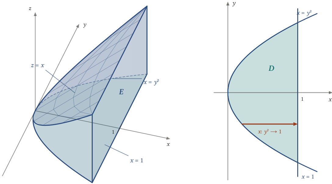
Şekil 6.7: Solda E cismi: altta z = 0 , üstte z = x düzlemi; yan yüzleri x = 1 düzlemi ve x = y^2 parabolik silindiridir. Sağda izdüşümü D : sabit y için x , y^2 'den 1'e değişir.
