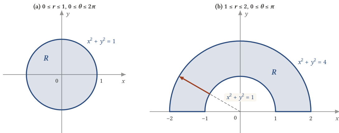
Şekil 3.1: Kutupsal koordinatlarla kolay yazılan iki bölge. (a) Birim disk: 0 \leq r \leq 1 , 0 \leq \theta \leq 2\pi . (b) Üst yarı düzlemde x^2 + y^2 = 1 ile x^2 + y^2 = 4 çemberleri arasındaki yarım halka: 1 \leq r \leq 2 , 0 \leq \theta \leq \pi . Okla gösterilen ışın bölgeye r = 1 'de girer, r = 2 'de çıkar.
