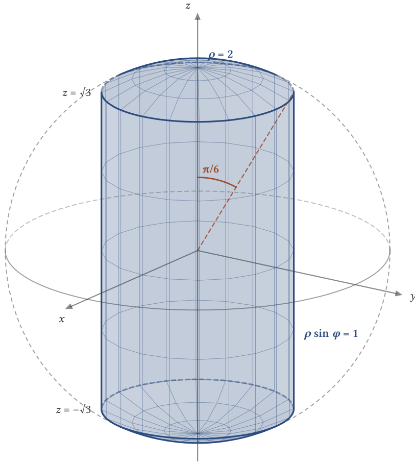
Şekil 8.7: \rho \leq 2 , \rho \leq \csc \varphi cismi: 2 yarıçaplı topun (kesikli) x^2 + y^2 \leq 1 silindiri içinde kalan kısmı. Yan yüzey \rho \sin \varphi = 1 silindiri, alt ve üst kapaklar \rho = 2 küresinin parçalarıdır; ikisi z = \pm\sqrt{3} çemberlerinde, yani \varphi = \pi/6 ve \varphi = 5\pi/6 'da birleşir.
