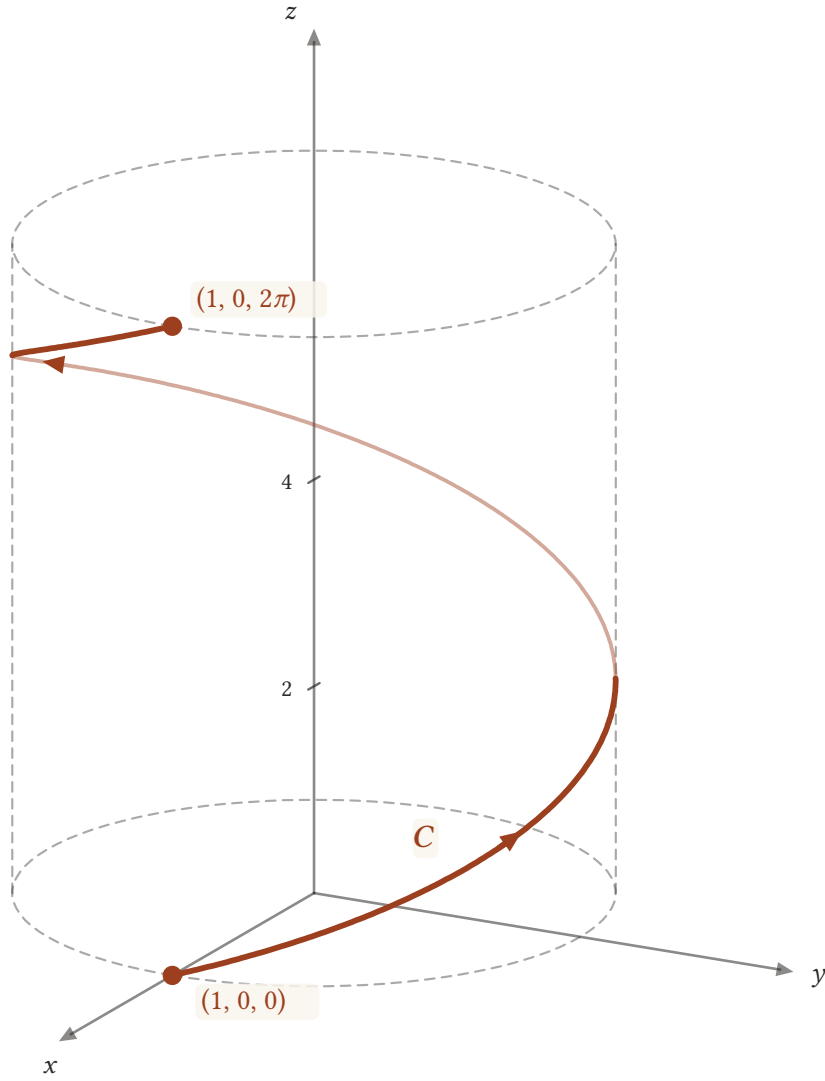
Şekil 11.3: x = \cos t , y = \sin t , z = t ( 0 \leq t \leq 2\pi ) dairesel helisi x^2 + y^2 = 1 silindirin üzerinde bir tam tur atarak (1, 0, 0) noktasından (1, 0, 2\pi) noktasına çıkar. Silindirin arka yüzündeki kısmı soluk çizilmiştir; şekil fazla uzamasın diye z eksenini kısaltılmış ölçekle çizilmiştir.
