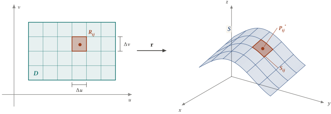
Şekil 16.1: \mathbf{r} , uv -düzlemindeki D dikdörtgenini S yüzeyine götürür. D 'nin \Delta u \times \Delta v boyutlu her R_{ij} alt dikdörtgeni, yüzeyde bir S_{ij} yamasına karşılık gelir. Riemann toplamında f , yamadan seçilen bir P_{ij}^* noktasında hesaplanır ve yamanın alanıyla çarpılır.
