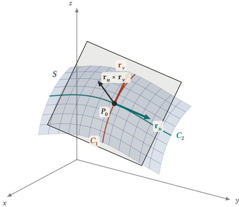
Şekil 15.7: P_0 'dan geçen C_1 (u = u_0) ve C_2 (v = v_0) koordinat eğrilerinin teğet vektörleri \mathbf{r}_v ve \mathbf{r}_u 'dur. Bu iki vektörü içeren düzlem teğet düzlemdir (gri); \mathbf{r}_u \times \mathbf{r}_v ona diktir.
