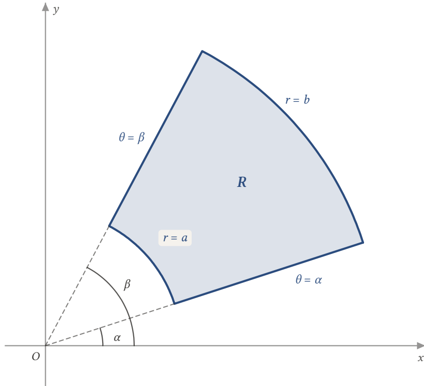
Şekil 3.2: Kutupsal dikdörtgen R = \{(r, \theta) \mid a \leq r \leq b, \alpha \leq \theta \leq \beta\} : iki çember yayı ile iki ışın parçasının sınırladığı halka dilimi.
