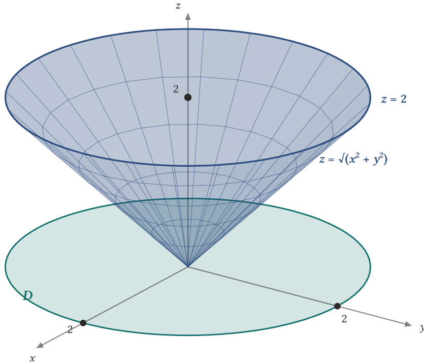
Şekil 7.7: Altta z = \sqrt{x^2 + y^2} konisi, üstte z = 2 düzlemiyle sınırlanan cisim. xy -düzlemine izdüşümü D : x^2 + y^2 \leq 4 diskidir; silindirik koordinatlarda cisim 0 \leq r \leq 2 , r \leq z \leq 2 ile verilir.
