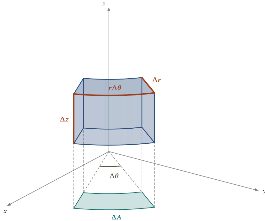
Şekil 7.4: Silindirik bir kutu: tabanı alanı \Delta A olan bir kutupsal dikdörtgen, yüksekliği \Delta z 'dir. Kenarları yaklaşık \Delta r , r \Delta \theta ve \Delta z olduğundan hacmi yaklaşık r \Delta r \Delta \theta \Delta z 'dir.
