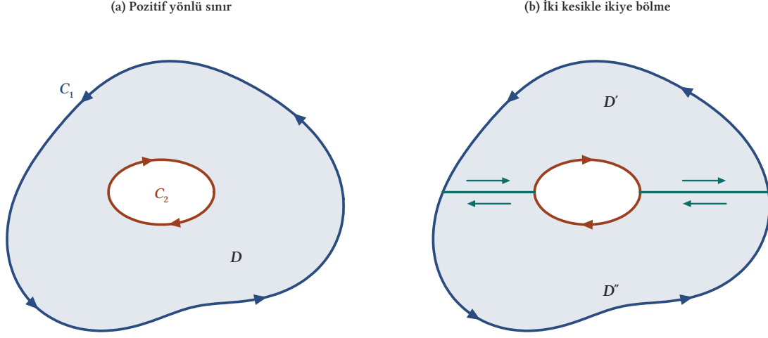
Şekil 13.6: (a) Delikli D bölgesinin pozitif yönlü sınırı: dış eğri C_1 saat yönünün tersine, iç eğri C_2 saat yönünde dolaşılır; iki durumda da D solda kalır. (b) İki kesik D 'yi D' ve D'' parçalarına ayırır. Her kesik iki parçanın sınırında zıt yönlerde dolaşıldığından kesikler üzerindeki integraller birbirini götürür.
