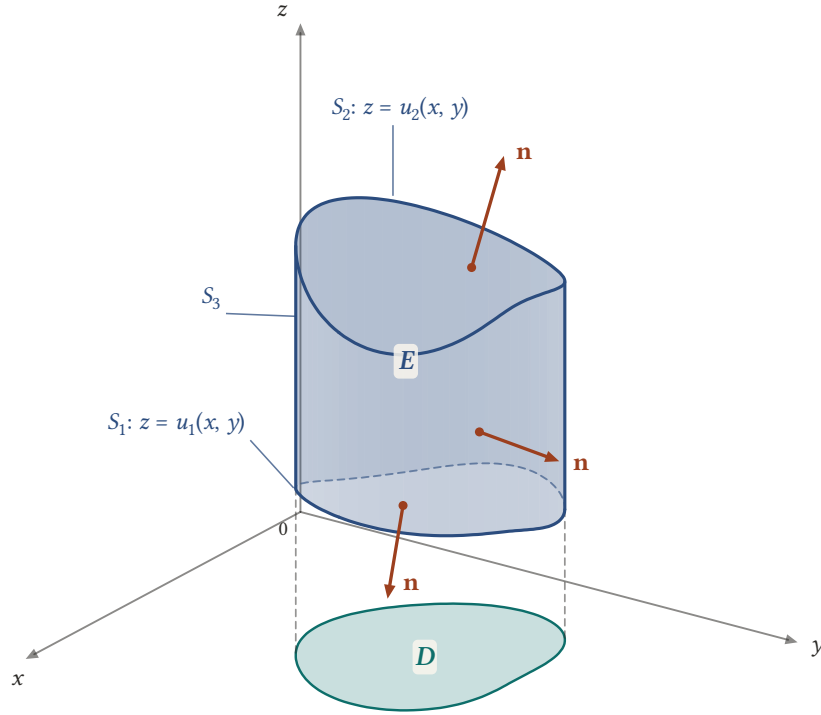
Şekil 18.2: E'ye tip 1 bölge olarak bakmak. Sınır üç parçadır: alttaki S_1 , üstteki S_2 ve D'nin sınırı üzerinde yükselen düşey S_3 . Dış normal S_2 'de yukarı, S_1 'de aşağı bakar; S_3 'te yataydır, bu yüzden orada \mathbf{k} \cdot \mathbf{n} = 0 olur.
