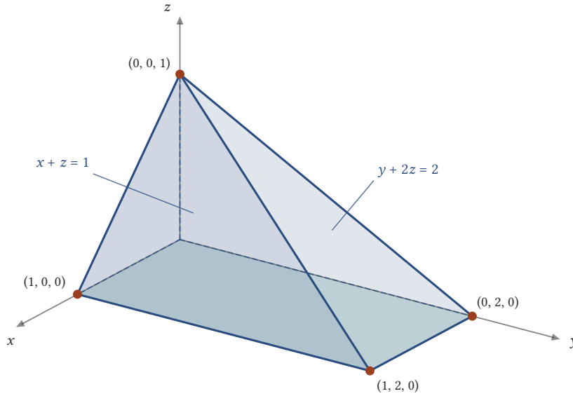
Şekil 6.8: Ardışık integralin cismi: tabanı xy -düzlemindeki [0, 1] \times [0, 2] dikdörtgeni, tepesi (0, 0, 1) olan bir piramit. Eğik yüzleri x + z = 1 ve y + 2z = 2 düzlemleridir; arka yüzleri koordinat düzlemleridir.
