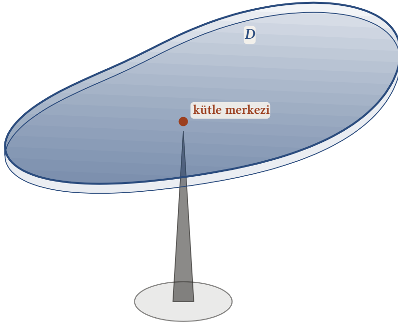
Şekil 4.2: Levha, bütün kütlesi kütle merkezinde toplanmış gibi davranır: kütle merkezinin altından bir iğne ucuyla desteklenen levha yatay olarak dengede kalır. Koyu bölgeler daha yoğundur ve kütle merkezi o yana kayar.
