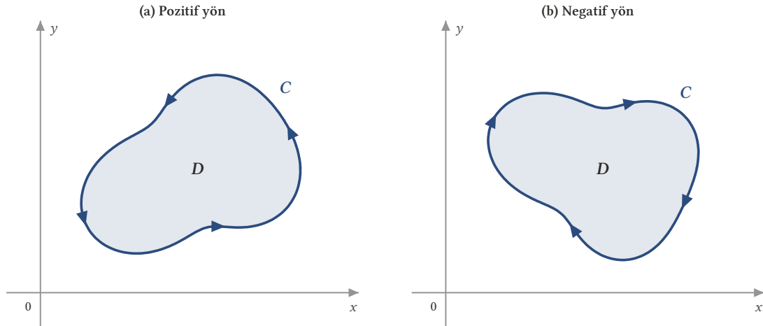
Şekil 13.1: (a) Pozitif yönlü C eğrisi saat yönünün tersine bir kez dolaşılır; eğri boyunca ilerleyen biri D bölgesini hep solunda görür. (b) Ters yönde dolaşılan eğri negatif yönlüdür: D bu kez hep sağda kalır.
