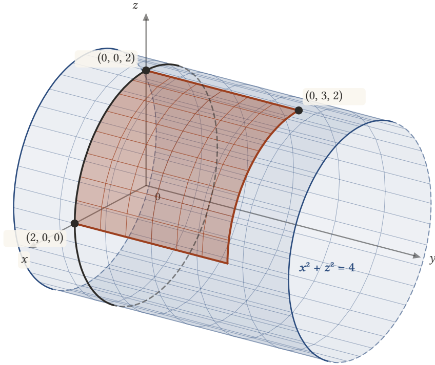
Şekil 15.2: x^2 + z^2 = 4 silindirin bir parçası (açık) ve 0 \leq u \leq \pi/2 , 0 \leq v \leq 3 parametre bölgesinin görüntüsü olan çeyrek silindir (koyu). Siyah çember, v = 0 koordinat eğrisidir; (2, 0, 0) ve (0, 0, 2) noktalarından geçer.
