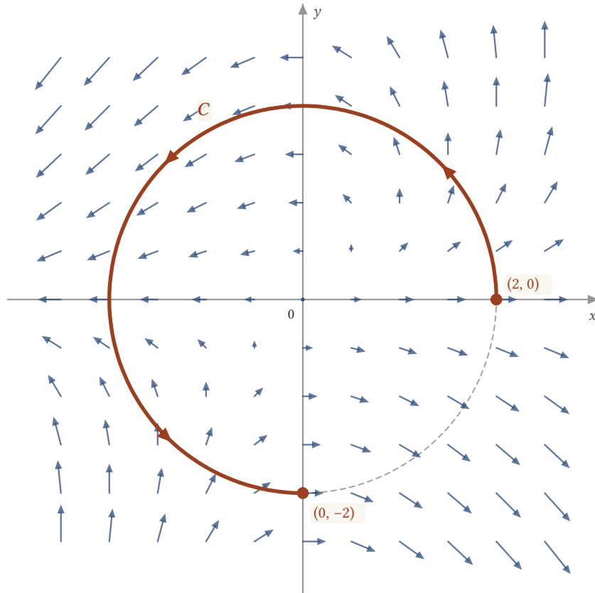
Şekil 11.8: \mathbf{F}(x, y) = (x - y)\mathbf{i} + xy\mathbf{j} alanı ve x^2 + y^2 = 4 çemberinin (2, 0) noktasından saat yönünün tersine (0, -2) noktasına giden C yayı. Okların yönü \mathbf{F} 'nin yönüdür; uzunlukları |\mathbf{F}| ile artar ama okunaklı kalsın diye orantılı çizilmemiştir.
