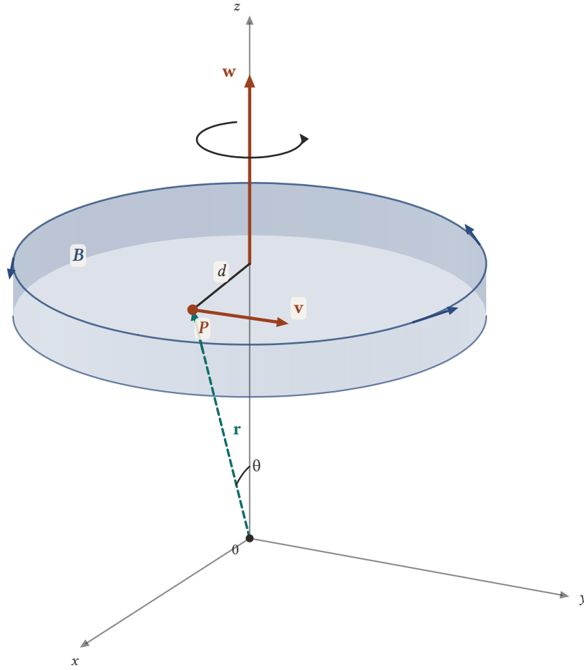
Şekil 14.7: B cismi z eksenini etrafında \omega açısal hızıyla döner; \mathbf{w} = \omega \mathbf{k} . P noktasının eksenine uzaklığı d = |\mathbf{r}| \sin \theta , hızı ise eksenine ve \mathbf{r} 'ye dik, büyüklüğü \omega d olan \mathbf{v} vektörüdür.
