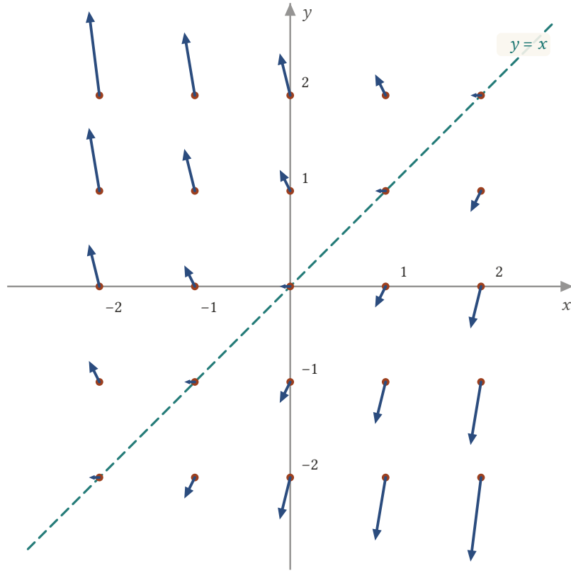
Şekil 10.8: F(x, y) = -\frac{1}{2} \mathbf{i} + (y - x) \mathbf{j} alanının tam sayı koordinatlı noktalarındaki vektörleri (hepsi aynı oranda kısaltılmış). Oklar y = x doğrusu üzerinde yatay ve sola doğrudur; doğrunun üstünde yukarı, altında aşağı eğilir ve doğrudan uzaklaştıkça uzar.
