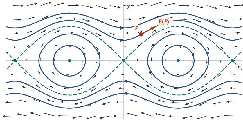
Şekil 10.5: \mathbf{F}(x, y) = y\mathbf{i} + \sin x\mathbf{j} alanı (ince oklar, kısaltılmış) ve birkaç akış çizgisi (mavi). Akış çizgisi üzerindeki bir P noktasında alanın vektörü \mathbf{F}(P) eğriye teğettir ve parçacığın o andaki hızını verir. Yeşil noktalarda \mathbf{F} = \mathbf{0} 'dir; kesikli eğriler, kapalı akış çizgilerini dalgali olanlardan ayıran akış çizgileridir.
