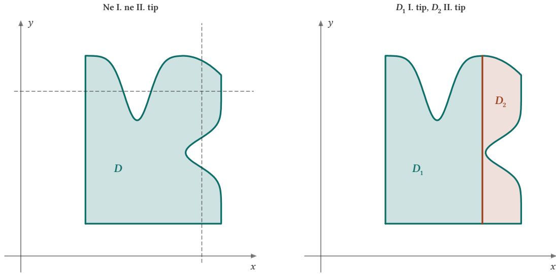
Şekil 2.8: Solda ne I. ne II. tip olan bir D bölgesi: kesikli dikey doğru sınırı dört kez, kesikli yatay doğru da dört kez keser. Sağda D bir dikey doğru parçasıyla iki parçaya ayrılmıştır: D_1 I. tip, D_2 II. tip bir bölgedir ve iki parça yalnız bu doğru parçası boyunca ortaktır.
