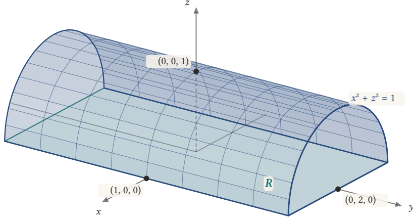
Şekil 1.4: z = \sqrt{1-x^2} yüzeyi, eksen y eksenine ve yarıçapı 1 olan silindirin üst yarısıdır. R = [-1, 1] \times [-2, 2] üzerindeki cismin her kesiti alanı \pi/2 olan bir yarım dairedir ve cismin uzunluğu 4'tür.
