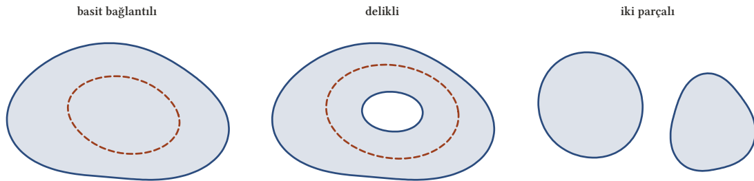
Şekil 12.6: Soldaki bölge basit bağlantılıdır: içindeki her basit kapalı eğri (kesikli) yalnız bölgenin noktalarını çevreler. Ortadaki bölgede deliği dolanan kesikli eğri, bölgede olmayan noktaları çevreler; sağdaki küme ise bağlantılı bile değildir. Bu iki küme basit bağlantılı değildir.
