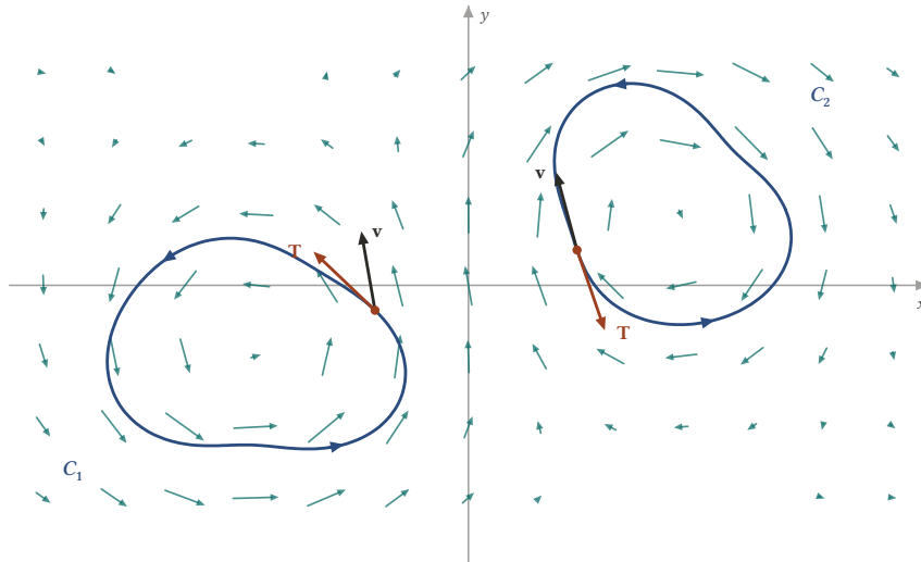
Şekil 17.6: Bir akışkanın hız alanı \mathbf{v} (oklar) ve iki kapalı eğri. C_1 boyunca \mathbf{v} çoğunlukla eğrinin \mathbf{T} teğetiyle aynı yöne akar, \mathbf{v} \cdot \mathbf{T} > 0 olur ve dolanım pozitiftir. C_2 boyunca akış eğrinin yönüne karşıdır, dolanım negatiftir.
