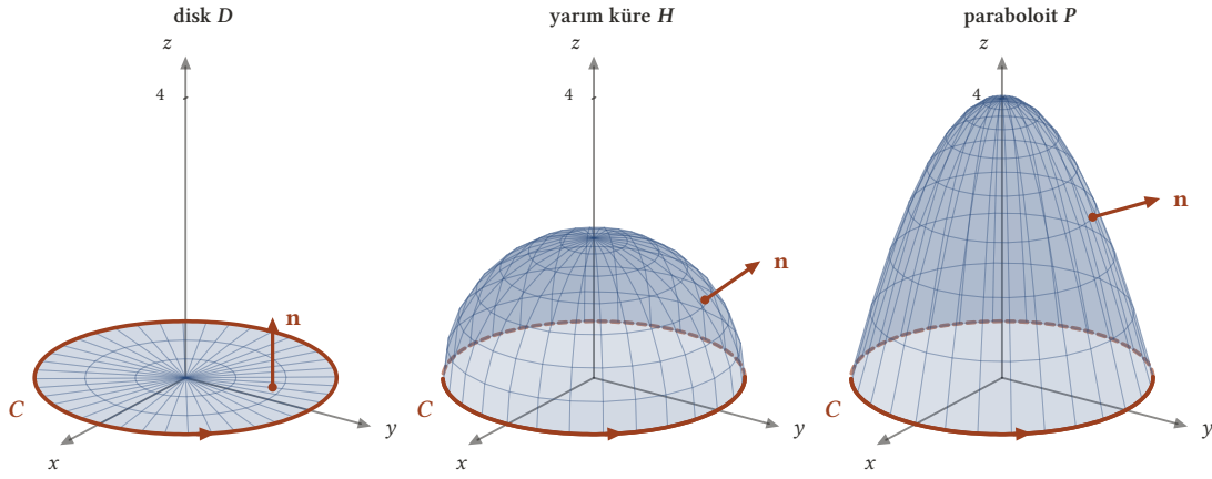
Şekil 17.4: Sınırı aynı C çemberi ( x^2 + y^2 = 4, z = 0 ) olan üç yüzey: x^2 + y^2 \leq 4 diski, x^2 + y^2 + z^2 = 4 küresinin üst yarısı ve z = 4 - x^2 - y^2 paraboloidinin xy -düzleminin üstündeki parçası. Üçü de yukarı yönlendirildiğinde C 'ye aynı pozitif yönü verir.
