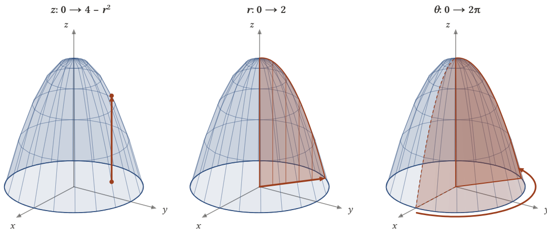
Şekil 7.5: Ardışık integralin cismi adım adım taradığını gösterir. Solda r ve \theta sabitken z tabandan paraboloidin üstüne kadar uzanan dikey bir çizgiyi tarar; ortada \theta sabitken bu dikey çizgiler r = 0 'dan r = 2 'ye kayarak dikey bir dilim oluşturur; sağda dilim z eksenini etrafında \theta = 0 'dan 2\pi 'ye döner ve bütün cismi süpürür.
