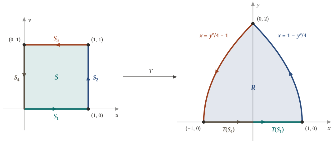
Şekil 9.2: x = u^2 - v^2 , y = 2uv dönüşümü birim karenin S_1 , S_2 , S_3 , S_4 kenarlarını aynı renkteki sınır parçalarına götürür. Kare saat yönünün tersine dolaşılınca R 'nin sınırı da saat yönünün tersine dolaşılır.
