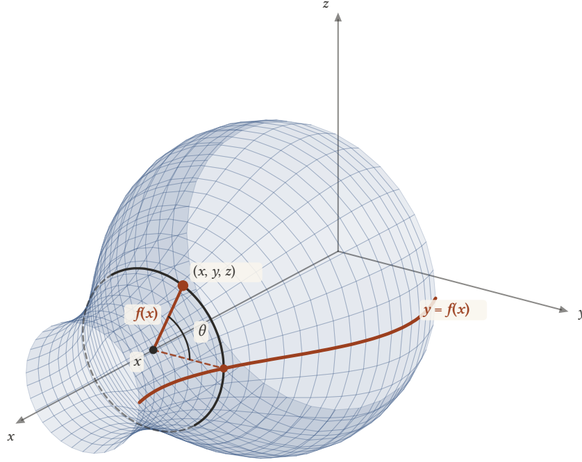
Şekil 15.5: y = f(x) eğrisi x eksenine çevresinde dönerken eğrinin her noktası, x eksenine dik düzlemde f(x) yarıçaplı bir çember çizer. y ekseninin yönünden \theta kadar dönmüş nokta (x, f(x) \cos \theta, f(x) \sin \theta) olur.
