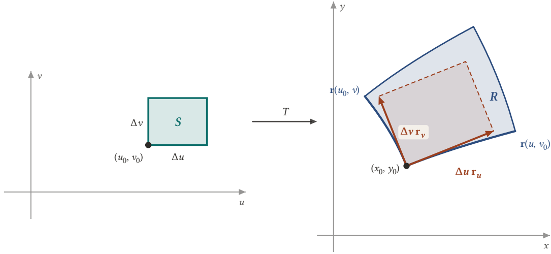
Şekil 9.3: Kenarları \Delta u ve \Delta v olan küçük S dikdörtgeninin görüntüsü eğri kenarlı bir R bölgesidir. R , (x_0, y_0) köşesindeki \Delta u \mathbf{r}_u ve \Delta v \mathbf{r}_v teğet vektörlerinin gerdiği paralelkenara (kesikli) yakındır. Burada T(u, v) = (u^2 - v^2, 2uv) , S = [1; 1.5] \times [0.4; 0.8] alınmıştır.
