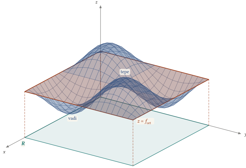
Şekil 1.7: Engibeli bir z = f(x, y) yüzeyi ve z = f_{\text{ort}} düzlemi (turuncu). Düzlemin üstünde kalan tepeler kesilip altında kalan vadilere doldurulursa yüzey tümüyle düzleşir; tabanı R , yüksekliği f_{\text{ort}} olan kutunun hacmi yüzeyin altındaki hacme eşittir.
