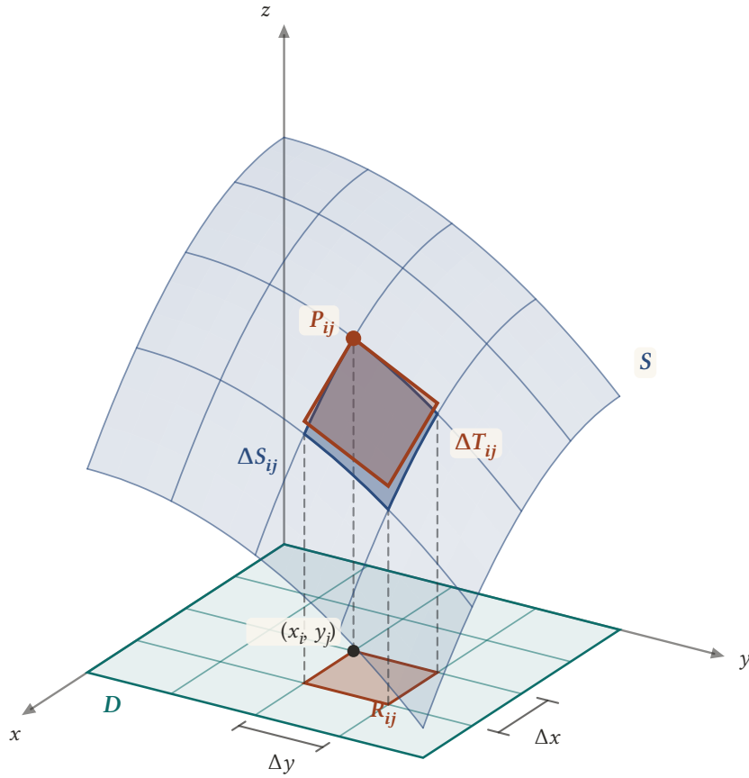
Şekil 5.1: D dikdörtgeni \Delta x \times \Delta y boyutlu alt dikdörtgenlere bölünür. R_{ij} 'nin sol alt köşesi (x_i, y_j) 'nin üstündeki P_{ij} noktasında S 'ye teğet olan düzlemin R_{ij} üstündeki parçası bir paralelkenardır (turuncu). Alanı \Delta T_{ij} , yüzeyin R_{ij} üstündeki parçasının (mavi) alanı \Delta S_{ij} 'ye yakındır.
