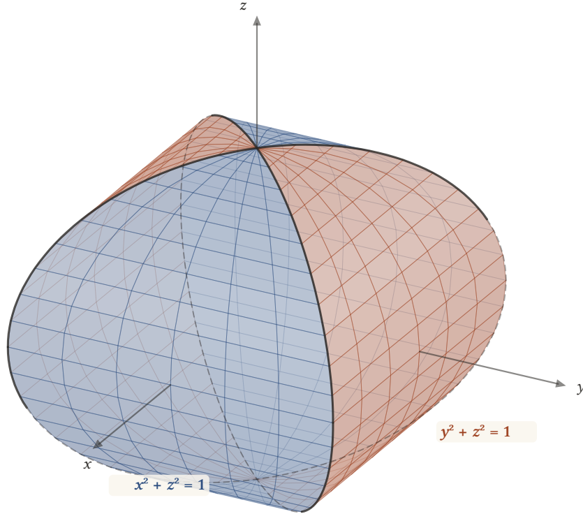
Şekil 5.7: y^2 + z^2 \leq 1 ve x^2 + z^2 \leq 1 eşitsizliklerini birlikte sağlayan cismin yüzeyi. Mavi parçalar x^2 + z^2 = 1 silindirinden ( |y| \leq |x| ), turuncu parçalar y^2 + z^2 = 1 silindirinden ( |x| \leq |y| ) gelir; iki silindir y = \pm x düzlemlerindeki elipsler boyunca birleşir.
