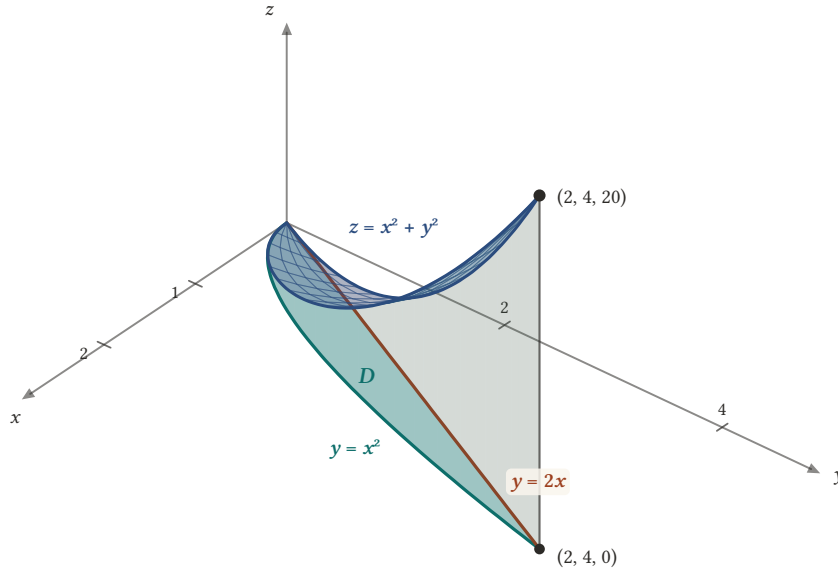
Şekil 2.4: Örnekteki cisim: tabanı xy -düzlemindeki D bölgesi, tavanı z = x^2 + y^2 paraboloidi, yan yüzleri y = 2x düzlemi ile y = x^2 parabolik silindridir. En yüksek noktası (2, 4, 20) 'dir; şekil sığsın diye z eksenini kısaltılarak çizilmiştir.
