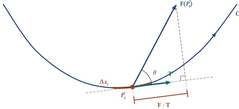
Şekil 11.5: Parçacık turuncu alt yayı geçerken yaklaşık \mathbf{T} birim teğet vektörü yönünde \Delta s_i kadar ilerler. \mathbf{F} 'nin bu yöndeki bileşeni \mathbf{F} \cdot \mathbf{T} = |\mathbf{F}| \cos \theta , yani \mathbf{F} 'nin teğet doğrusu üzerindeki dik izdüşümünün uzunluğudur; bu parçada yapılan iş yaklaşık (\mathbf{F} \cdot \mathbf{T}) \Delta s_i olur.
