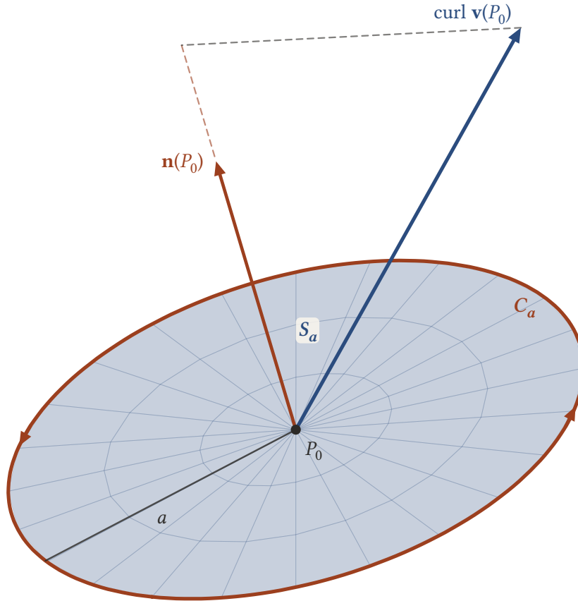
Şekil 17.7: P_0 merkezli, a yarıçaplı ve birim normali \mathbf{n} olan küçük S_a diski ile sınırı C_a . C_a etrafındaki dolanım yaklaşık olarak (\text{curl } \mathbf{v}(P_0) \cdot \mathbf{n}) \pi a^2 'dir; çarpandaki iç çarpım, \text{curl } \mathbf{v} 'nin \mathbf{n} doğrultusundaki bileşenidir (kesikli izdüşüm).
