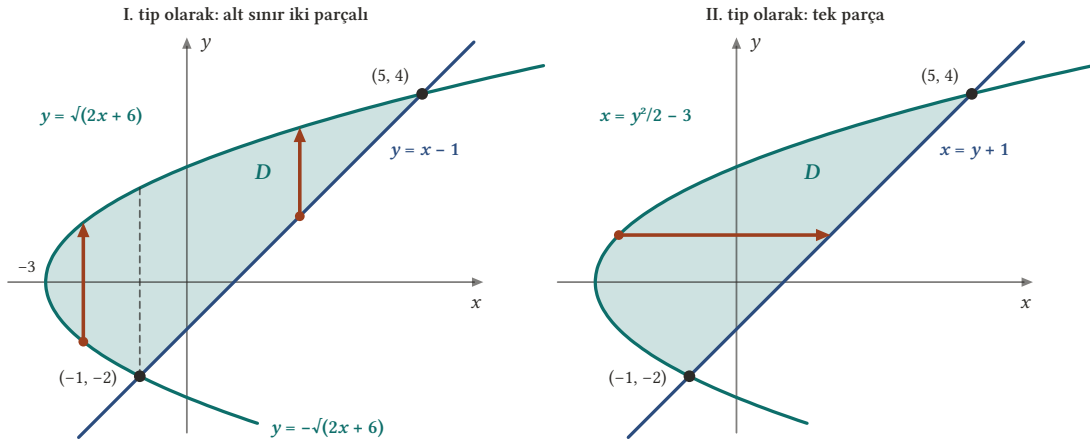
Şekil 2.5: y = x - 1 doğrusu ile y^2 = 2x + 6 parabolü arasındaki D bölgesi. Solda düşey oklar: x = -1 'in solunda alt sınır parabolün alt kolu, sağında doğrudur; bu yüzden I. tip yazım iki integral ister. Sağda yatay oklar hep parabolden girip doğrudan çıkar: II. tip yazım tek integraldir.
