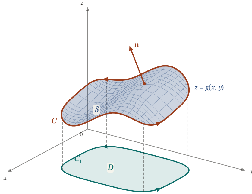
Şekil 17.2: S yüzeyi z = g(x, y) grafiği olduğunda gölgesi D bölgesidir ve S'nin sınırı C, D'nin sınırı C_1 'in tam üstünde durur. S yukarı yönlendirilmişse C'nin pozitif yönü, C_1 'in pozitif yönünün (saat yönünün tersinin) üstündeki yöndür.
