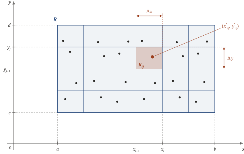
Şekil 1.1: R = [a, b] \times [c, d] dikdörtgeni m = 6 , n = 4 için 24 alt dikdörtgene bölünmüştür. Turuncu R_{ij} alt dikdörtgeninin kenarları \Delta x ve \Delta y , alanı \Delta A = \Delta x \Delta y 'dir; her alt dikdörtgenden bir örnek noktası (nokta) seçilir.
