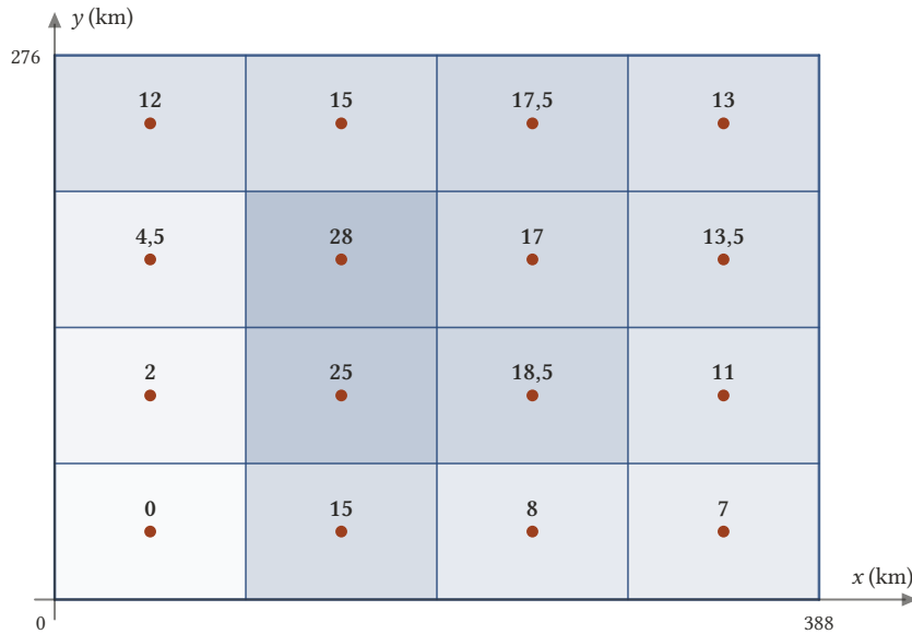
Şekil 1.8: Bölge 4 \times 4 = 16 eş dikdörtgene bölünmüştür; noktalar alt dikdörtgenlerin merkezleri, sayılar bu merkezlerde ölçülen kar kalınlığıdır (cm). Koyu renkli hücrelerde kar daha kalındır.
