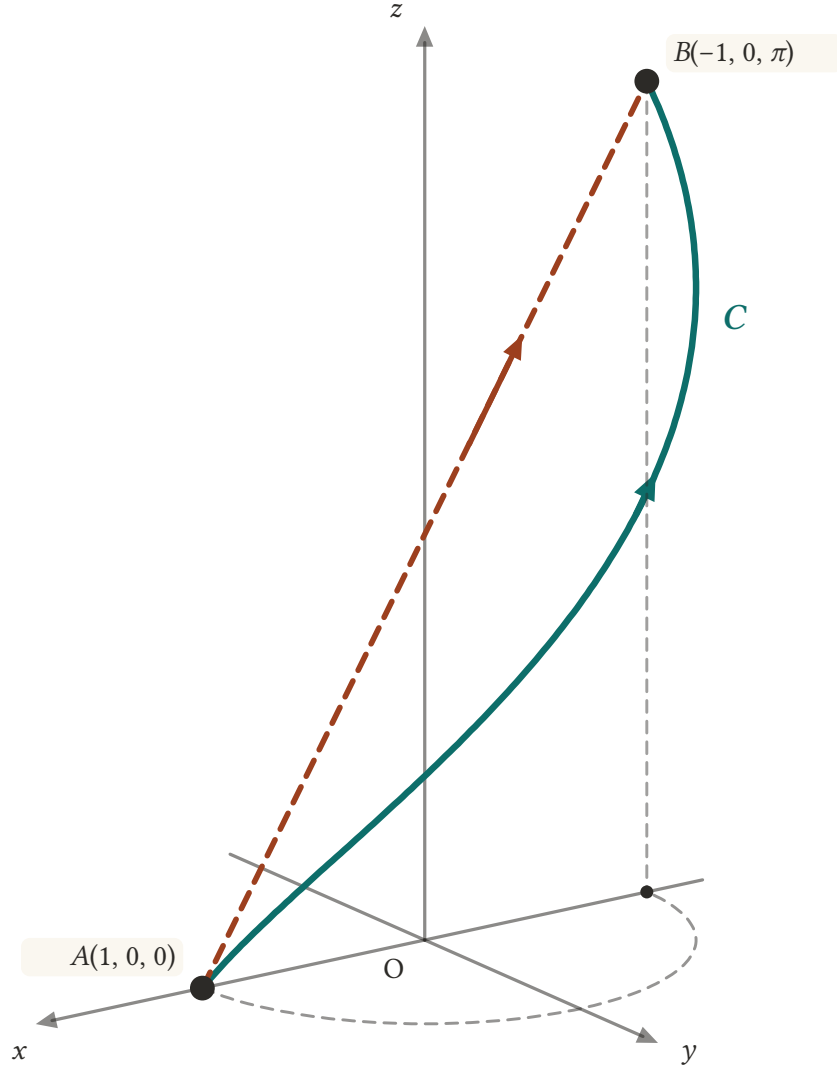
Şekil 12.2: C sarmalı A(1, 0, 0) noktasından B(-1, 0, \pi) noktasına z eksenine çevresinde yarım tur atarak çıkar; zemindeki kesikli yay, sarmalın xy -düzlemindeki izdüşümüdür. Kesikli doğru parçası aynı iki noktayı birleştirir. Temel teoreme göre \nabla f alanının bu iki yol boyunca integralleri eşittir.
