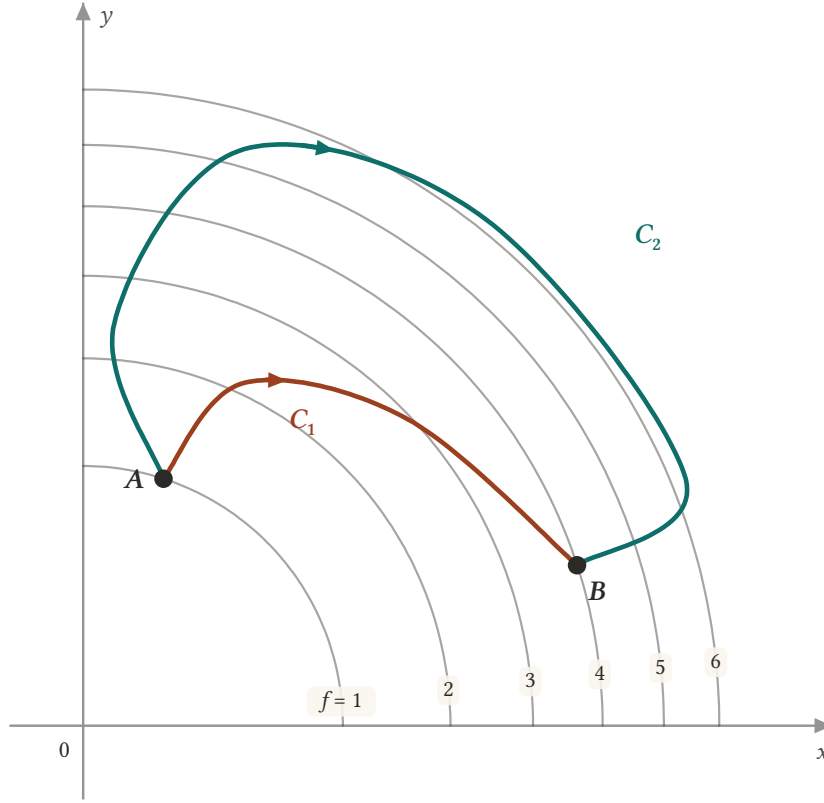
Şekil 12.1: f(x, y) = x^2 + y^2 fonksiyonunun f = 1, 2, \dots, 6 seviye eğrileri ve A'dan B'ye giden iki yol. A noktası f = 1 , B noktası f = 4 eğrisi üzerindedir. C_2 yolu f = 6 eğrisini aşıp geri dönse de iki yol boyunca \int \nabla f \cdot d\mathbf{r} = f(B) - f(A) = 4 - 1 = 3 olur: yükselirken toplanan değerler alçalışken geri verilir.
