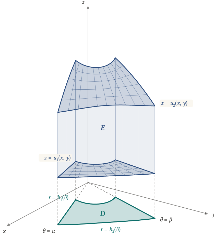
Şekil 7.3: E cismi, xy-düzlemindeki izdüşümü D'nin üstünde, z = u_1(x, y) ile z = u_2(x, y) yüzeyleri arasında kalır. D kutupsal koordinatlarda \alpha \leq \theta \leq \beta , h_1(\theta) \leq r \leq h_2(\theta) ile verilir.
