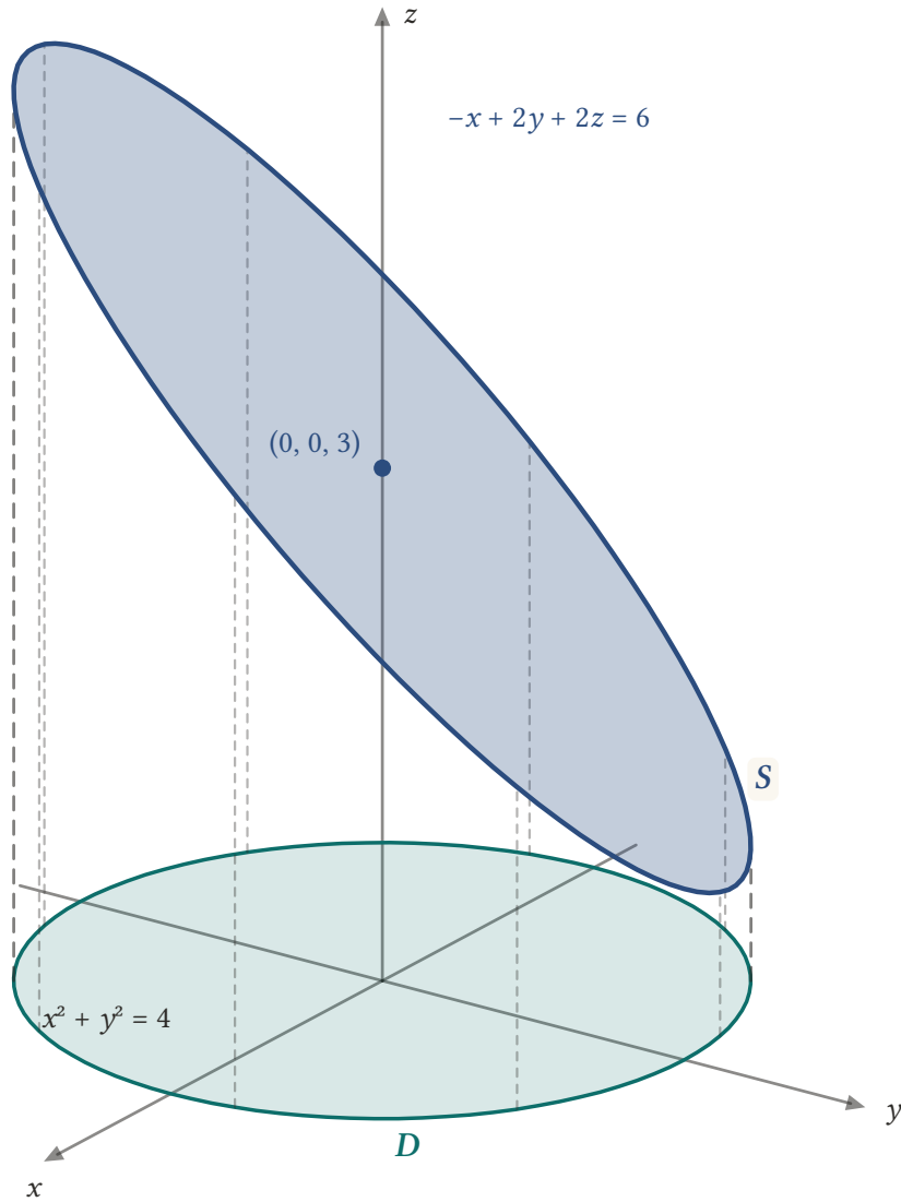
Şekil 5.4: -x + 2y + 2z = 6 düzleminin x^2 + y^2 = 4 silindiri içinde kalan parçası S bir elipstir; gölgesi D ise 2 yarıçaplı dairedir. Eğik düzlem gölgesinden büyüktür: alanı D 'nin alanının 3/2 katıdır.
