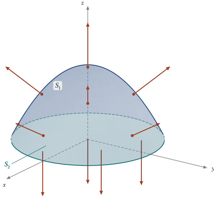
Şekil 16.7: E cisminin sınırı iki parçadır: z = 1 - x^2 - y^2 paraboloidinin z \geq 0 kısmı S_1 ve z = 0 düzlemindeki birim daire S_2 . Dışa doğru yönlendirmede S_1 'in normalleri yukarı, S_2 'ninkiler aşağı bakar.
