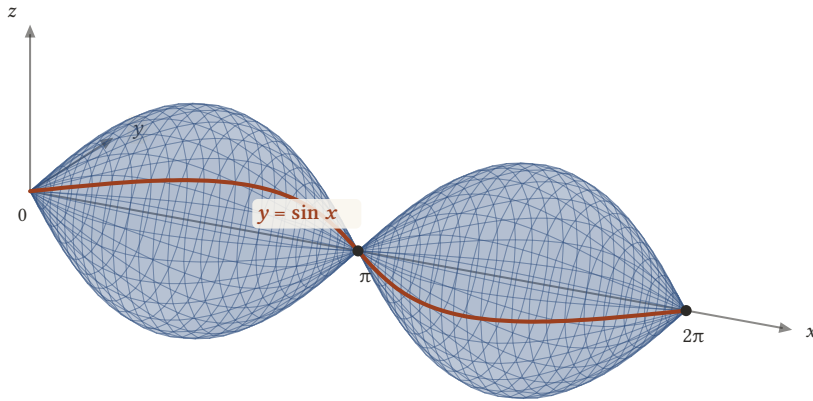
Şekil 15.6: y = \sin x, 0 \leq x \leq 2\pi eğrisinin x ekseninde döndürülmesiyle oluşan yüzey: x = 0, \pi ve 2\pi noktalarında eksene değen iki iğ.
