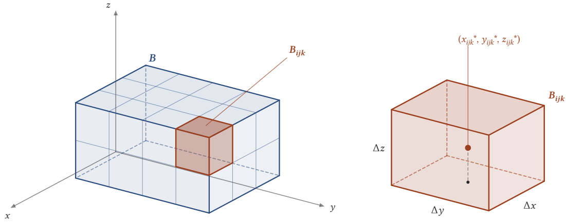
Şekil 6.1: Solda B kutusu l = 3, m = 4, n = 2 için 24 alt kutuya bölünmüştür; turuncu alt kutu B_{ijk} 'dir. Sağda bu alt kutu büyütülmüştür: kenarları \Delta x, \Delta y, \Delta z , hacmi \Delta V = \Delta x \Delta y \Delta z 'dir ve içinden bir örnek nokta seçilir.
