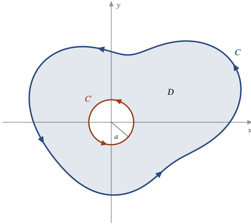
Şekil 13.7: Orijini çevreleyen C eğrisi ve C 'nin içinde kalan, a yarıçaplı C' çemberi. Aradaki D bölgesi orijini içermez; pozitif yönlü sınırı C ile ters yönde dolaşılacak C' çemberinden, yani C \cup (-C') eğrisinden oluşur.
