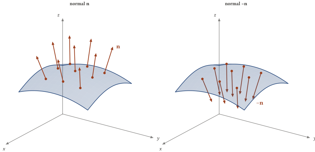
Şekil 16.4: Yönlendirilebilir bir yüzeyin iki yönlendirmesi. Solda her noktada \mathbf{n} , sağda -\mathbf{n} seçilmiştir; iki seçimde de normal yüzey boyunca sürekli değişir. Bu yüzey bir fonksiyon grafiği olduğundan soldaki yukarı, sağdaki aşağı yönlendirmedir.
