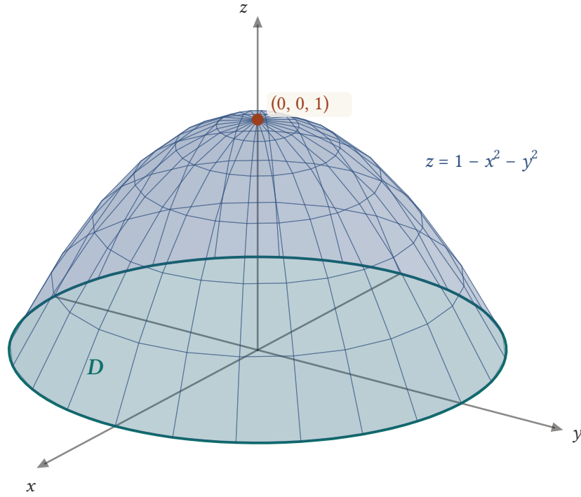
Şekil 3.5: z = 1 - x^2 - y^2 paraboloidi ile xy -düzlemi arasındaki cisim. Paraboloid düzlemi x^2 + y^2 = 1 çemberi boyunca keser; taban D birim diskidir.
