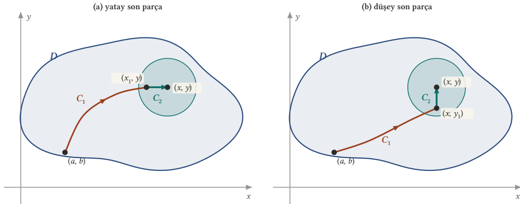
Şekil 12.4: f(x, y) değerini veren yol, (x, y) merkezli ve D 'de kalan diskin içinde bir doğru parçasıyla biter. (a) Yatay C_2 parçasında dy = 0 olduğundan yalnız P katkı verir ve f_x = P bulunur. (b) Düşey parçada dx = 0 'dır ve f_y = Q bulunur.
