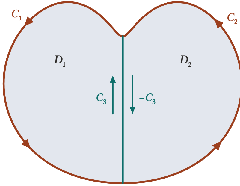
Şekil 13.4: D = D_1 \cup D_2 : ortak kenar C_3 , D_1 'in sınırında yukarı, D_2 'nin sınırında aşağı doğru ( -C_3 ) dolaşılır. Bu iki katkı birbirini götürür ve geriye D 'nin dış sınırı C_1 \cup C_2 kalır.
