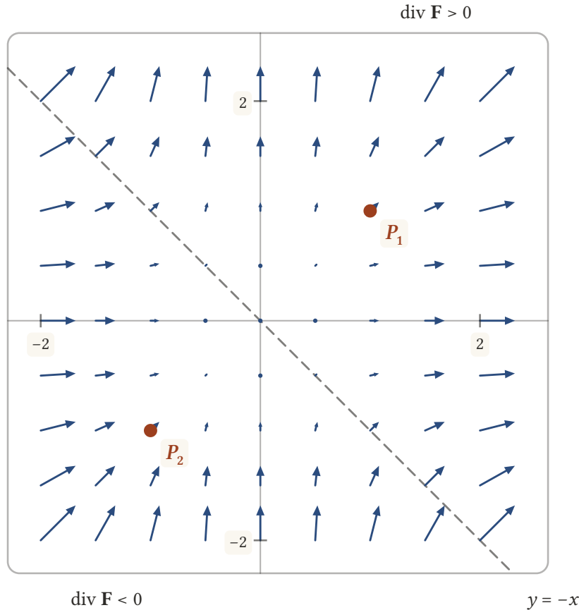
Şekil 18.6: \mathbf{F}(x, y) = x^2 \mathbf{i} + y^2 \mathbf{j} alanı (oklar aynı oranda kısaltıldı). P_1(1, 1) 'in çevresinden çıkan oklar girenlerden uzun, P_2(-1, -1) 'in çevresinde ise kısadır. Kesikli y = -x doğrusunun üstünde \operatorname{div} \mathbf{F} > 0 , altında \operatorname{div} \mathbf{F} < 0 'dır.
