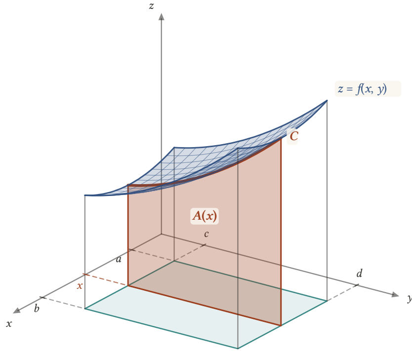
Şekil 1.5: Cismin x noktasından geçen ve x eksenine dik düzlemle kesiti (turuncu), c \leq y \leq d aralığında C: z = f(x, y) eğrisinin altında kalan bölgedir. Alanı A(x) = \int_c^d f(x, y) dy olduğundan hacim \int_a^b A(x) dx ardışık integrale eşittir.
