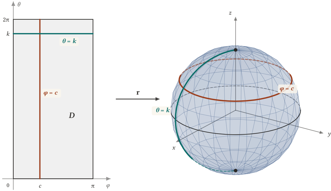
Şekil 15.4: Küre parametrelemesi \mathbf{r}(\phi, \theta) , [0, \pi] \times [0, 2\pi] dikdörtgenini küreye gönderir. Düşey \phi = c doğrusu bir enlem çemberine, yatay \theta = k doğrusu kutupları birleştiren bir meridyene gider.
