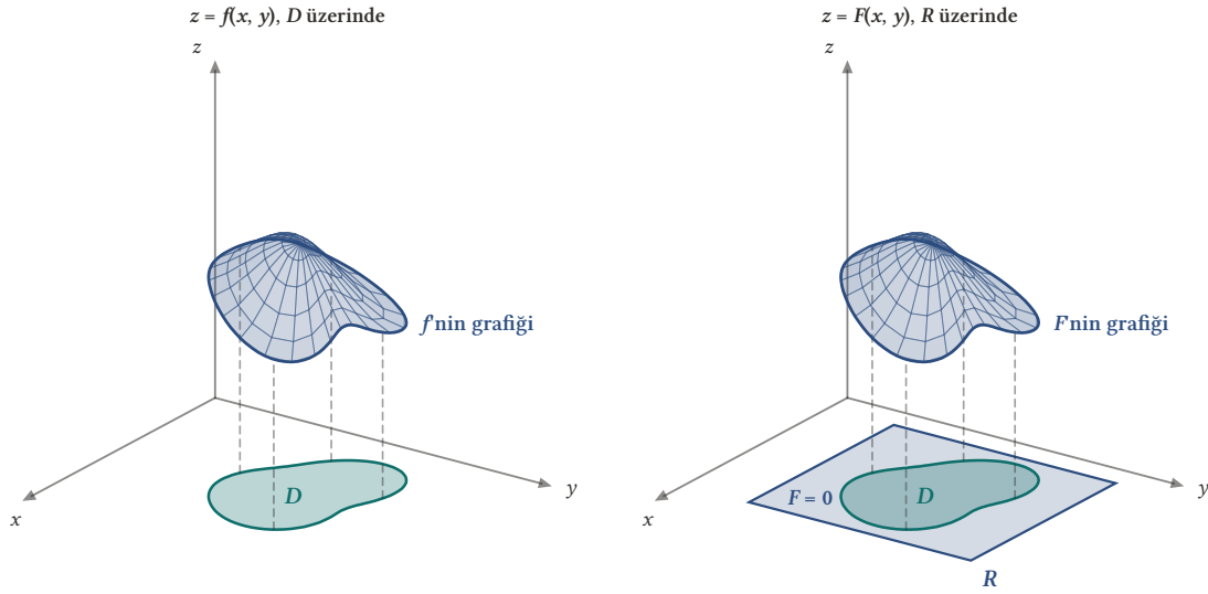
Şekil 2.1: Solda f 'nin D üzerindeki grafiği. Sağda D 'yi içeren R dikdörtgeni ve F 'nin grafiği: D üzerinde f ile aynı yüzey, R 'nin geri kalanında taban düzlemi ( F = 0 ). İki grafiğin altında kalan hacim aynıdır.
