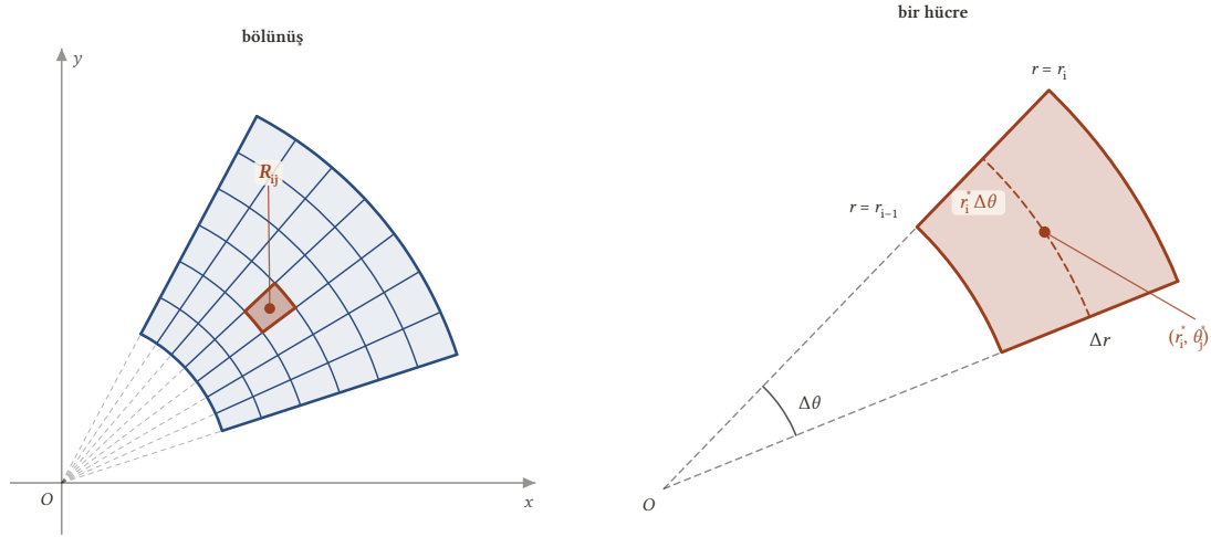
Şekil 3.3: Sol: r = r_i çemberleri ve \theta = \theta_j ışınları R 'yi küçük kutupsal dikdörtgenlere böler. Sağ: bir R_{ij} hücresi. Işın yönündeki kenarı \Delta r , merkezinden geçen yayın uzunluğu r_i^* \Delta \theta ve alanı tam olarak \Delta A_{ij} = r_i^* \Delta r \Delta \theta dir.
