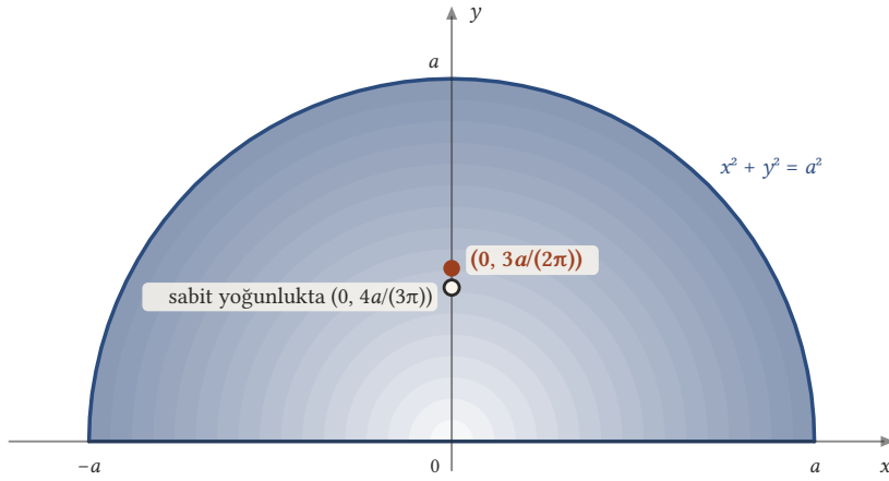
Şekil 4.4: Yoğunluk merkeze uzaklıkla orantılı olduğunda (koyu renk büyük yoğunluk) kütle merkezi (0, 3a/(2\pi)) \approx (0; 0,477a) noktasıdır. Yoğunluk sabit olsaydı kütle merkezi (0, 4a/(3\pi)) \approx (0; 0,424a) olurdu (içi boş nokta): ağırlık dışa doğru arttığı için kütle merkezi yukarı kayar.
