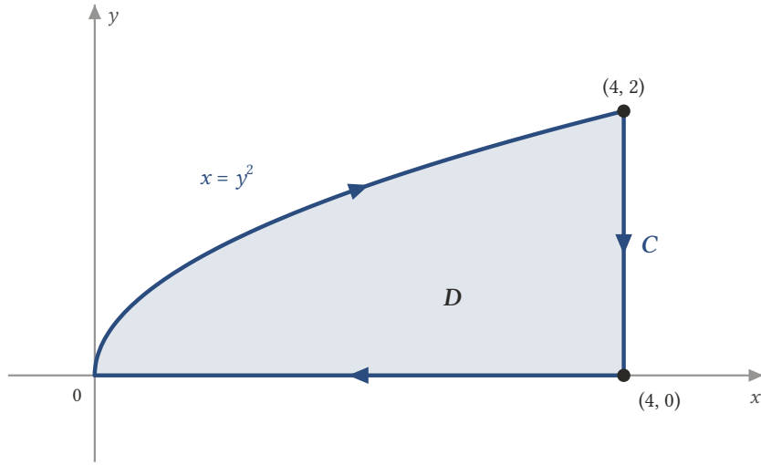
Şekil 13.8: C eğrisi önce x = y^2 parabolü boyunca (0, 0) 'dan (4, 2) 'ye, sonra düşey doğru parçasıyla (4, 0) 'a, oradan da x eksenini boyunca orijine döner. Bu dolaşımda D bölgesi sağda kalır: C saat yönünde, yani negatif yönlüdür.
