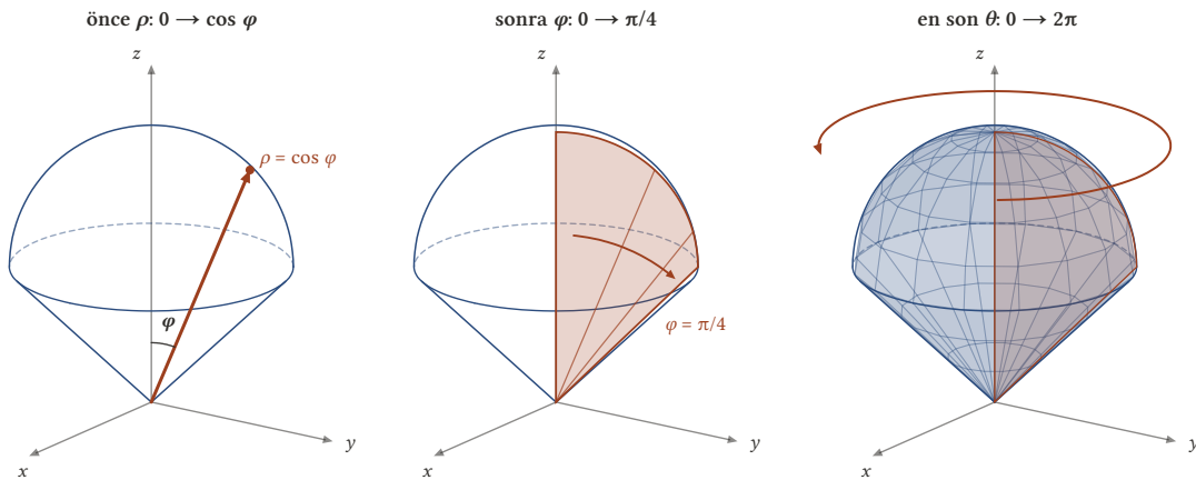
Şekil 8.6: Ardışık integralin cismi taraması. Önce \phi ve \theta sabitken \rho , 0'dan küre üzerindeki \cos \phi değerine gider ve bir doğru parçası çizer. Sonra \theta sabitken \phi , 0'dan \pi/4 'e gider ve bu parçalar bir yarı düzlem dilimini doldurur. En son \theta , 0'dan 2\pi 'ye gider ve dilim z ekseninde dönerek cismin tamamını tarar.
