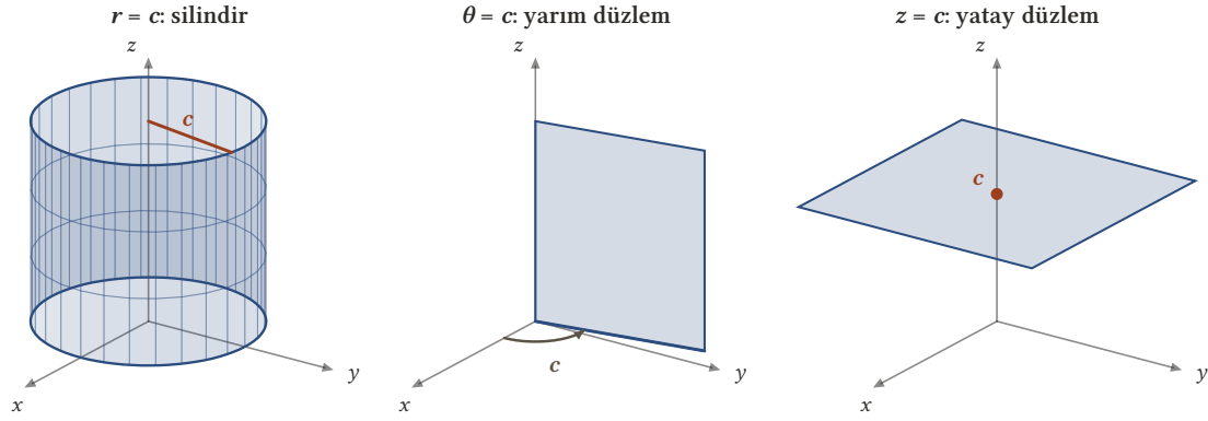
Şekil 7.2: Silindirik koordinatlarda bir koordinatı sabitlemek: r = c eksen z eksenine olan dairesel bir silindir, \theta = c kenarı z eksenine olan düşey bir yarım düzlem, z = c yatay bir düzlemdir. Her yüzeyin yalnız bir parçası çizilmiştir.
