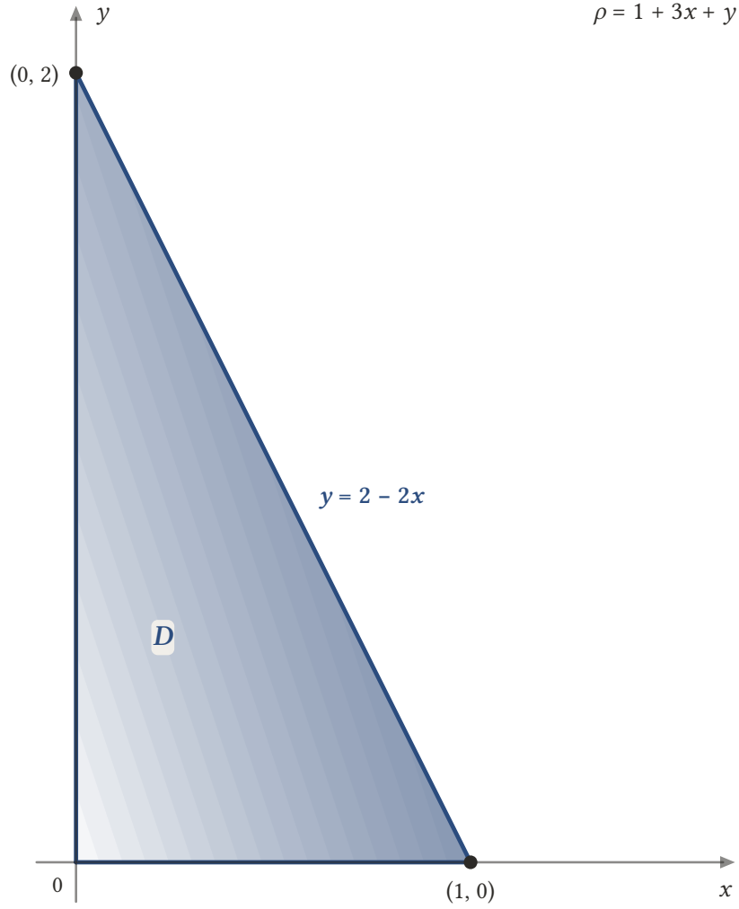
Şekil 4.3: Köşeleri (0, 0) , (1, 0) ve (0, 2) olan üçgen levha. Renk koyulaştıkça yoğunluk \rho(x, y) = 1 + 3x + y büyür: en hafif köşe orijin ( \rho = 1 ), en ağır köşeler (1, 0) ve (0, 2) 'dir ( \rho = 4 ve 3 ).
