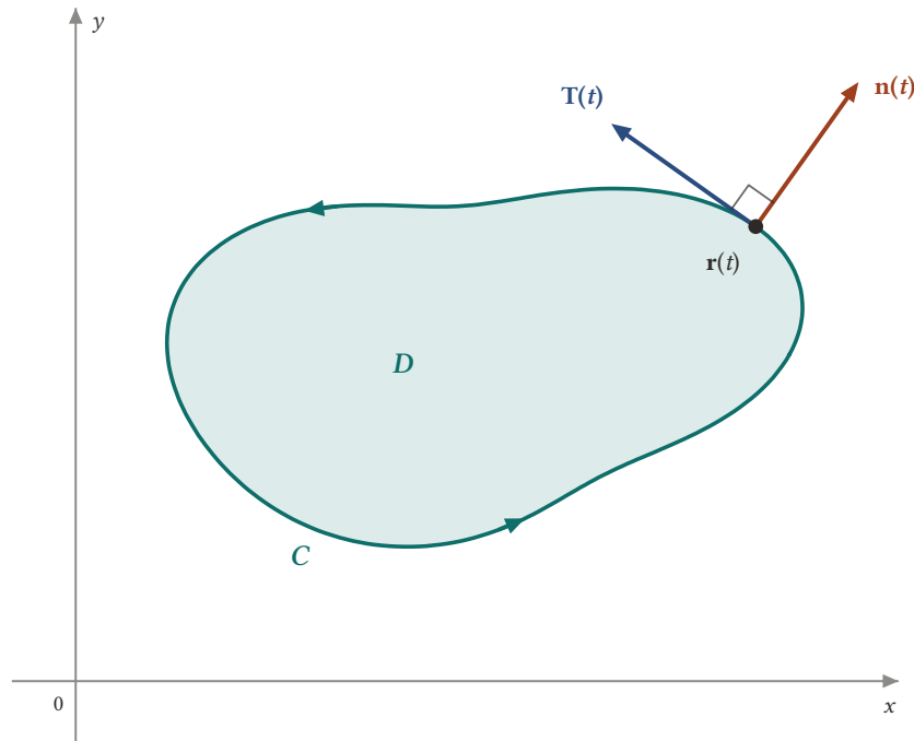
Şekil 14.5: C pozitif yönde ( D solda kalacak biçimde) dolaşılır. \mathbf{T}(t) birim teğet vektördür; \mathbf{n}(t) , \mathbf{T}(t) 'nin saat yönünde 90^\circ döndürülmesiyle elde edilir ve D 'nin dışını gösterir.
