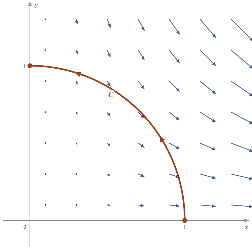
Şekil 11.6: \mathbf{F}(x, y) = x^2 \mathbf{i} - xy \mathbf{j} kuvvet alanı ve (1, 0) noktasından (0, 1) noktasına giden çeyrek çember C . Oklar eğri boyunca hareketle geniş açı yapar, yani alan hareketi engeller; bu yüzden yapılan iş negatiftir.
