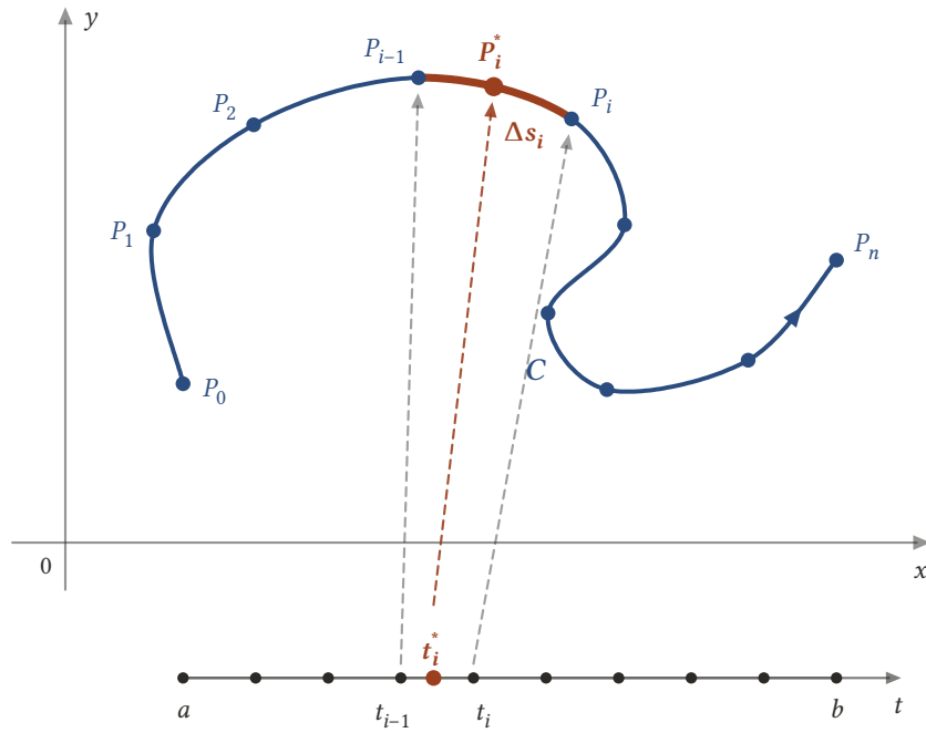
Şekil 11.1: [a, b] parametre aralığı n eşit parçaya bölününce C eğrisi de P_0, P_1, \dots, P_n noktalarıyla n alt yaya bölünür; P_i = \mathbf{r}(t_i) olur. i -inci alt yayın uzunluğu \Delta s_i , üzerinden seçilen nokta P_i^* = \mathbf{r}(t_i^*) noktasıdır.
