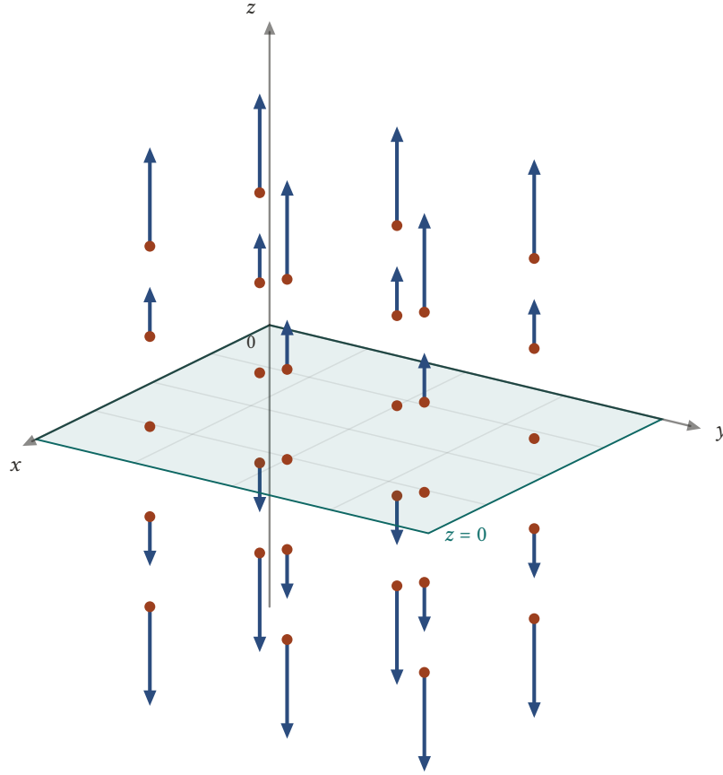
Şekil 10.4: F(x, y, z) = z \mathbf{k} . Bütün oklar düşeydir: xy -düzleminin üstünde yukarı, altında aşağı bakar ve düzlemden uzaklaştıkça uzar. Düzlemin üzerindeki noktalarda vektör sıfırdır.
