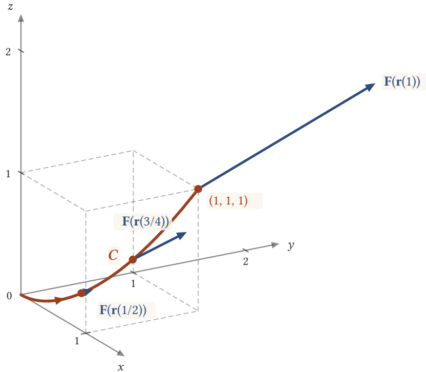
Şekil 11.7: x = t , y = t^2 , z = t^3 ( 0 \leq t \leq 1 ) kübik eğrisi ve t = 1/2, 3/4, 1 noktalarında \mathbf{F} = xy \mathbf{i} + yz \mathbf{j} + zx \mathbf{k} vektörleri (gerçek uzunluklarıyla). Kesikli çizgiler birim küpün kenarlarıdır.
