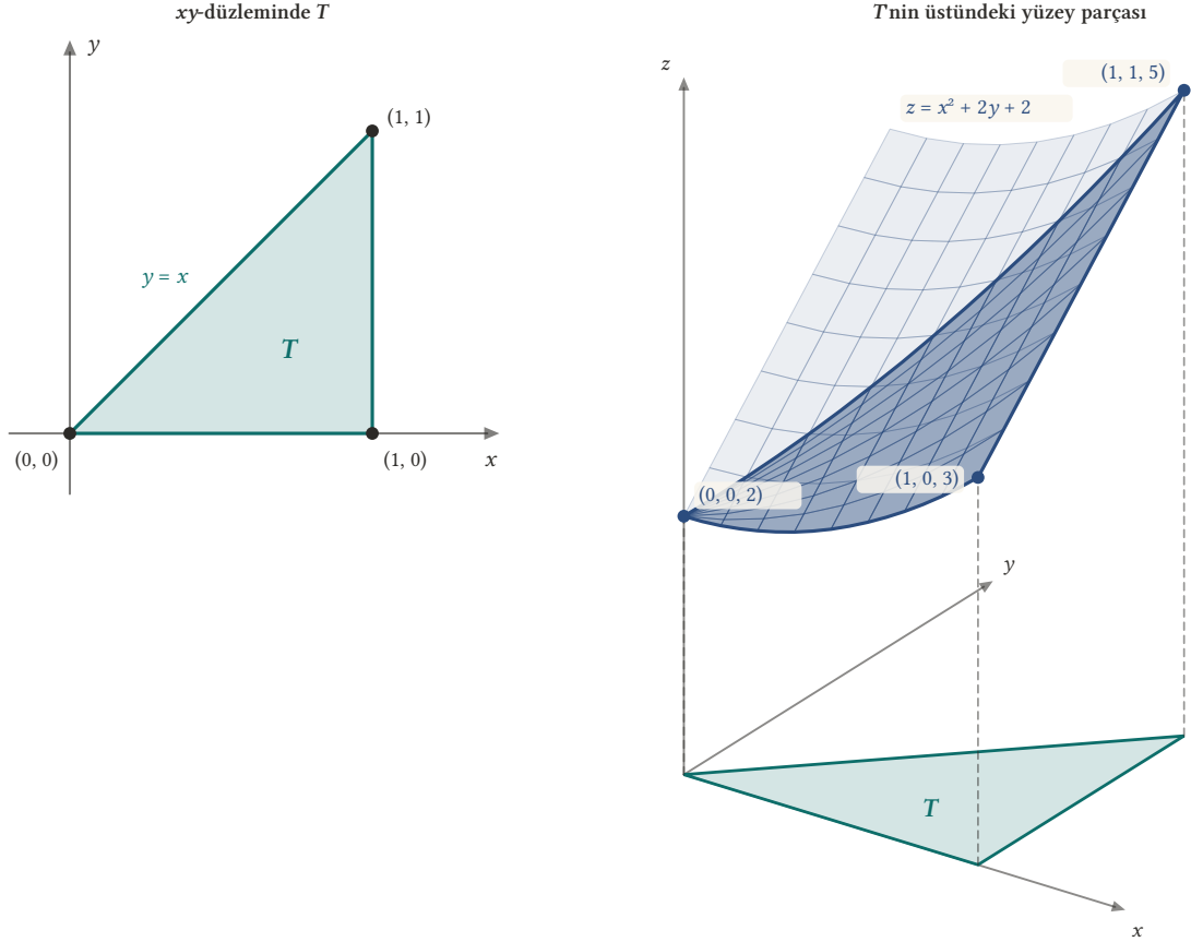
Şekil 5.5: Solda (0, 0) , (1, 0) , (1, 1) köşeli T üçgeni: 0 \leq x \leq 1 , 0 \leq y \leq x . Sağda z = x^2 + 2y + 2 yüzeyinin T üstündeki parçası (koyu) ve birim kare üstündeki devamı (açık). Sağ panelde düşey ölçek küçültülmüştür.
