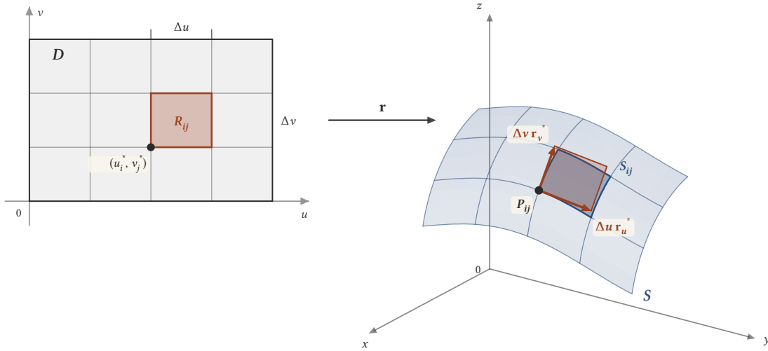
Şekil 15.8: D dikdörtgeni \Delta u \times \Delta v boyutlu alt dikdörtgenlere bölünür. R_{ij} 'nin görüntüsü S_{ij} yamasıdır (koyu). Yama, P_{ij} köşesinden çıkan \Delta u \mathbf{r}_u^* ve \Delta v \mathbf{r}_v^* vektörlerinin gerdiği paralelkenarla (turuncu) yaklaşık olarak aynı alana sahiptir.
