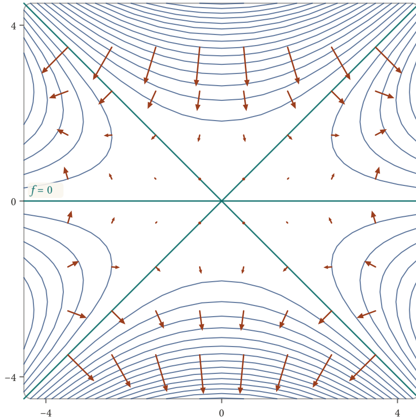
Şekil 10.7: f(x, y) = x^2y - y^3 fonksiyonunun seviye eğrileri (mavi; ardışık seviyeler arasındaki fark 6'dır, f = 0 seviyesi üç doğrudur) ve gradyan vektör alanı (turuncu, oklar aynı oranda kısaltılmış). Oklar seviye eğrilerine diktir; eğrilerin sık olduğu yerde uzun, seyrek olduğu yerde kısadır.
