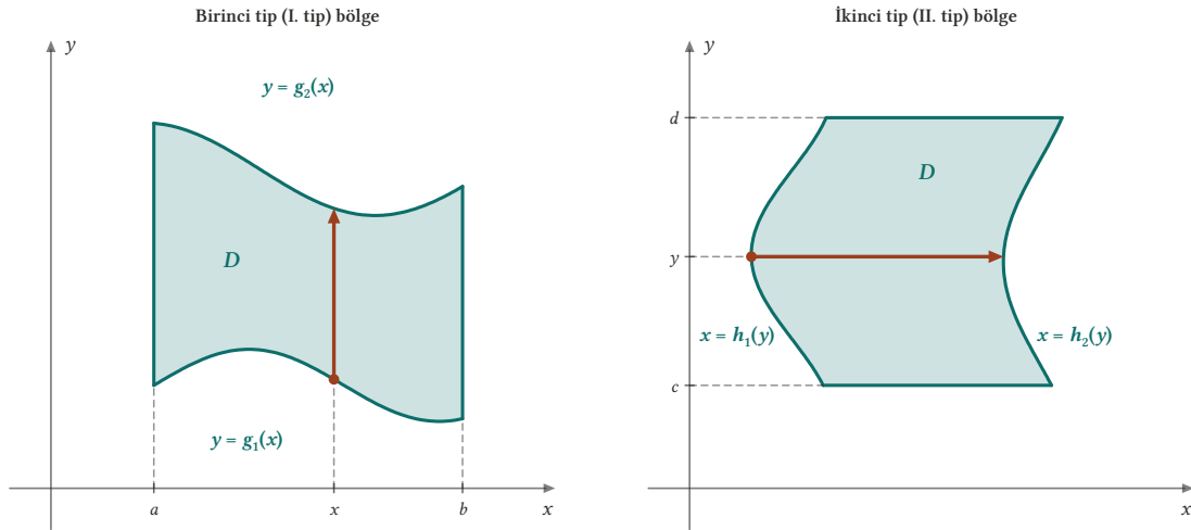
Şekil 2.2: Solda I. tip bir bölge: alt ve üst kenarı x 'in fonksiyonlarının grafikleridir. Düşey ok y = g_1(x) eğrisinden girip y = g_2(x) eğrisinden çıkar ve iç integralin sınırlarını verir. Sağda II. tip bir bölge: sol ve sağ kenarı y 'nin fonksiyonlarıdır; yatay ok x = h_1(y) eğrisinden x = h_2(y) eğrisine gider.
