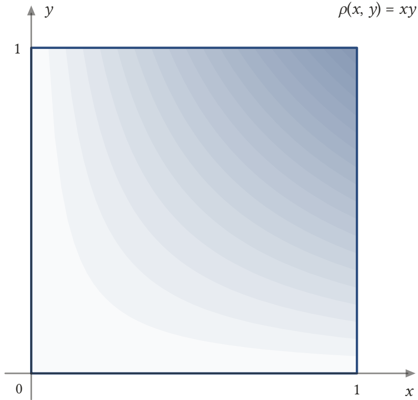
Şekil 4.8: Yoğunluğu \rho(x, y) = xy olan kare levha; renk koyulaştıkça yoğunluk büyür. Sol ve alt kenarlarda yoğunluk 0'dır.
