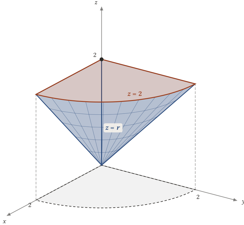
Şekil 7.8: 0 \leq \theta \leq \pi/2 , r \leq z \leq 2 cismi: z = r konisinin üstünde, z = 2 düzleminin altında kalan dolu koninin x \geq 0 , y \geq 0 tarafındaki çeyreği.
