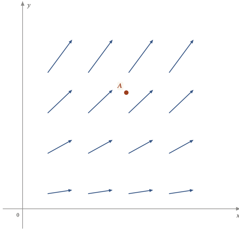
Şekil 14.6: Alanın xy -düzlemindeki kısmı. Alan z 'den bağımsızdır ve z -bileşeni 0'dır.
