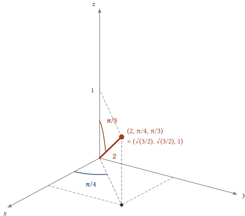
Şekil 8.2: Küresel koordinatları (2, \pi/4, \pi/3) olan nokta: orijinden 2 birim uzakta, z eksenine \pi/3 açı yapan ve izdüşümü x eksenine \pi/4 açı yapan doğrultuda. Dik koordinatları (\sqrt{3/2}, \sqrt{3/2}, 1) 'dir.
