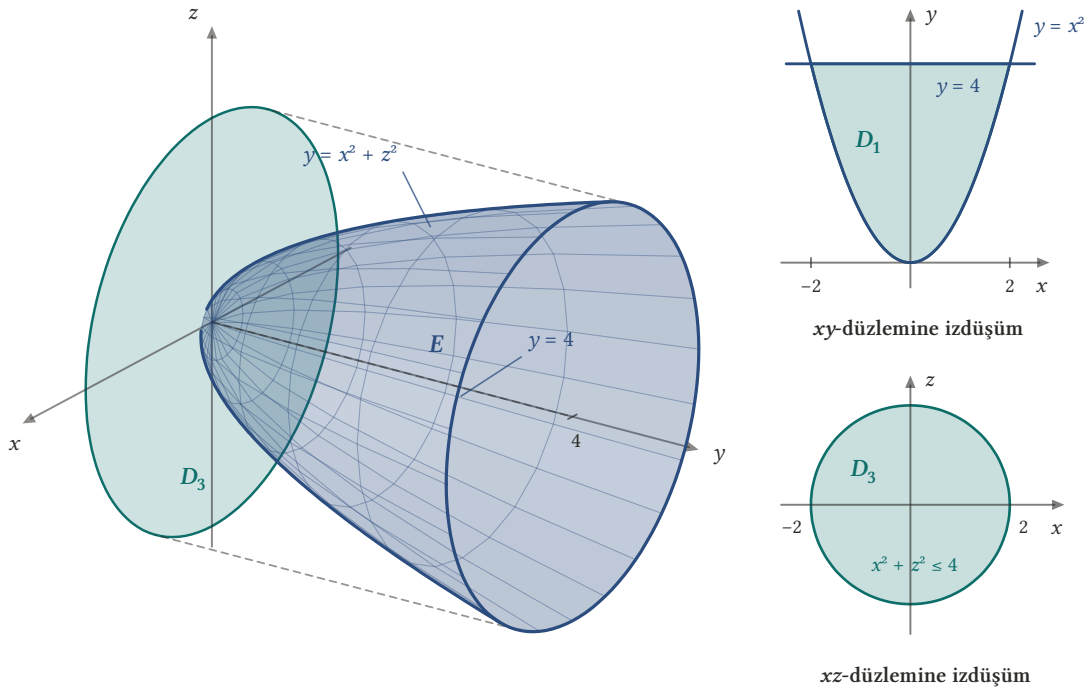
Şekil 6.5: Solda y = x^2 + z^2 paraboloidi ile y = 4 düzlemi arasındaki E cismi ve onun xz -düzlemine izdüşümü D_3 . Sağ üstte E 'nin xy -düzlemine izdüşümü D_1 ( x^2 \leq y \leq 4 ), sağ altta D_3 diski ( x^2 + z^2 \leq 4 ).
