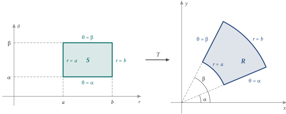
Şekil 9.5: x = r \cos \theta , y = r \sin \theta dönüşümü r\theta -düzlemindeki [a, b] \times [\alpha, \beta] dikdörtgenini xy -düzlemindeki kutupsal dikdörtgene götürür: r = \text{sabit} doğruları çember yaylarına, \theta = \text{sabit} doğruları orijinden çıkan ışınlara gider.
