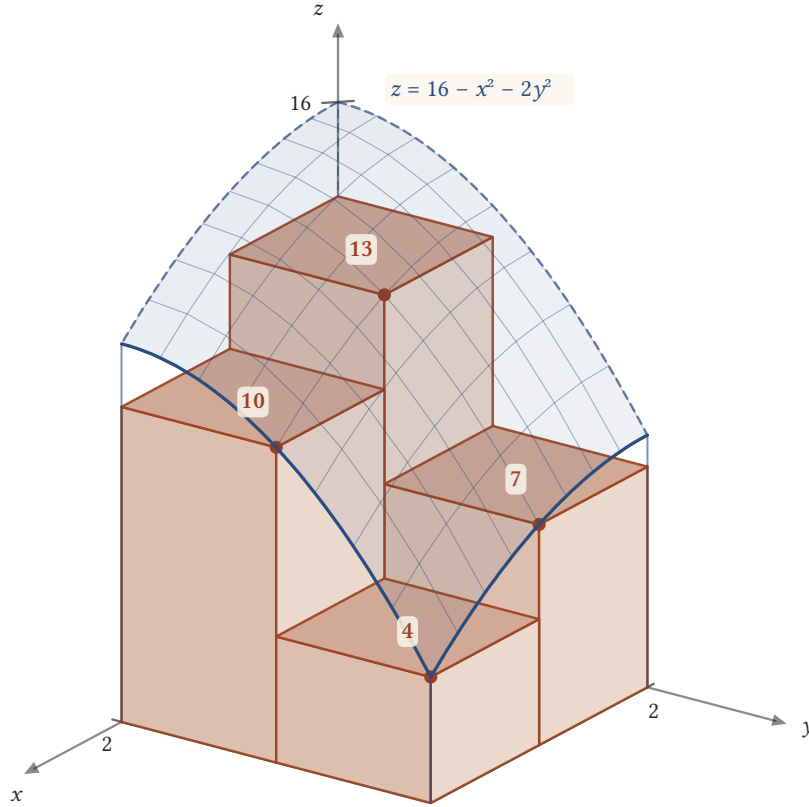
Şekil 1.3: z = 16 - x^2 - 2y^2 paraboloidinin altına dikilen dört kutu (düşey eksen küçültülmüş ölçekte). Yükseklikler karelerin sağ üst köşelerindeki değerlerdir: 13, 7, 10 ve 4. Kutuların toplam hacmi 34'tür.
