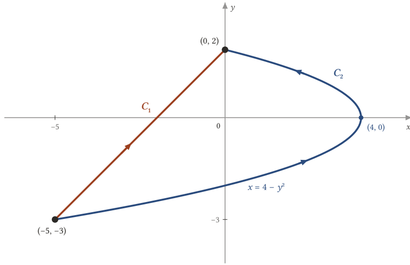
Şekil 11.4: (-5, -3) noktasından (0, 2) noktasına giden iki yol: C_1 doğru parçası ve C_2 : x = 4 - y^2 parabol yayı. Uç noktalar aynı olduğu hâlde \int y^2 dx + x dy integrali C_1 boyunca -5/6 , C_2 boyunca 245/6 olur.
