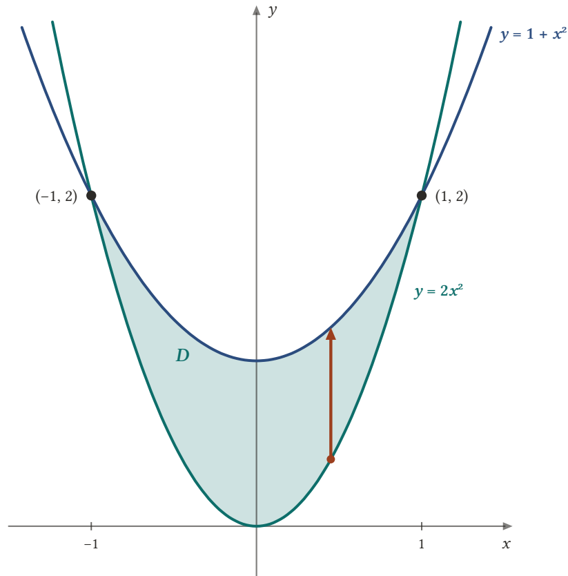
Şekil 2.3: y = 2x^2 ve y = 1 + x^2 parabolleri (-1, 2) ve (1, 2) noktalarında kesişir. Aradaki D bölgesi I. tiptir: her düşey ok alttaki y = 2x^2 parabolünden girer, üstteki y = 1 + x^2 parabolünden çıkar.
