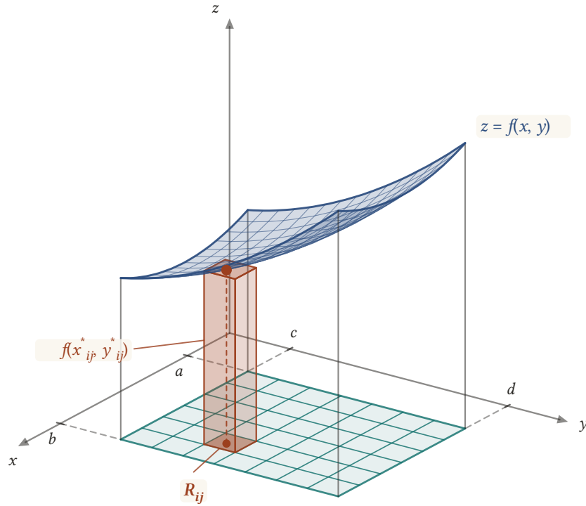
Şekil 1.2: Tabanı R_{ij} , yüksekliği f(x_{ij}^*, y_{ij}^*) olan kutu (turuncu), cismin R_{ij} üzerindeki ince parçasının yerini tutar; hacmi f(x_{ij}^*, y_{ij}^*) \Delta A 'dır. Bütün alt dikdörtgenlerdeki kutuların hacimleri toplamı iki katlı Riemann toplamıdır.
