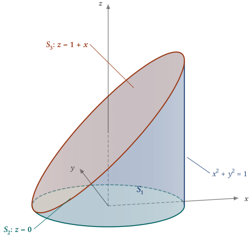
Şekil 16.2: S yüzeyi üç parçadan oluşur: x^2 + y^2 = 1 silindirin yan yüzü S_1 , z = 0 düzlemindeki birim daire S_2 ve z = 1 + x düzleminin bu dairenin üstündeki parçası S_3 . Tavan, x = 1 'de 2 yüksekliğine çıkar ve (-1, 0, 0) noktasında tabana değer.
