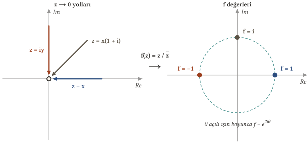
Şekil 7.2: f(z) = z/\bar{z} her ışıın üzerinde sabittir ama ışıından ışıına değişir: reel ekseninde 1, sanal ekseninde -1, köşegende i ; genel olarak \theta açılı ışıında e^{2i\theta} . Değerler birim çember üzerinde dağıldığından z \rightarrow 0 için tek bir limit yoktur.
