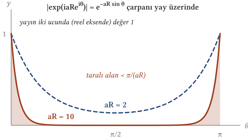
Şekil 17.2: C_R üzerinde e^{iaz} çarpanının modülü e^{-aR \sin \theta} 'dir; yayın uçlarında 1'e eşittir ama aR büyüdükçe yayın iç kısmında hızla sıfıra çöker. Bu yüzden eğrinin altındaki alan \pi/(aR) ile sınırlıdır ve yay integrallerinde ML kestirimindeki R çarpanı yok olur — Jordan lemmasının kazancı budur.
