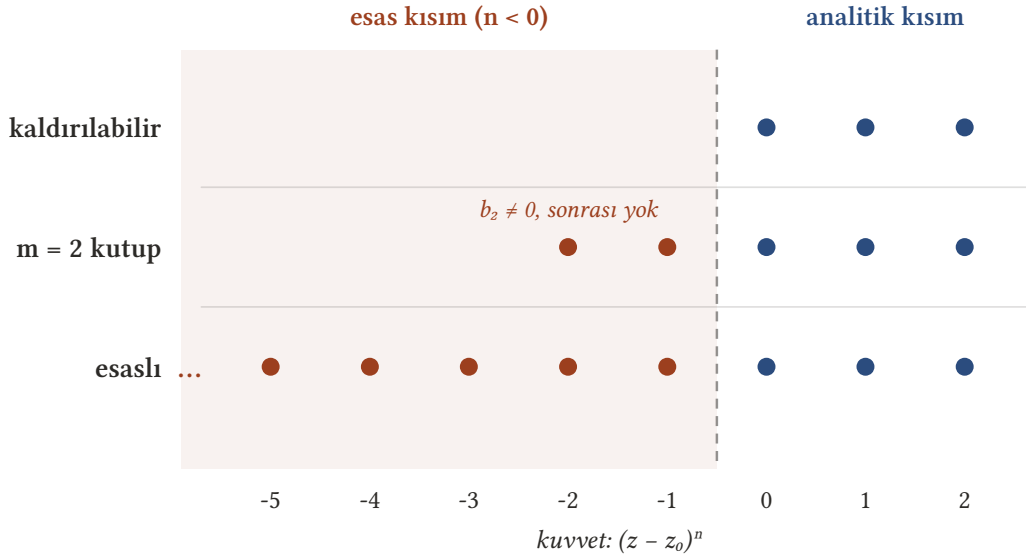
Şekil 13.1: Üç tekillik tipi, tek bakışta: her satır bir Laurent açılımıdır, dolu noktalar sıfırdan farklı katsayıları gösterir. Fark yalnızca esas kısımdaki (negatif kuvvetli) terim sayıdadır: hiç yoksa kaldırılabilir, sonluysa kutup, sonsuzsa esaslı tekil nokta.
