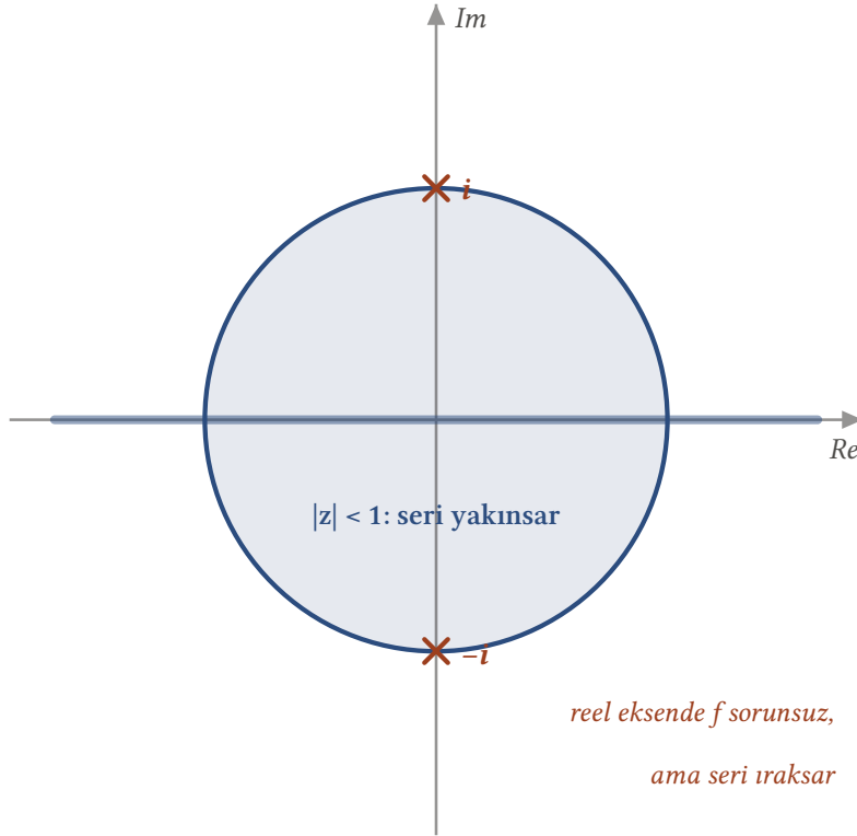
Şekil 9.2: 1/(1+z^2) reel eksenin her noktasında düzgün ve sonsuz kez türevlenebilirdir; yine de Maclaurin serisi yalnız |z| < 1 'de yakınsar. Engel reel ekseninde değil, sanal eksenindedir: tekil noktalar \pm i merkeze 1 uzaklıktadır ve yakınsaklık çemberi onlara değince büyümesi durur.
