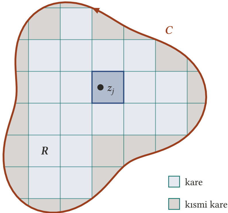
Şekil 1.1: R bölgesi ( C ile içi) eksenlere paralel bir ızgarayla örtülür: tamamen C 'nin içinde kalan hücreler kare , C 'nin kestiği hücrelerin R 'de kalan parçaları kısmi kare dir. Her alt bölgede lemmanın sabit z_j noktası seçilir; kısmi karenin sınırı, kare kenarlarının parçalarının yanı sıra C 'nin yaylarını da içerir.
