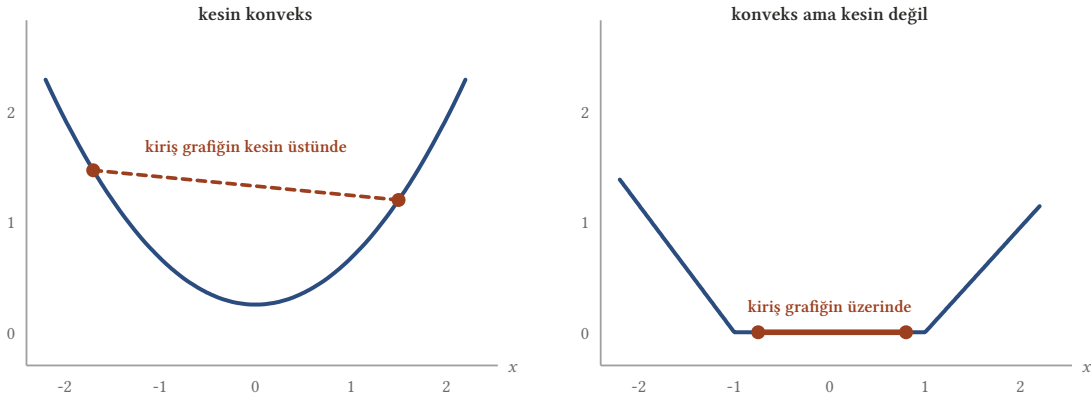
Şekil 11.6: Kesin konvekslikte uç noktalar dışında kiriş ile grafik hiç değmez. Sağdaki fonksiyon konvektir ama düz parçası üzerinde kiriş grafiğin tam üstüne oturur; eşitsizlik eşitliğe dönüştüğünden kesin konveks değildir. Kesin konvekslik, bir eniyileme probleminin çözümünün tek olduğunu garanti etmek için istenen ek koşuldur.
