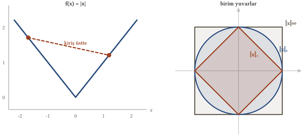
Şekil 11.5: Norm fonksiyonu üçgen eşitsizliği ile homojenlik sayesinde konvektir: \|\lambda x_1 + (1-\lambda)x_2\| \leq \lambda\|x_1\| + (1-\lambda)\|x_2\| . Bunun geometrik karşılığı, her normun birim yuvarının konveks olmasıdır — birim yuvar, normun 1 seviye kümesidir.
