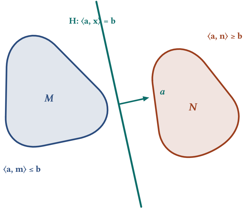
Şekil 10.3: Bir H hiperdüzlemi, M 'nin bütün noktalarını \langle a, x \rangle \leq b , N 'nin bütün noktalarını \langle a, x \rangle \geq b yarı uzayında bırakıyorsa iki kümeyi ayırır . Ayırma, iki kümeyi tek bir lineer eşitsizlikle birbirinden ayırt edebilmek demektir; konveks analizin dualite kuramı bu fikrin üzerine kurulur.
