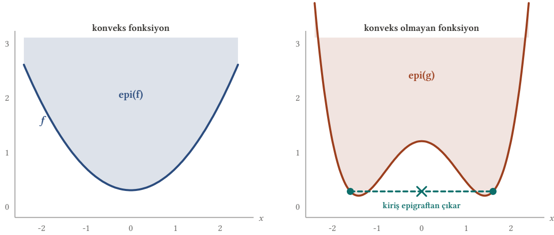
Şekil 11.3: Bir fonksiyonun grafiküstü (epigraf) kümesi, grafiğinin üzerinde kalan noktalardan oluşur. Konveks fonksiyon tanımı gereği epigrafı konveks olan fonksiyondur. Sağdaki fonksiyonda epigrafın iki noktasını birleştiren kiriş kümenin dışına düşer; bu, kirişin grafiğin altına inmesiyle aynı şeydir.
