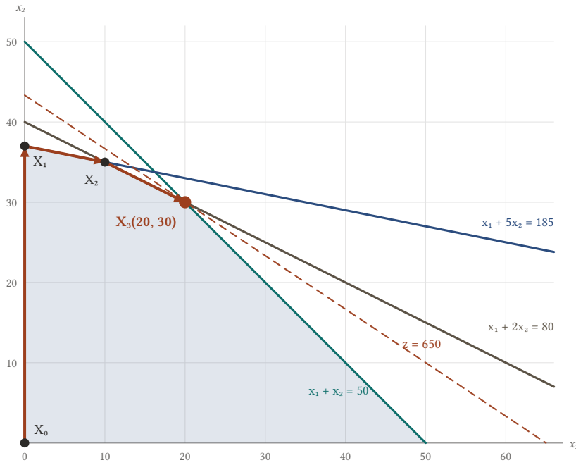
Şekil 11.3: Beş kısıtlı maksimum probleminin uygun bölgesi. Simpleks yöntem X_0(0, 0) köşesinden ( z = 0 ) başlar; x_2 baza girince X_1(0, 37) köşesine ( z = 555 ), x_1 baza girince X_2(10, 35) köşesine ( z = 625 ), x_6 baza girince X_3(20, 30) köşesine ( z = 650 ) geçer. Kesikli doğru z = 650 seviye doğrusudur. Şekilde yalnız bölgeyi sınırlayan kısıt doğruları çizildi: 2x_1 + x_2 \leq 110 ve 5x_1 + 6x_2 \leq 300 kısıtları bölgenin her noktasında kendiliğinden sağlanır; optimal çözümde aylak değişkenleri x_4 = 40 ve x_7 = 20 'dir.
