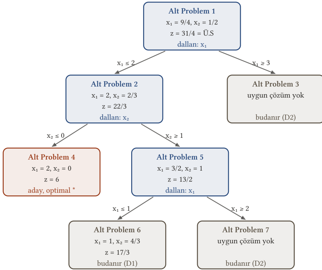
Şekil 13.10: Ek örneğin dal-sınır ağacı. Alt Problem 3 ve 7 uygun olmadığı için, Alt Problem 6 da z = 17/3 değeri mevcut aday değeri 6'yı geçemediği için budanır. Tek aday Alt Problem 4'tür: x_1 = 2, x_2 = 0, z = 6 .
