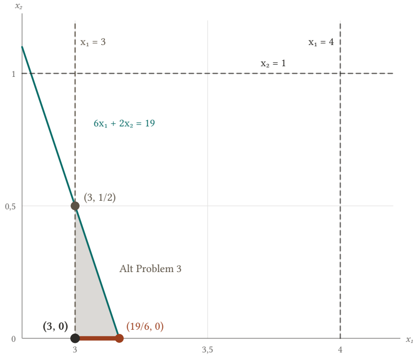
Şekil 14.5: Alt Problem 3'ün uygun bölgesi (3, 0) , (19/6, 0) , (3, 1/2) köşeli küçük üçgendir. x_2 \geq 1 yarı düzlemi bu üçgene değmez (Alt Problem 5 uygun değildir); x_2 \leq 0 ile kesişimi kalın çizilen doğru parçasıdır (Alt Problem 4). Bu parçanın x_1 \leq 3 ile kesişimi yalnız (3, 0) noktasıdır (Alt Problem 6), x_1 \geq 4 ile kesişimi boştur (Alt Problem 7).
