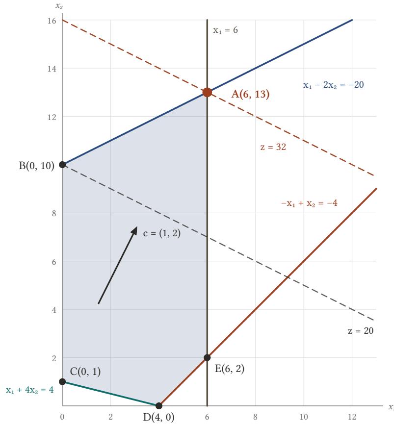
Şekil 3.5: Uygun bölge ABCDE beşgenidir. Kesikli doğrular z = x_1 + 2x_2 amaç fonksiyonunun z = 20 ve z = 32 seviye doğrularıdır; ok gradyan yönünü gösterir. Seviye doğrusu gradyan yönünde kaydırıldığında bölgeden en son A(6, 13) köşesinde ayrılır: \max z = 32 .
