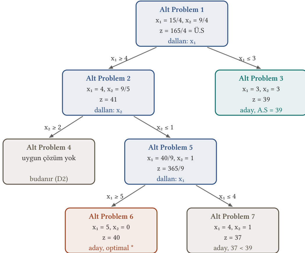
Şekil 13.7: Örneğin dal-sınır ağacı. Her kutuda alt problemin rahatlatılmış optimumu, z değeri ve verilen karar yazılıdır; oklarda eklenen kısıt durur. Alt Problem 4 uygun olmadığı, Alt Problem 3, 6 ve 7 tam sayılı çözüm verdiği için dallanmaz. En iyi aday Alt Problem 6'dır: x_1 = 5, x_2 = 0, z = 40 .
