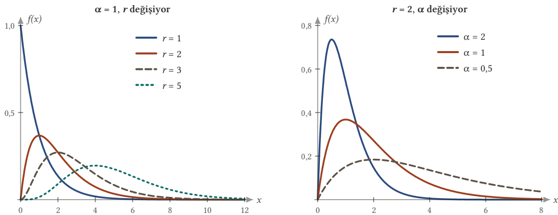
Şekil 4.3: \text{Gamma}(r, \alpha) yoğunlukları. Solda \alpha = 1 iken r büyüdükçe tepe sağa kayar ve eğri yayvanlaşır; r = 1 üstel yoğunluktur. Sağda r = 2 iken \alpha büyüdükçe yoğunluk sıfıra doğru sıkışır: \alpha bir ölçek (oran) parametresidir.
