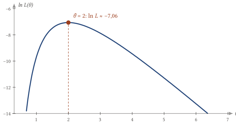
Şekil 10.5: N(\theta, \theta) modelinde 0, 2, 2, 4 örnekleme için log-olabilirlik. Eğrinin tek bir tepesi vardır ve bu tepe \theta^2 + \theta = 6 denkleminin pozitif kökü \theta = 2 'dedir.
