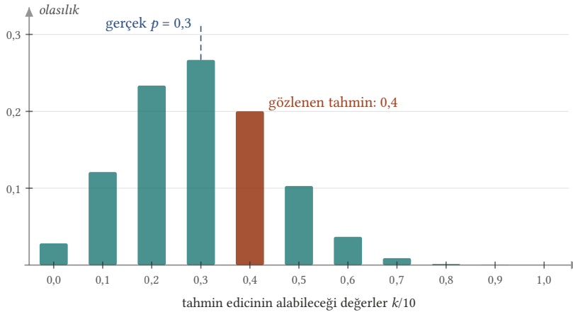
Şekil 9.1: p = 0,3 iken 10 atışlık örneklemde hesaplanan \hat{p} = \bar{X} tahmin edicisinin olasılık fonksiyonu. Tahmin edici 0; 0,1; ...; 1 değerlerinden birini rastgele alır; bu örneklemde gözlenen değer 0,4'tür.
