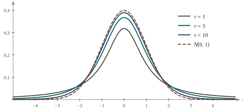
Şekil 12.3: Serbestlik derecesi v = 1, 3 ve 10 olan t yoğunlukları ile standart normal yoğunluk (kesikli). Hepsisi 0 'a göre simetriktir. t eğrilerinin tepesi daha alçak, kuyrukları daha kalındır; v büyüdükçe eğri standart normale yaklaşır.
