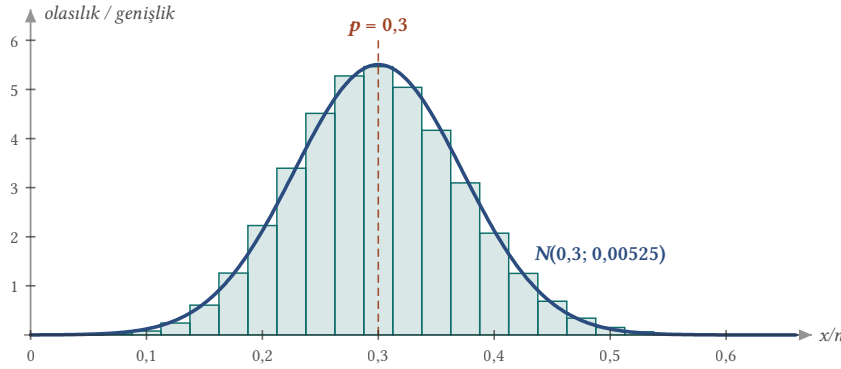
Şekil 15.1: n = 40 ve p = 0,3 iken \hat{p} = X/n oranının olasılıkları: k/40 değerinin olasılığı, genişliği 1/40 olan bir dikdörtgenin alanıdır. Üstteki eğri N(p, pq/n) = N(0,3; 0,00525) yoğunluğudur; dikdörtgenler eğriyi yakından izler ve p = 0,3 çevresinde toplanır.
