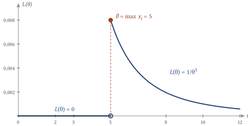
Şekil 10.6: U(0, \theta) modelinde 2, 3, 5 gözlemleri için olabilirlik. \theta < 5 iken 5 gözlemi imkânsızdır ve L(\theta) = 0 'dır; \theta \geq 5 iken L(\theta) = 1/\theta^3 azalır. En büyük değer, türevin sıfır olduğu bir noktada değil, sıçramanın olduğu \theta = 5 'te alınır.
