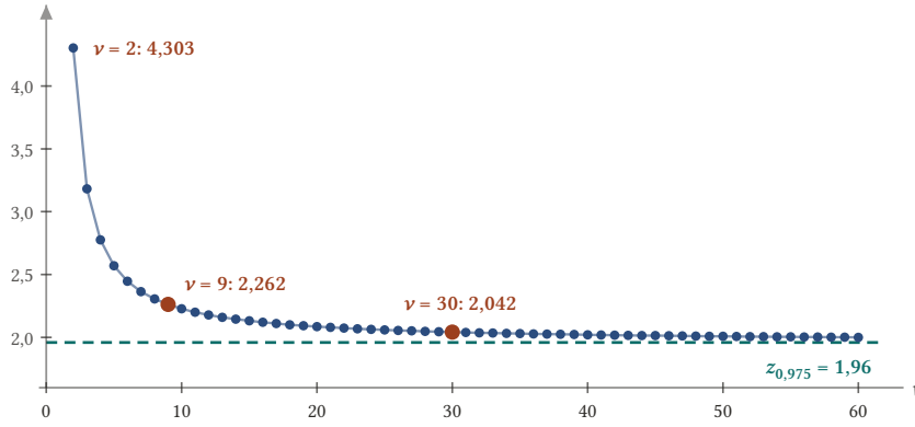
Şekil 13.5: Serbestlik derecesine göre t(\nu; 0,975) kantilleri. \nu küçükken kantil 1,96’dan belirgin biçimde büyüktür; \nu = 30 civarında fark 0,1’in altına iner ve \nu büyüdükçe kantiller z(0,975) = 1,96 ’ya yaklaşır.
