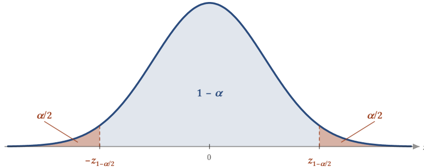
Şekil 13.2: Standart normal eğrisinin ortasında 1 - \alpha alan bırakan iki nokta: -z(1-\alpha/2) ve z(1-\alpha/2) . Her kuyrukta \alpha/2 alan kalır. Z = (\bar{X} - \mu)/(\sigma/\sqrt{n}) bu iki nokta arasına 1 - \alpha olasılıkla düşer.
