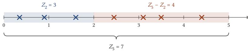
Şekil 3.2: (0, 2] aralığında 3, (2, 5] aralığında 4 olay: toplamda Z_5 = 7 . Ayrık iki aralıktaki sayılar bağımsızdır, ama Z_2 ile Z_5 ortak bir parçayı paylaştıkları için bağımsız değildir.
