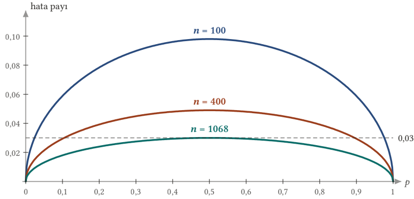
Şekil 15.3: %95 güven düzeyinde hata payı 1,96 \cdot \sqrt{p(1-p)/n} , p 'nin fonksiyonu olarak. Her n için en büyük değer p = 1/2 'de alınır; n = 1068 iken bu en büyük değer bile 0,03'ün altında kalır.
