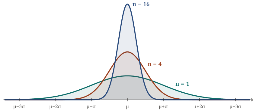
Şekil 7.4: N(\mu, \sigma^2) kitlesinden alınan örneklem ortalaması N(\mu, \sigma^2/n) dağılımlıdır. n = 1, 4 ve 16 için standart sapma \sigma, \sigma/2 ve \sigma/4 olur: eğri \mu 'de kalır ama n büyüdükçe daralır ve yükselir.
