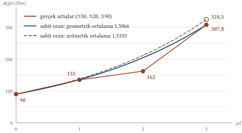
Şekil 6.2: 90 bin liralık eşyanın üç yıllık değeri. Gerçek yol (kırık çizgi) ile her yıl 1,5066 katına çıkan sabit artış aynı noktada, 307,8 bine biter. Oranların aritmetik ortalaması 1,5333 ise değeri 324,5 bine çıkararak olduğundan büyük gösterir.
