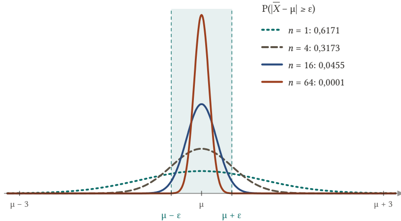
Şekil 11.8: \sigma = 1 olan normal bir kitleden \bar{X} 'in dağılımı n = 1, 4, 16, 64 için; taralı şerit \mu \pm \varepsilon , \varepsilon = 0,5 . n büyüdükçe dağılım \mu 'nün çevresine sıkışır ve şeridin dışına düşme olasılığı sifıra gider: \bar{X}, \mu 'nün tutarlı bir tahmin edicisidir.
