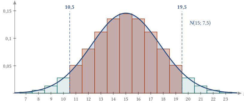
Şekil 5.10: \text{Binom}(30; 1/2) olasılıkları ve N(15; 7,5) eğrisi. 11'den 19'a kadar (uçlar dâhil) olan dikdörtgenler 10,5 ile 19,5 arasını kaplar; yaklaşık olasılık eğrinin bu aralıktaki alanıdır.
