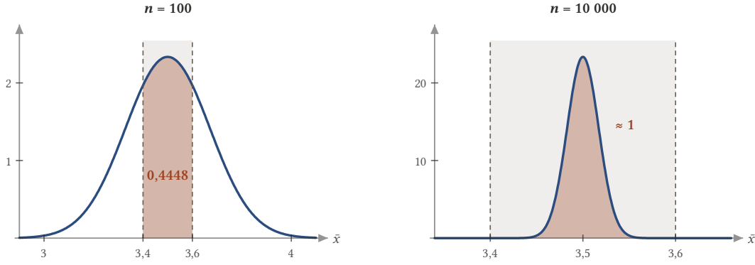
Şekil 8.6: Zar ortalamasının yaklaşık yoğunluğu N(3,5; (35/12)/n) ve 3,4 ile 3,6 arasındaki bant. n = 100 iken bandın içinde kalan alan 0,4448'dir. n = 10\,000 iken yoğunluk öylesine sivrilir ki (eksen ölçeği farklı) bütün alan bandın içine sığar: olasılık 0,99999995'tir.
