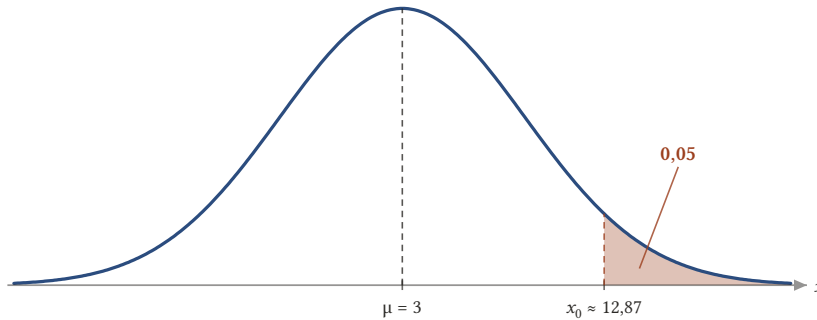
Şekil 5.7: X \sim N(3, 36) için sağ kuyruğun alanı 0,05 olacak biçimde seçilen nokta: x_0 = 3 + 6 \cdot 1,645 \approx 12,87 .
