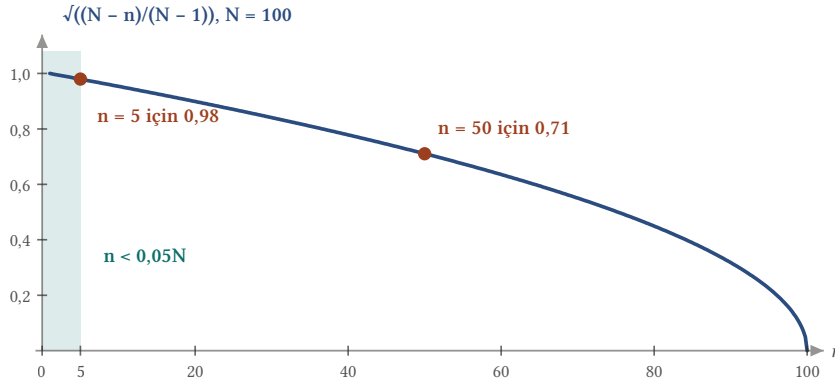
Şekil 7.1: N = 100 birimlik bir kitleden standart hatayı düzelten \sqrt{(N-n)/(N-1)} çarpanı. Örneklem kitlenin %5'inden küçükken (taralı şerit) çarpan 1'e çok yakındır; n büyüdükçe küçülür ve n = N olduğunda sıfır olur.
