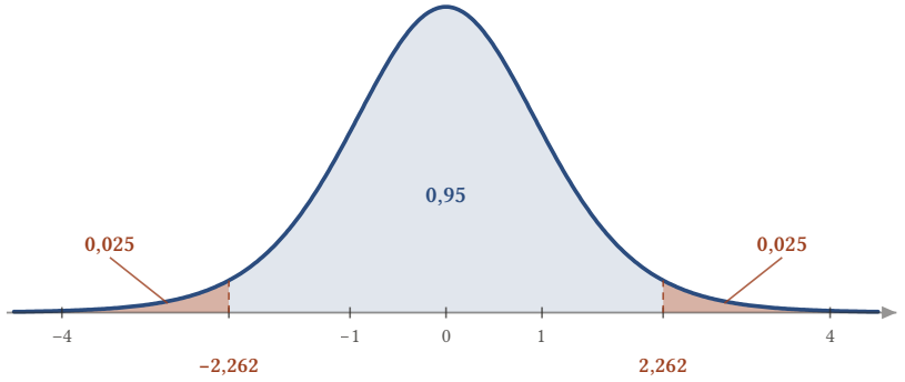
Şekil 12.4: t , yoğunluğu. Simetri nedeniyle 2,262'nin sağındaki ve -2,262'nin solundaki alanlar eşittir (0,025'er); aradaki alan 0,95'tir.
