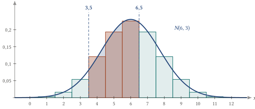
Şekil 5.9: Binom(12; 1/2) olasılıkları, her biri x - 1/2 ile x + 1/2 arasında duran genişliği 1 olan dikdörtgenler olarak çizildi; eğri N(6, 3) yoğunluğudur. 4, 5 ve 6'nın dikdörtgenleri (turuncu) 3,5 ile 6,5 arasını kaplar; bu yüzden normal yaklaşımda eğrinin altında 3,5 ile 6,5 arasında kalan alan (mavi) kullanılır.
