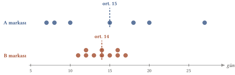
Şekil 15.4: İki lastik markasının dayanma süreleri. Ortalamalar (15 ve 14) birbirine yakın, fakat A markasının gözlemleri B markasınıninkilerden çok daha geniş bir alana yayılmış.
