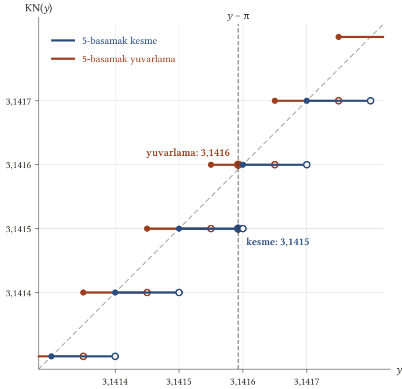
Şekil 2.4: \pi yakınındaki sayıların 5-basamak kesme (mavi) ve 5-basamak yuvarlama (turuncu) ile bulunan KN(y) değerleri. Basamakların sol ucu dahil, sağ ucu hariçtir; kesikli köşegen KN(y) = y doğrusudur. Kesme basamakları köşegenin hep altında kalır, yuvarlama basamakları köşegeni ortalar. y = \pi doğrusu kesmede 3,1415, yuvarlamada 3,1416 değerini verir.
