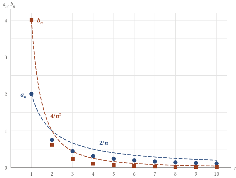
Şekil 3.4: a_n = (n+1)/n^2 (mavi daireler) ve b_n = (n+3)/n^3 (kırmızı kareler) dizilerinin ilk on terimi ile üst sınırları 2/n ve 4/n^2 (kesikli). n=1 'de iki dizi de sınırına eşittir; n \geq 3 için b_n sıfıra a_n 'den çok daha hızlı iner.
