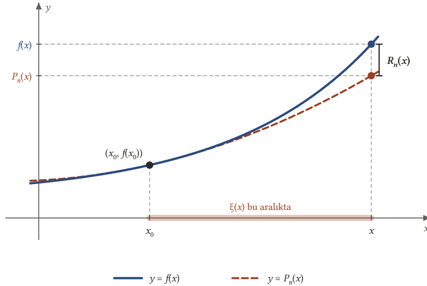
Şekil 1.6: Taylor teoremi: P_n , f 'nin grafiğine (x_0, f(x_0)) noktasında yapışır. Bir x noktasında iki grafik arasındaki dikey fark kesme hatası R_n(x) = f(x) - P_n(x) 'tir; formüldeki \xi(x) , x_0 ile x arasındaki (eksende kalın çizilen) aralıktadır.
