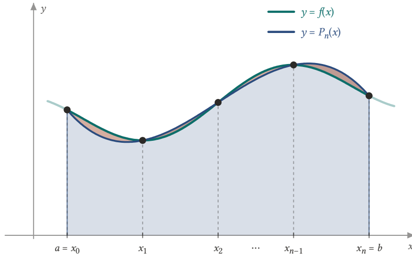
Şekil 11.5: Kapalı formülde [a, b] aralığını n eşit parçaya bölen n + 1 noktanın hepsi, uç noktalar dahil, düğümdür. f 'nin yerine bu noktalardan geçen y = P_n(x) polinomunun integrali alınır; taralı alan formülün değeridir.
