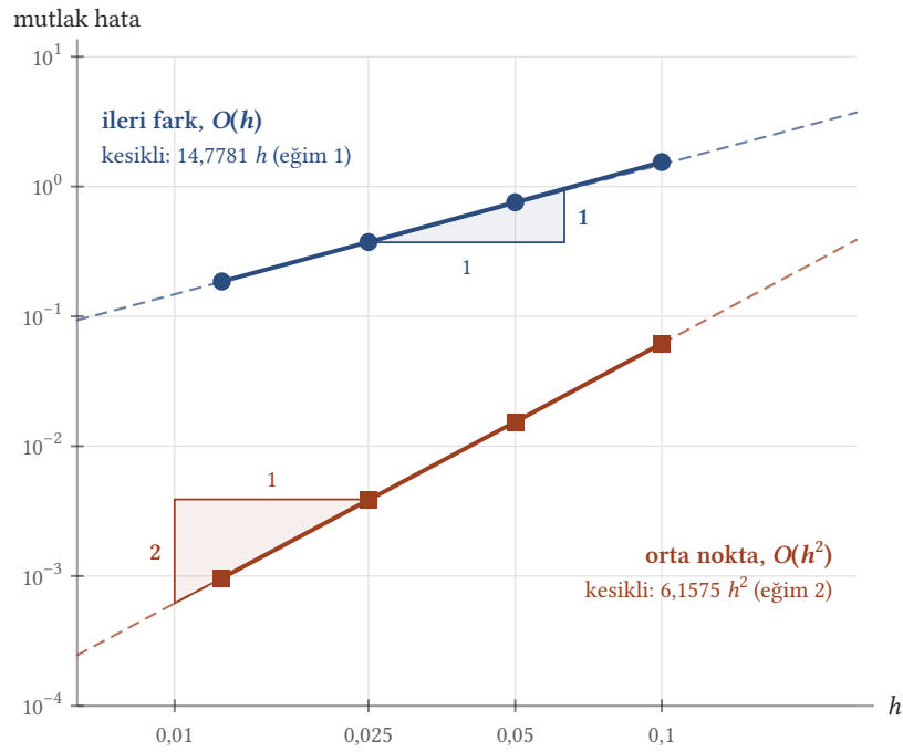
Şekil 10.4: f(x) = xe^x için f'(2) yaklaşımlarının mutlak hataları, log-log ölçeğe. Daireler ileri fark, kareler orta nokta formülüdür; h = 0,1; 0,05; 0,025; 0,0125 . Kesikli doğrular 14,7781 h ve 6,1575 h^2 referanslarıdır. İleri fark hataları eğimi 1, orta nokta hataları eğimi 2 olan doğru üzerinde dizilir.
