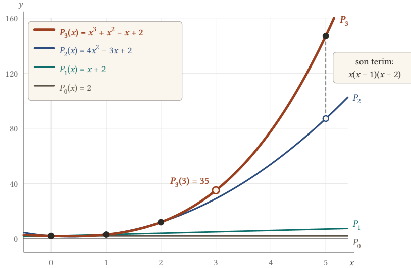
Şekil 9.2: Newton biçiminin kısmi toplamaları. P_0 yalnız (0; 2) noktasından, P_1 ilk iki noktadan, P_2 ilk üç noktadan geçer. P_2(5) = 87 olduğundan (5; 147) noktasına ancak son terim x(x - 1)(x - 2) eklenince ulaşılır. İçi boş daire P_3(3) = 35 değeridir.
