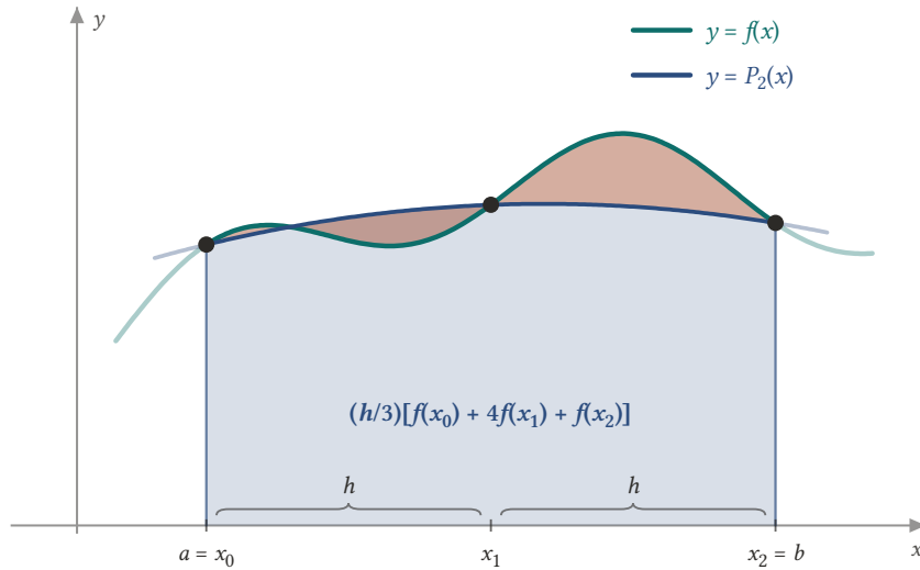
Şekil 11.3: Simpson Kuralı f 'yi üç düğümden geçen y = P_2(x) parabolüyle değiştirir. Taralı alan formülün ana kısmıdır; eğri ile parabol arasında kalan bölgeler hatayı gösterir.
