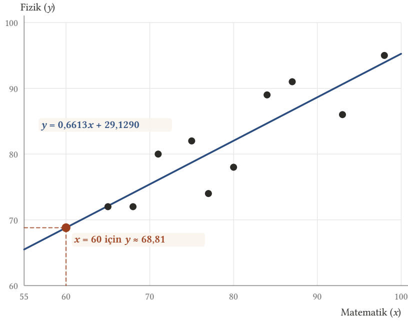
Şekil 12.4: On öğrencinin (Matematik, Fizik) notları ve regresyon doğrusu y = 0,6613x + 29,1290 . Matematik notu 60 olan öğrencinin Fizik notu tahmini doğru üzerindeki noktadan okunur: y \approx 68,81 , yani yaklaşık 69.
