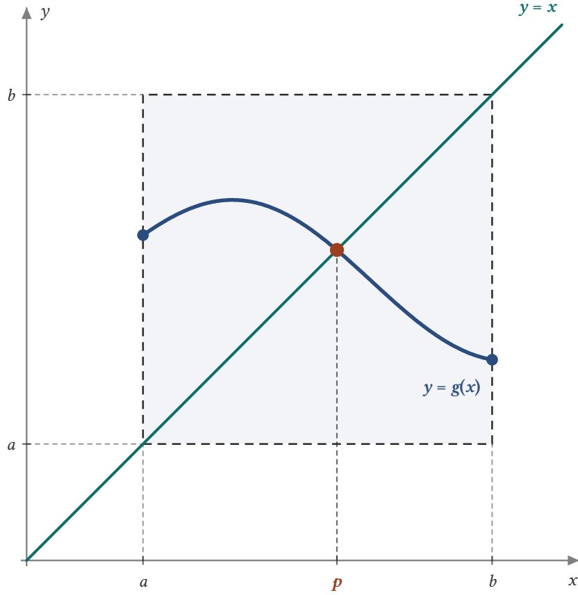
Şekil 5.2: g , [a, b] aralığını kendi içine gönderdiğinden grafiği kesikli karenin içinde kalır. Grafik karenin sol kenarında y = x doğrusunun üstünde, sağ kenarında altındadır; bu yüzden doğruyu bir (p, p) noktasında keser ve p bir sabit noktadır.
