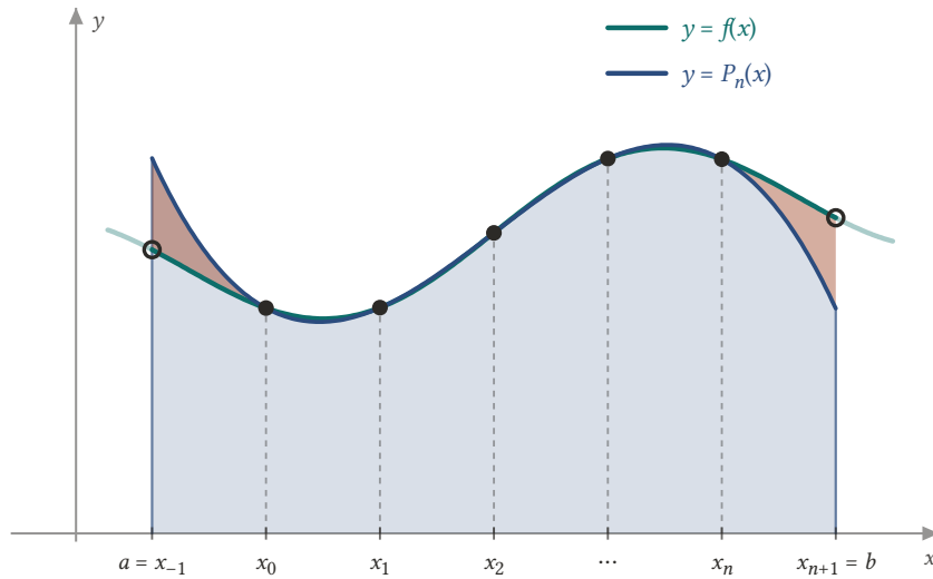
Şekil 11.7: Açık formülde [a, b] aralığı n + 2 eşit parçaya bölünür ve yalnız x_0, \dots, x_n iç noktaları düğümdür; f uç noktalarda hesaplanmaz (boş daireler). P_n yine de bütün [a, b] üzerinden integrelenir.
