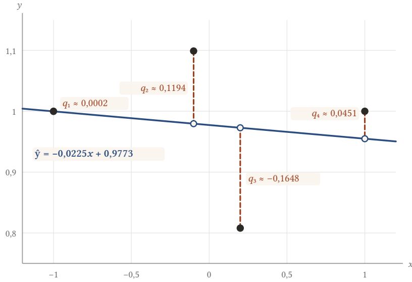
Şekil 12.2: Dört veri noktası (dolu daireler) ve regresyon doğrusu \hat{y} = -0,0225x + 0,9773 . Doğru üzerindeki içi boş daireler \hat{y}_i tahmini değerleridir. Kesikli parçalar q_i = y_i - \hat{y}_i artıklarıdır: her nokta ile doğru arasındaki dikey uzaklık. E, bu dört parçanın uzunluklarının karelerinin toplamıdır: E \approx 0,0435 .
