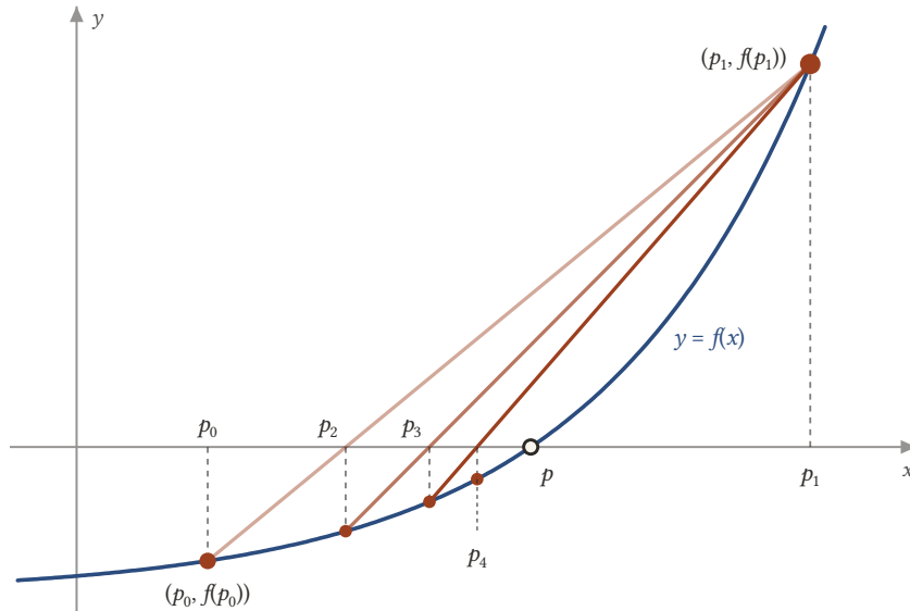
Şekil 7.3: Secant metodunun şeklindeki eğri ve başlangıç noktalarıyla Regula Falsi metodu. Yeni yaklaşımlarda f hep negatif kaldığından her kiriş, f 'nin pozitif olduğu (p_1, f(p_1)) ucuna bağlı kalır ve x eksenini p_2 , p_3 , p_4 'te keser. İlk iki kiriş Secant metodundakilerle aynıdır; ama p_4 kökün öbür yanına geçmez. Yaklaşımlar p 'ye hep soldan yaklaşır ve kök her adımda kirişin iki ucu arasında kalır.
