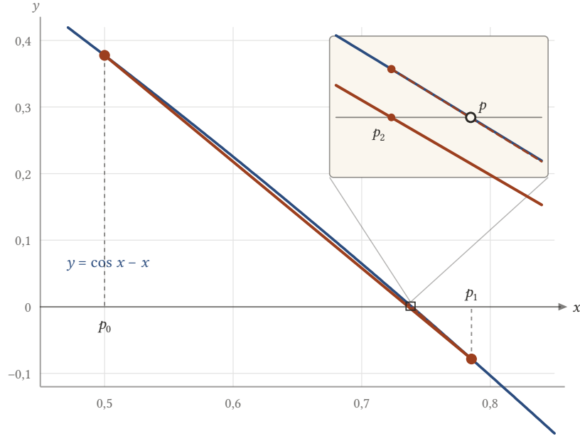
Şekil 7.2: y = \cos x - x eğrisi ve Secant metodunun ilk iki kirişi. (p_0, f(p_0)) ile (p_1, f(p_1)) noktalarından geçen kiriş x eksenini p_2 = 0,736384139 'da keser. Büyütülmüş pencerede kesikli çizilen ikinci kiriş eğriyle neredeyse çakışır ve eksen p_3 = 0,739058139 'da, p = 0,739085133 kökünün hemen yanında keser.
