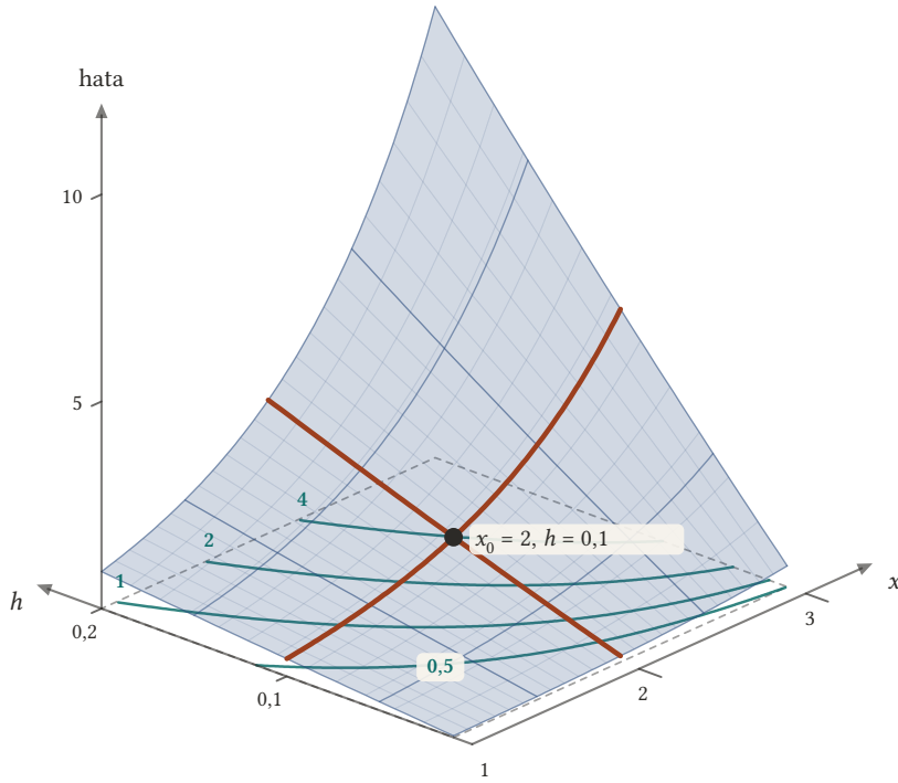
Şekil 10.5: İleri fark hatası E(x, h) = [f(x+h) - f(x)]/h - f'(x) , f(x) = x e^x , 1 \leq x \leq 3 , 0,01 \leq h \leq 0,2 . Yüzey h yönünde neredeyse doğrusal, x yönünde üstel büyür: en küçük değer yaklaşık 0,041 ( x = 1 , h = 0,01 ), en büyük değer yaklaşık 10,9 ( x = 3 , h = 0,2 ). Vurgulu eğriler h = 0,1 ve x = 2 kesitleridir; kesişimlerinde hata 1,5412779'dur. Tabandaki eğriler yaklaşık eşit hata eğrileridir (0,5; 1; 2; 4).
