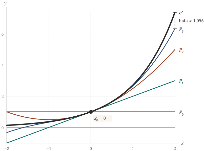
Şekil 8.3: e^x (kalın) ve x_0 = 0 civarındaki P_0, P_1, P_2, P_3 Taylor polinomları. Eğriler (0, 1) noktasında birbirine değeri ve 0 civarında üst üste biner, uçlara doğru açılarak ayrılır. x = 2 'de e^2 \approx 7,389 ile P_3(2) \approx 6,333 arasındaki fark yaklaşık 1,056'dır.
