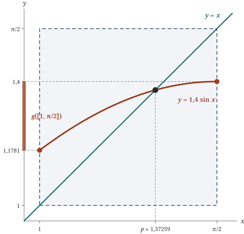
Şekil 5.4: g(x) = 1,4 \sin x fonksiyonu [1, \frac{\pi}{2}] aralığında artandır ve değerleri [1,1781; 1,4] aralığında kalır; bu aralık kesikli karenin içindedir. Eğri y = x doğrusunu karenin içinde tek bir p \approx 1,37259 noktasında keser.
