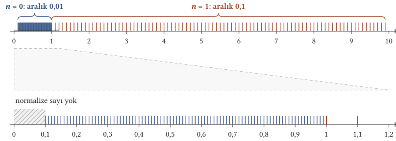
Şekil 2.3: İki basamaklı ( k = 2 ) pozitif normalize sayılar. Üstte [0, 10] aralığı: n = 0 için 0,10; 0,11; \dots; 0,99 sayıları [0,1; 1) içine sıkışır, n = 1 için 1,0; 1,1; \dots; 9,9 sayıları 0,1 aralıklarla dizilir. Altta [0; 1,2] parçasının büyütmesi: 0 ile 0,10 arasında normalize sayı yoktur.
