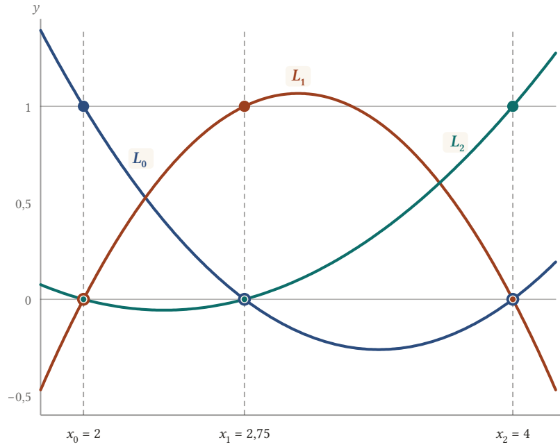
Şekil 8.5: x_0 = 2 , x_1 = 2,75 , x_2 = 4 düğümleri için L_0 , L_1 , L_2 Lagrange katsayı polinomları. Her L_k kendi düğümünde 1, öteki iki düğümde 0 değerini alır.
