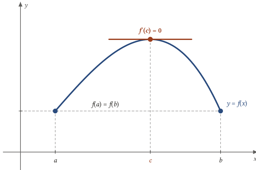
Şekil 1.1: Rolle teoremi: f(a) = f(b) olduğundan grafik iki uçta aynı yüksekliktedir. Arada bir c noktasında teğet yataydır, yani f'(c) = 0 olur.
