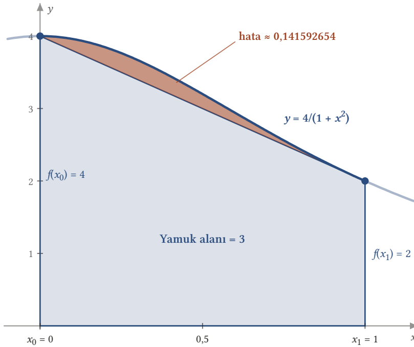
Şekil 11.2: f(x) = 4/(1+x^2) eğrisi ve Yamuk Kuralının kullandığı yamuk. Yamuğun alanı 3'tür. Eğri (0, 4) ile (1, 2) noktalarını birleştiren kirişin üstünde kaldığından yamuk integrali eksik ölçer; turuncu ince bölgenin alanı gerçek hata olan \pi - 3 \approx 0,141592654 'tür.
