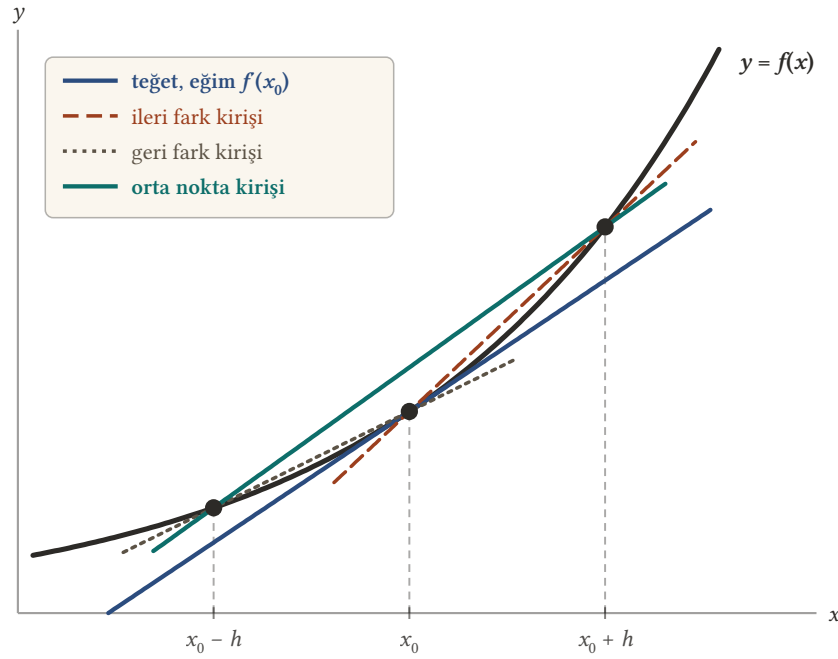
Şekil 10.2: x_0 noktasındaki teğet ve üç kiriş. İleri fark kirişi x_0 ile x_0 + h 'yi, geri fark kirişi x_0 - h ile x_0 'ı, orta nokta kirişi x_0 - h ile x_0 + h 'yi birleştirir. Tek yanlı kirişlerden biri teğetten dik, öteki yatık kalır; orta nokta kirişi ise teğete neredeyse paraleldir.
