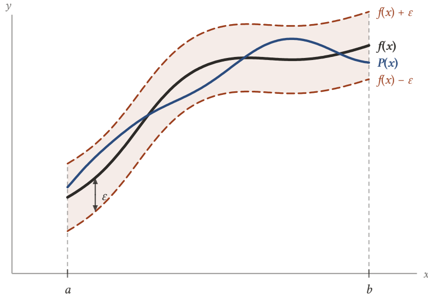
Şekil 8.1: f grafiğinin çevresinde, y = f(x) - \varepsilon ile y = f(x) + \varepsilon kesikli eğrileri arasındaki şerit. Teorem, [a, b] aralığının tamamında bu şeridin içinde kalan bir P polinomu bulunduğunu söyler.
