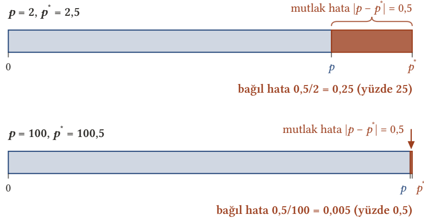
Şekil 2.1: Aynı mutlak hata, iki farklı büyüklükte. Mavi çubuk p , turuncu parça |p - p^*| = 0,5 mutlak hatasıdır; her satır kendi ölçeğinde çizilmiştir. p = 2 iken hata çubuğun dörtte biri kadardır (bağıl hata 0,25). p = 100 iken aynı hata ancak ince bir çizgidir (bağıl hata 0,005).
