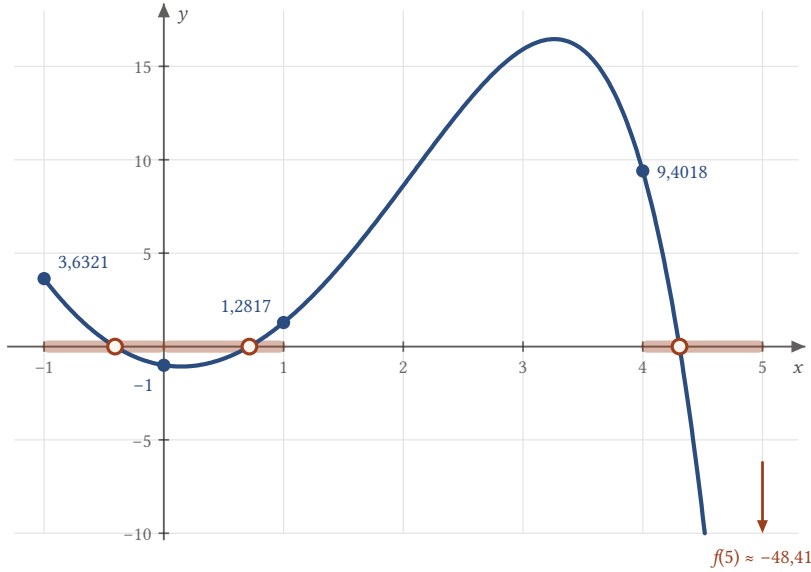
Şekil 1.5: y = 4x^2 - e^x grafiği. İşaretli noktalar f(-1) , f(0) , f(1) ve f(4) değerleridir. Eğri x ekseninin altına iner ve f(5) \approx -48,41 olur. Boş daireler x \approx -0,4078 ; 0,7148 ; 4,3066 köklerini, kalın parçalar bu kökleri içeren (-1, 0) , (0, 1) ve (4, 5) aralıklarını gösterir.
