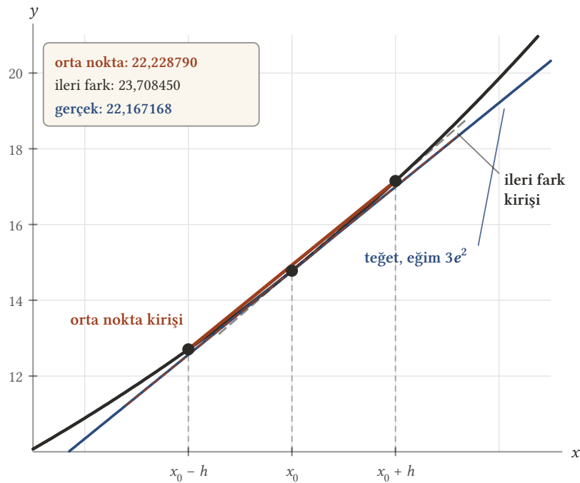
Şekil 10.3: f(x) = x e^x grafiği ve x_0 = 2 , h = 0,1 için tablo noktaları. Orta nokta kirişi (1,9; 12,703199) ile (2,1; 17,148957) noktalarını birleştirir; kesikli ince çizgi bu kirişin (2; 14,778112)'den geçen paralelidir ve teğetle neredeyse çakışır. Gri kesikli ileri fark kirişi belirgin biçimde daha diktir. Eğimler kutuda verilmiştir.
