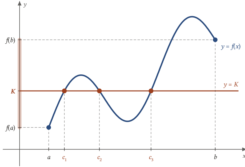
Şekil 1.4: Ara değer teoremi: K , f(a) ile f(b) arasında (eksendeki kalın parça) olduğundan y = K doğrusu grafiği en az bir noktada keser. Bu grafikte üç kesim noktası var; c_1, c_2, c_3 'ün her biri için f(c) = K olur.
