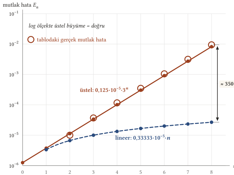
Şekil 3.3: Logaritmik ekseninde iki hata büyümesi. Kırmızı doğru üstel büyüme E_n = 0,125 \cdot 10^{-5} \cdot 3^n , içi boş daireler tablodaki beş-basamak hesabın gerçek mutlak hatalarıdır; kesikli mavi eğri lineer büyüme E_n = 0,33333 \cdot 10^{-5} \cdot n 'dir. n = 8 'de tablodaki hata lineer hatanın yaklaşık 350 katıdır.
