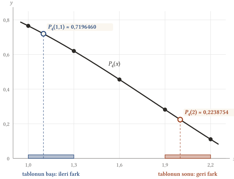
Şekil 9.4: (1,0; 0,7651977), \dots, (2,2; 0,1103623) beş noktasından geçen tek bir P_4 polinomu. x = 1,1 tablonun başında olduğundan ileri fark formülüyle, x = 2 tablonun sonunda olduğundan geri fark formülüyle hesaplanır; iki değer de aynı eğrinin üzerindedir.
