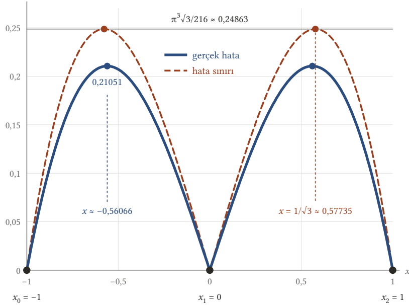
Şekil 8.6: Kalın eğri gerçek hata |\sin(\pi x/2) - x| , kesikli eğri teoremden gelen (\pi^3/48)|x^3 - x| sınırıdır. Sınırın tepeleri x = \pm 1/\sqrt{3} noktalarında \pi^3\sqrt{3}/216 \approx 0,24863 , gerçek hatanın tepeleri x \approx \pm 0,56066 noktalarında 0,21051'dir. Üç düğümde ikisi de sıfırdır ve sınır her yerde gerçek hatanın üstünde kalır.
