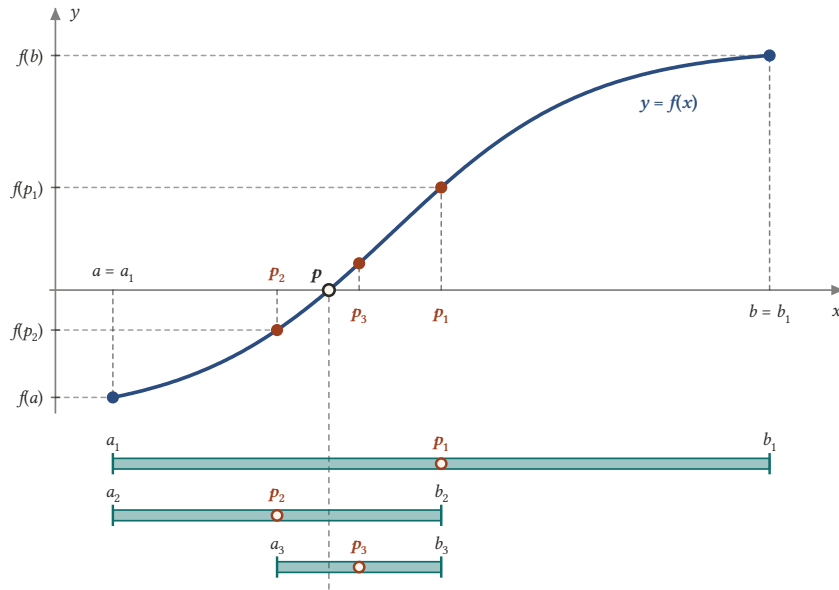
Şekil 4.1: İkiye bölme metodunun ilk üç adımı. f(p_1) > 0 olduğundan kök [a_1, p_1] yarısında, f(p_2) < 0 olduğundan [p_2, b_2] yarısındadır. Altta iç içe aralıkların her biri bir öncekinin yarısıdır ve p kökünü içerir.
