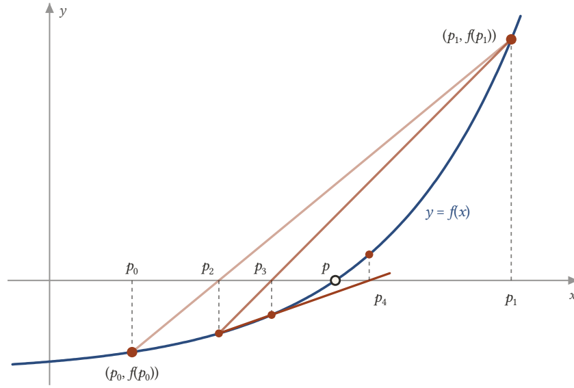
Şekil 7.1: Secant metodu. (p_0, f(p_0)) ile (p_1, f(p_1)) noktalarından geçen kiriş x eksenini p_2 'de keser. Sonraki her kiriş son iki noktadan geçer: (p_1, f(p_1)) ile (p_2, f(p_2)) kirişi p_3 'ü, (p_2, f(p_2)) ile (p_3, f(p_3)) kirişi p_4 'ü verir. p_4 , p kökünün öbür yanına düşer.
