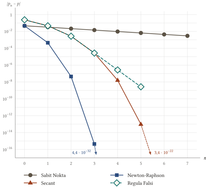
Şekil 7.5: \cos x - x = 0 denkleminde dört yöntemin |p_n - p| hataları, logaritmik dikey eksenle ( p = 0,7390851332 ). Sabit Nokta İterasyonunun hatası her adımda aynı oranda azalır ve noktalar bir doğru boyunca iner. Newton-Raphson ve Secant'ın eğrileri giderek dikleşir; aşağı oklar, eksenin altında kalan sonraki hataları gösterir. Secant ile Regula Falsi n = 3 'e kadar çıkışır, sonra Regula Falsi yavaşlar.
