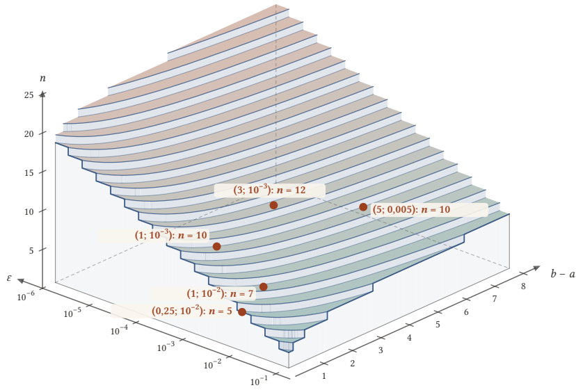
Şekil 4.4: n = \lceil \log_2((b-a)/\varepsilon) \rceil + 1 adım sayısı: b-a \in [0,25; 8] ve \varepsilon \in [10^{-6}, 10^{-1}] (logaritmik eksen) üzerinde tam sayı değerli teraslardan oluşan bir merdiven. Renk n büyüdükçe değişir. Etiketlerde (b-a; \varepsilon) çifti ve adım sayısı yazılıdır. (1; 10^{-3}) ile (5; 0,005) aynı terastadır, çünkü ikisinde de (b-a)/\varepsilon = 1000 'dir.
