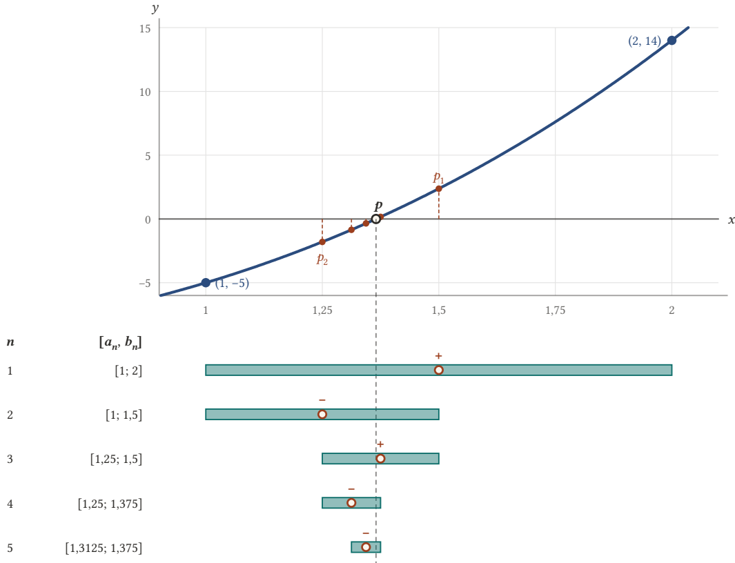
Şekil 4.3: Üstte f(x) = x^3 + 4x^2 - 10 grafiği; kesikli dikey parçalar p_1 = 1,5 , p_2 = 1,25 , p_3 = 1,375 , p_4 = 1,3125 , p_5 = 1,34375 orta noktalarındaki fonksiyon değerleridir. Altta aynı ölçekte ilk beş [a_n, b_n] aralığı, orta noktaları ve f(p_n) değerinin işareti. Her aralık bir öncekinin yarısıdır ve hepsi p \approx 1,3652 kökünü (kesikli çizgi) içerir.
