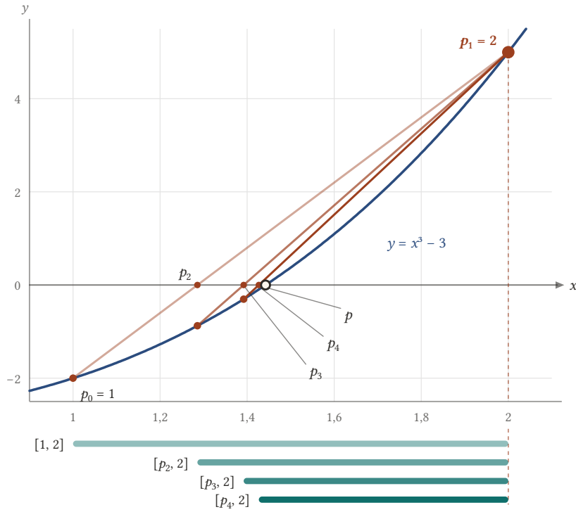
Şekil 7.4: y = x^3 - 3 için Regula Falsi metodunun ilk üç kirişi. Bütün kirişler sağ uçtaki (2, 5) noktasından çıkar ve x eksenini sırasıyla p_2 = 1,285714286 , p_3 = 1,392059553 , p_4 = 1,426733629 'da keser; kök p = 1,442249570 'tir. Altta çubuklar kökü içeren aralıklardır: sol uç köke yaklaşırken sağ uç hep 2'de kalır.
