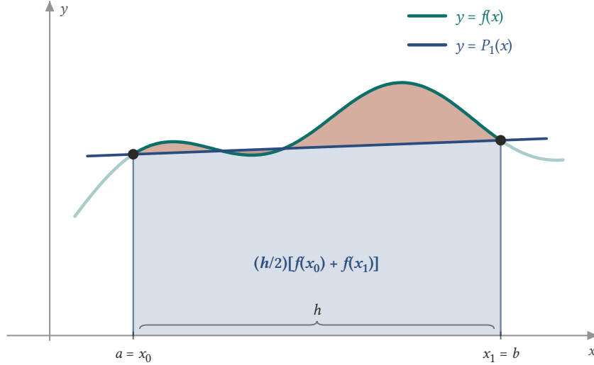
Şekil 11.1: Yamuk Kuralı f' 'yi uç noktalardan geçen y = P_1(x) doğrusuyla değiştirir. Taralı yamuğun alanı formülün ana kısmıdır; eğri ile doğru arasında kalan bölgeler hatayı gösterir.
