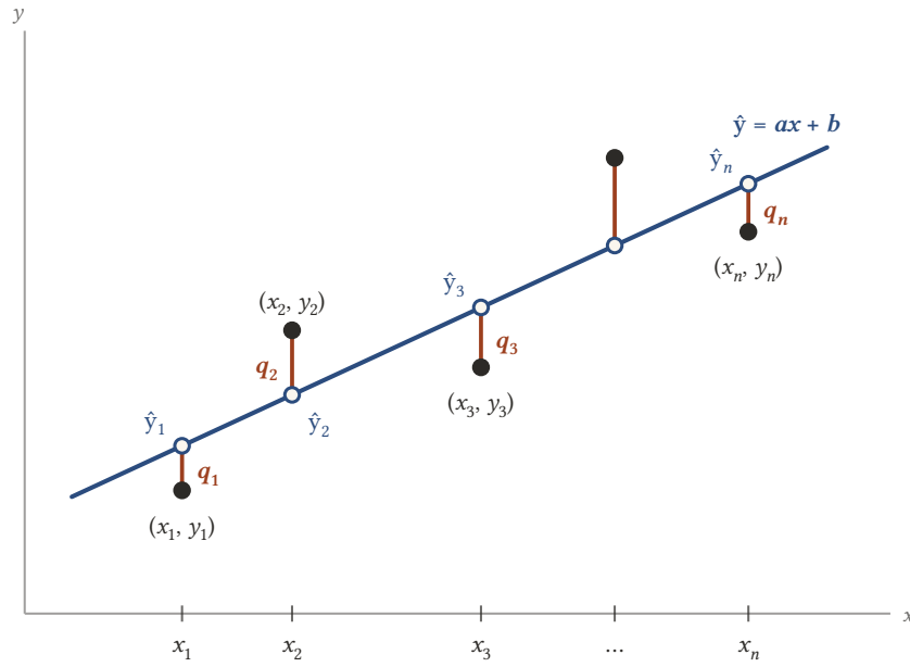
Şekil 12.1: Veri noktaları (x_i, y_i) (dolu daireler), \hat{y} = ax + b doğrusu ve doğru üzerindeki \hat{y}_i = ax_i + b tahmini değerleri (içi boş daireler). Dikey parçalar q_i = y_i - \hat{y}_i farklarıdır; en küçük kareler yöntemi bu parçaların uzunluklarının karelerinin toplamı E 'yi en küçük yapan doğruyu seçer.
