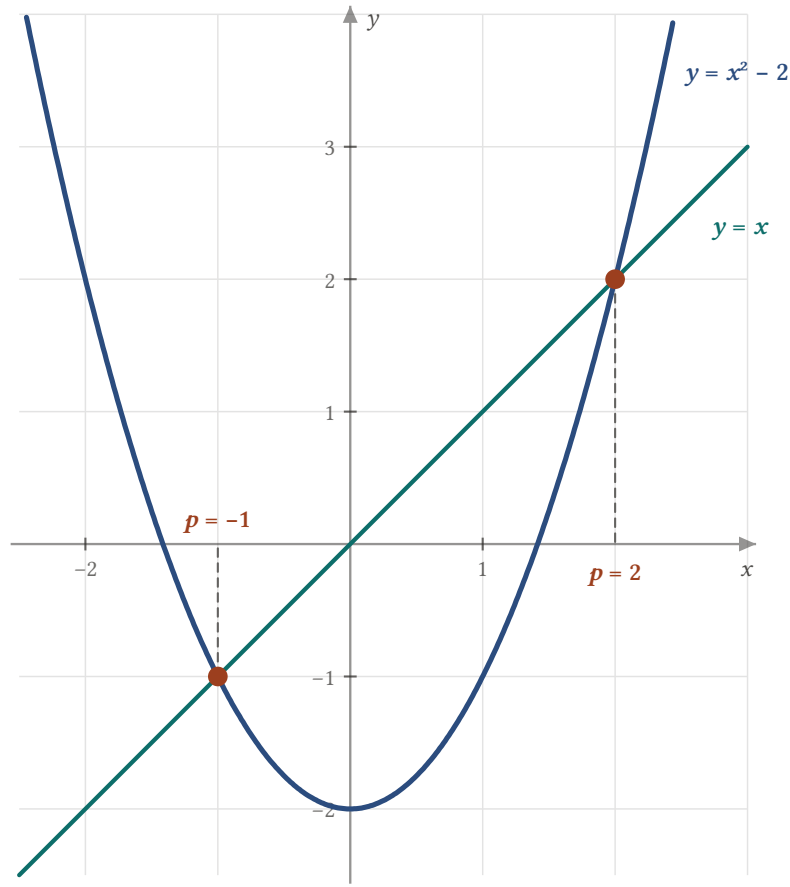
Şekil 5.1: y = x^2 - 2 parabolü y = x doğrusunu (-1, -1) ve (2, 2) noktalarında keser. Bu noktaların apsisleri g(x) = x^2 - 2 fonksiyonunun sabit noktalarıdır.
