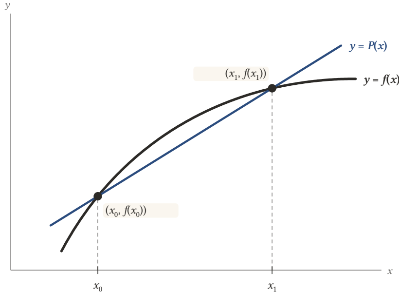
Şekil 8.4: y = f(x) eğrisi ve (x_0, f(x_0)) , (x_1, f(x_1)) noktalarından geçen y = P(x) doğrusu. P , iki düğümde f ile aynı değeri alır; düğümlerin arasında ve dışında f 'den ayrılır.
