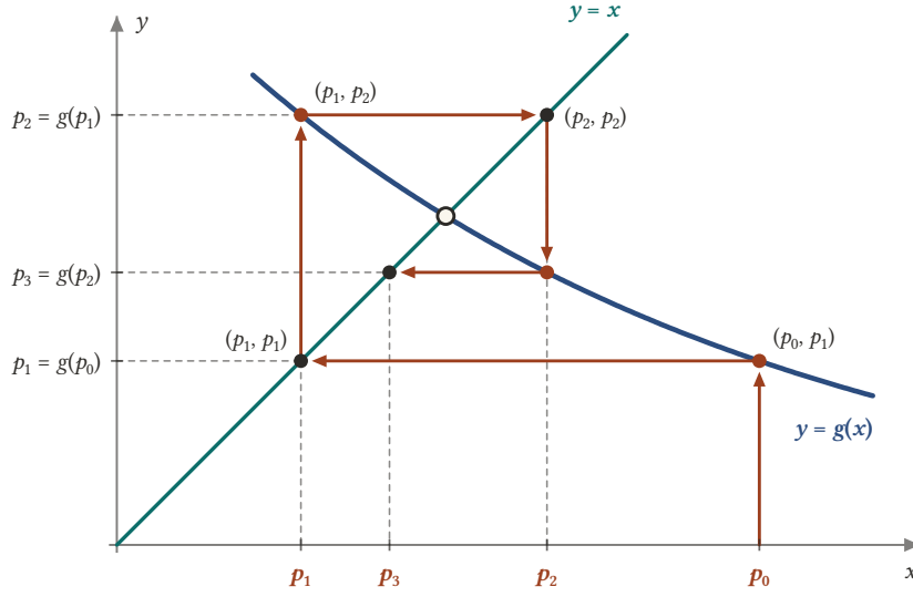
Şekil 5.3: Sabit nokta iterasyonunun geometrik yorumu. p_0 'dan dikey olarak y = g(x) grafiğine çıkılır ve p_1 = g(p_0) okunur. Yatay olarak y = x doğrusuna gidilince p_1 yatay eksenine taşınır ve adım tekrarlanır. Azalan g için terimler sabit noktanın (içi boş nokta) iki yanında dolanarak ona yaklaşır.
