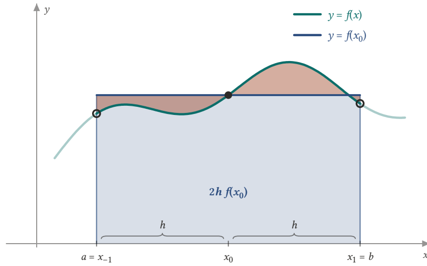
Şekil 11.8: Orta Nokta Kuralı f' 'yi orta noktadaki değerine eşit sabitle değiştirir: taralı dikdörtgenin tabanı 2h , yüksekliği f(x_0) 'dır. Eğri ile dikdörtgenin üst kenarı arasında kalan bölgeler hatayı gösterir.
