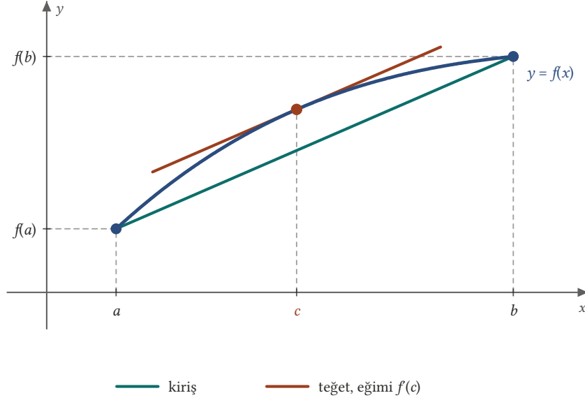
Şekil 1.2: Ortalama değer teoremi: (a, f(a)) ile (b, f(b)) noktalarını birleştiren kirişin eğimi (f(b) - f(a))/(b - a) 'dır. Arada bir c noktasındaki teğet bu kirişe paraleldir.
