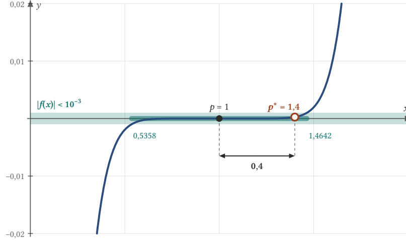
Şekil 4.2: f(x) = (x - 1)^9 grafiği. Taralı şerit |f(x)| < 10^{-3} bölgesidir. Grafik bu şeridin içinde (0,5358; 1,4642) aralığı boyunca kalır, kalın parça bu aralıktır. p^* = 1,4 noktasında f(1,4) \approx 0,000262 olduğundan nokta eksenin hemen üstündedir, ama kökten uzaklığı 0,4 'tür.
