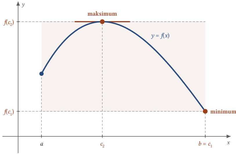
Şekil 1.3: Ekstrem değer teoremi: [a, b] üzerinde sürekli f bütün değerlerini f(c_1) ile f(c_2) arasında (taralı bant) alır. Maksimum bir iç noktada alınmıştır ve orada teğet yataydır ( f'(c_2) = 0 ); minimum ise b uç noktasında alınmıştır.
