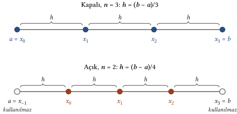
Şekil 11.6: Kapalı formülde ( n = 3 ) [a, b] üç eşit parçaya bölünür ve uç noktalar dahil dört nokta düğümdür. Açık formülde ( n = 2 ) aralık dört eşit parçaya bölünür; uç noktalar x_{-1} = a ve x_3 = b kullanılmaz, düğümler yalnız üç iç noktadır.
