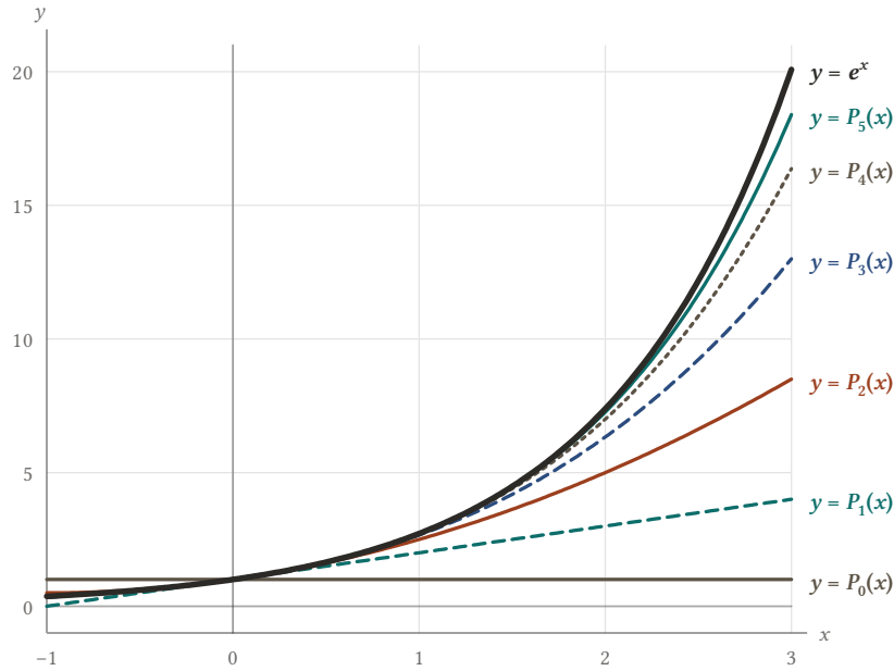
Şekil 8.2: e^x (kalın) ve x_0 = 0 civarındaki P_0, P_1, \dots, P_5 Taylor polinomları, [-1, 3] aralığında. 0 civarında bütün eğriler e^x ile neredeyse çakışır; x = 3 'te ise P_5(3) = 18,4 bile e^3 \approx 20,086 değerinden belirgin biçimde uzaktır.
