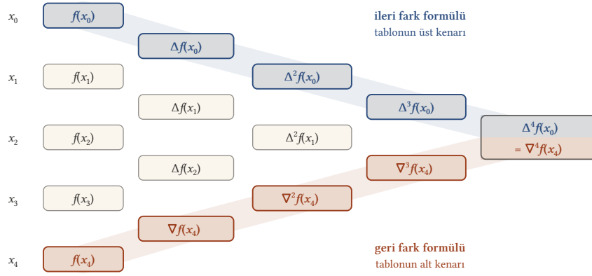
Şekil 9.3: Beş eşit aralıklı nokta için tek bir fark tablosu. İleri fark formülü üst kenardaki f(x_0), \Delta f(x_0), \dots, \Delta^4 f(x_0) sayılarını; geri fark formülü alt kenardaki f(x_4), \nabla f(x_4), \dots, \nabla^4 f(x_4) sayılarını kullanır. Alt kenardaki her girdi bir ileri farktır, örneğin \nabla^2 f(x_4) = \Delta^2 f(x_2) ; son sütundaki tek girdi iki kenarda ortaktır.
