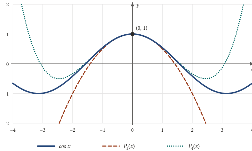
Şekil 1.7: y = \cos x ile x_0 = 0 civarındaki Taylor polinomları P_2(x) = 1 - x^2/2 ve P_4(x) = 1 - x^2/2 + x^4/24 . Üç eğri (0, 1) noktası civarında üst üste biner. Uzaklaştıkça önce P_2 , daha geç P_4 kosinüsten ayrılır: x = 2 'de \cos 2 \approx -0,4161 , P_2(2) = -1 , P_4(2) \approx -0,3333 olur.
