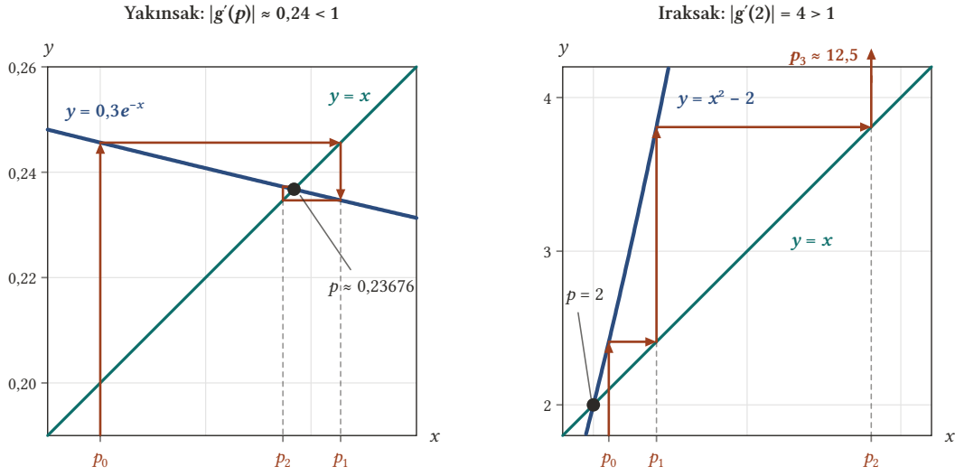
Şekil 5.5: Örümcek ağı diyagramları. Solda g(x) = 0,3e^{-x} ve p_0 = 0,2 : eğriye dikey, y = x doğrusuna yatay adımlar kökün iki yanında dolanarak p \approx 0,23676 noktasına daralır. Sağda g(x) = x^2 - 2 ve p_0 = 2,1 : adımlar 2,41 ve 3,8081 üzerinden p = 2 kökünden uzaklaşır, p_3 \approx 12,5 çerçevenin dışındadır.
