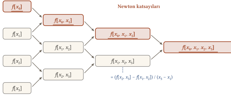
Şekil 9.1: Dört noktalı bölünmüş fark tablosunun hesap şeması. Her kutu, solundaki üst ve alt komşusundan hesaplanır: alttaki eksi üstteki, bölü kapsanan ilk ve son noktanın farkı. Örneğin f[x_1, x_2, x_3] = (f[x_2, x_3] - f[x_1, x_2]) / (x_3 - x_1) . Üst kenardaki altı çizili kutular Newton katsayılarıdır.
