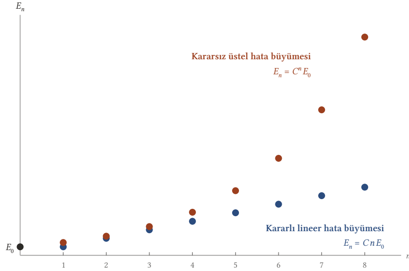
Şekil 3.1: İlk hata E_0 olmak üzere n = 1, 2, \dots, 8 adım sonraki hatalar. Mavi noktalar lineer büyüme E_n = CnE_0 ( C = 1 ), kırmızı noktalar üstel büyüme E_n = C^n E_0 ( C = 1,5 ) içindir. İlk adımlarda iki hata birbirine yakındır; n = 8 'de lineer hata 8E_0 , üstel hata yaklaşık 25,6E_0 olur.
