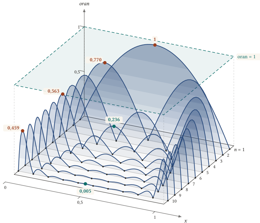
Şekil 8.7: [0, 1] aralığında h = 1/n adımlı n + 1 eşit aralıklı düğüm için |(x - x_0) \cdots (x - x_n)| çarpımının h^{n+1} n! / 4 sınırına oranı, n = 1, 2, \dots, 10 . Her şerit bir n değerine aittir; dolgu, oran büyüdükçe koyulaşır. Bütün şeritler oran = 1 düzleminin altında kalır. Uç alt aralıklardaki tepeler ( n = 1, 2, 5, 10 için 1; 0,770; 0,563; 0,459) yüksektir; orta alt aralıktaki tepe n = 4 'te 0,236, n = 10 'da 0,005'tir.
