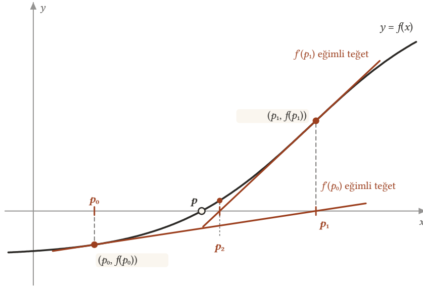
Şekil 6.1: Newton-Raphson Metodunun geometrik anlamı. (p_0, f(p_0)) noktasındaki teğet x eksenini p_1 'de, (p_1, f(p_1)) noktasındaki teğet p_2 'de keser; p_2 , p köküne p_0 'dan çok daha yakındır.
