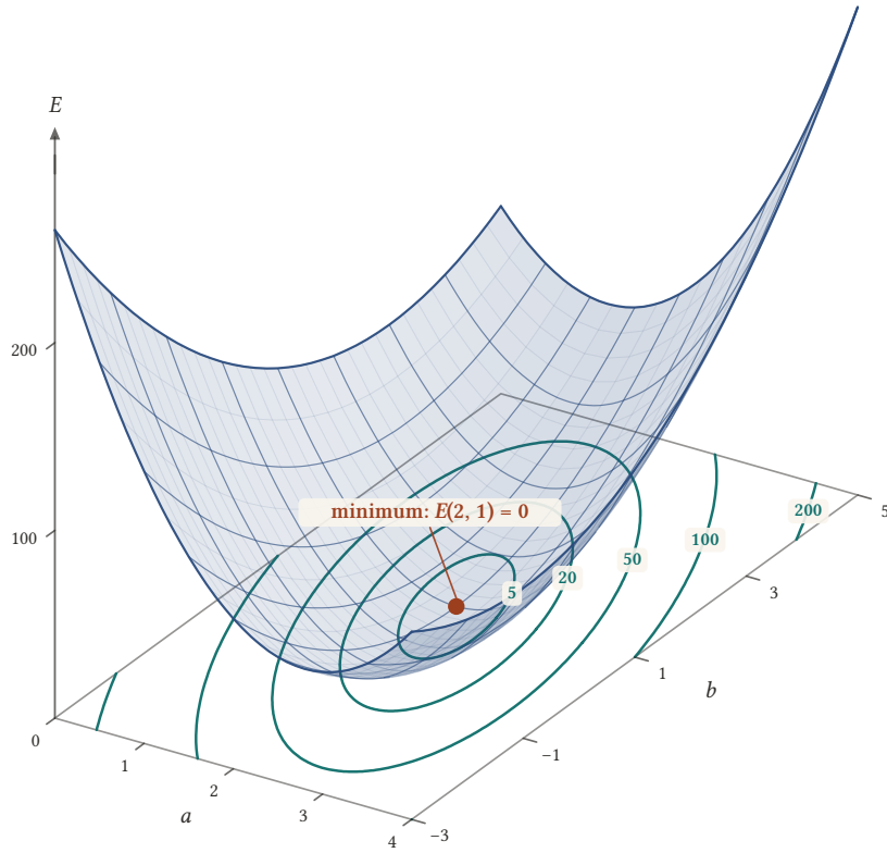
Şekil 12.3: E(a, b) = 25a^2 + 10ab + 5b^2 - 110a - 30b + 125 yüzeyinin 0 \leq a \leq 4 , -3 \leq b \leq 5 üzerindeki parçası. Köşelerde E 100 ile 260 arasındadır. Tabandaki eğik elipsler E = 5; 20; 50; 100; 200 seviye eğrileridir ve hepsi (2, 1) noktasını çevreler. Yüzeyin tek bir çukuru vardır; normal denklemlerin çözümü olan (2, 1) bu çukurun dibidir ve orada E = 0 olur. Yüzeyin arkasında kalan çizgiler soluk çizilmiştir.
