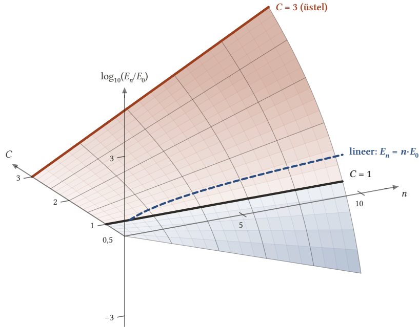
Şekil 3.2: z = \log_{10}(E_n/E_0) = n \log_{10} C yüzeyi ( 0 \leq n \leq 10 , 0,5 \leq C \leq 3 ). Mavi bölgede ( C < 1 ) hata söner, kırmızı bölgede ( C > 1 ) üstel olarak büyür; C = 1 kesitinde yüzey düzdür. Kırmızı kalın eğri C = 3 kesitidir, kesikli mavi eğri ise lineer büyüme E_n = nE_0 için \log_{10} n değeridir. Yüzeyin arkasında kalan çizgiler soluk çizilmiştir.
