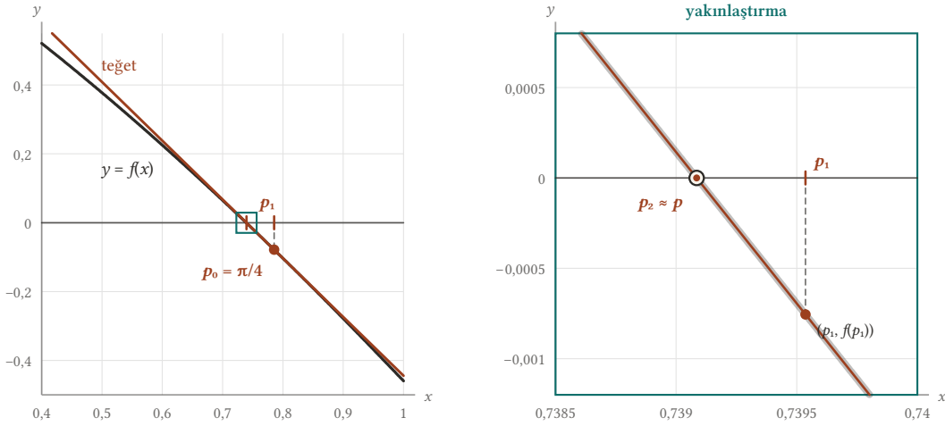
Şekil 6.3: f(x) = \cos x - x için Newton-Raphson adımları. Solda p_0 = \pi/4 noktasındaki teğet x eksenini p_1 = 0,739536 'da keser; teğet grafiğe o kadar yakındır ki ancak uçlarda ayrılır. Küçük kare, sağda büyütülen [0,7385; 0,7400] \times [-0,0012; 0,0008] penceresinin yerini gösterir (gerçek boyutu bu ölçekte bir pikselden küçüktür). Sağda grafik ile p_1 'deki teğet ayırt edilemez; teğet x eksenini p_2 = 0,739085178 'de keser ve içi boş daireyle gösterilen p = 0,739085133 kökü bu ölçekte p_2 ile üst üstedir.
